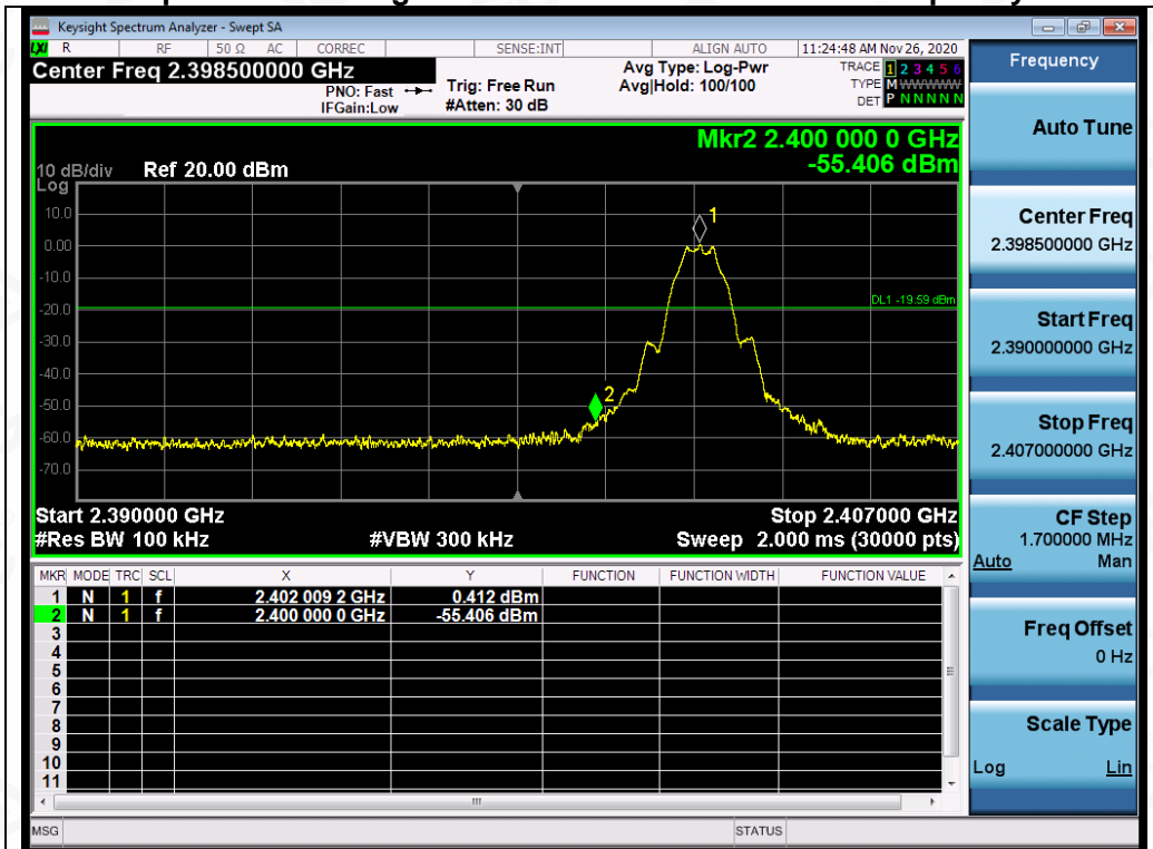
Test_Graph_LE1M_2402_1Mbps_Lower Band Edge Emissions
