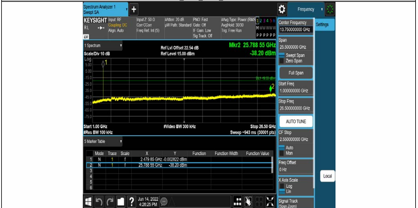
DH5_Ant1_2480_1000~26500
