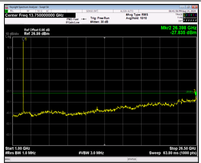
Band41-20MHz-QPSK-40620-1RB#0-Range2:1000~26500MHz
