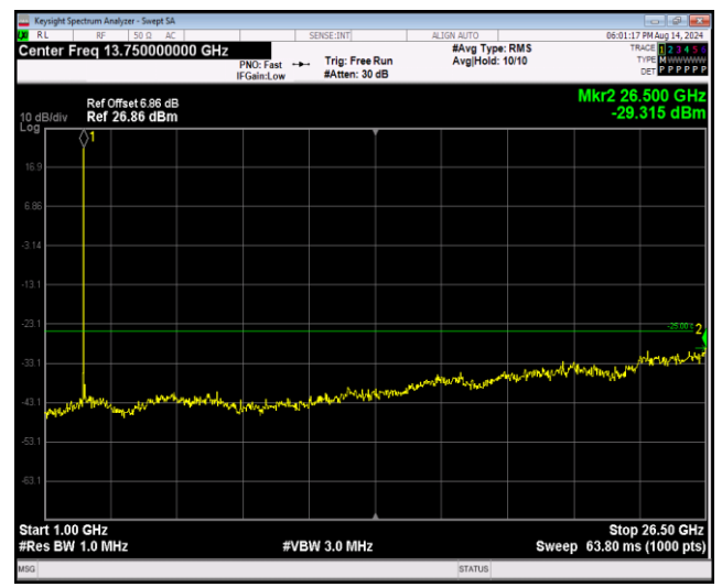
Band41-5MHz-QPSK-40620-1RB#0-Range2:1000~26500MHz
