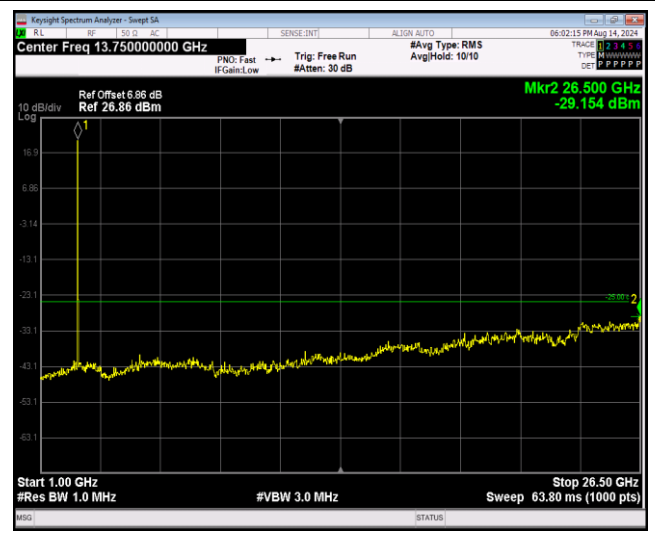
Band41-5MHz-QPSK-40620-1RB#0-Range2:1000~26500MHz
