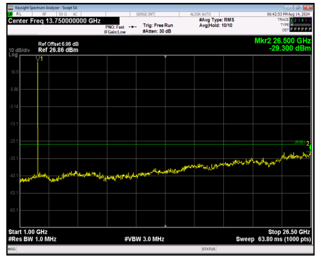
Band41-20MHz-QPSK-41490-1RB#0-Range2:1000~26500MHz
