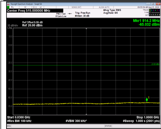
66-66-20MHz-5MHz-QPSK-QPSK-132397-132514-1RB# 0-1RB#24-30~1000MHz-PASS
