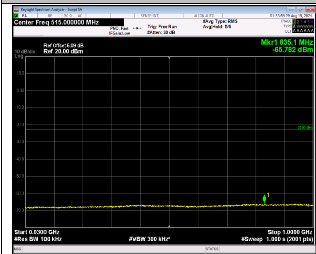
66-66-20MHz-5MHz-64QAM-64QAM-132072-132189-10 ORB#0-25RB#0-30~1000MHz-PASS
