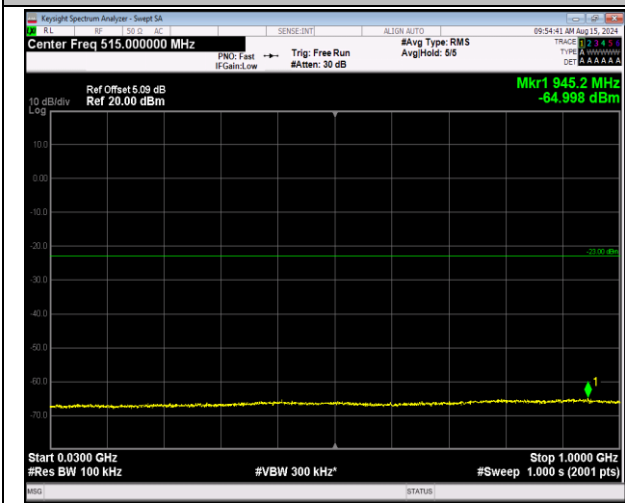
66-66-20MHz-5MHz-QPSK-QPSK-132397-132514-1RB# 99-0RB#0-30~1000MHz-PASS
