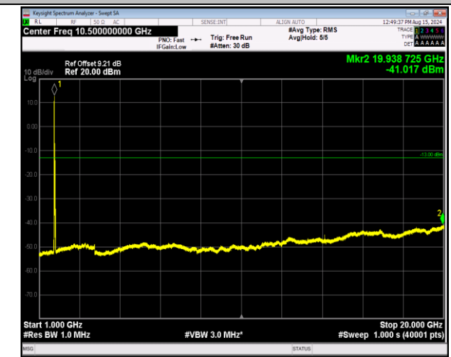
66-66-20MHz-20MHz-16QAM-16QAM-132072-132270-1RB #0-1RB#99-1000~20000MHz-PASS
