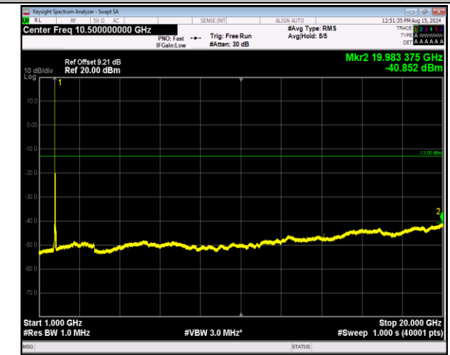
66-66-20MHz-20MHz-QPSK-QPSK-132323-132521-1RB#0 -0RB#0-1000~20000MHz-PASS
