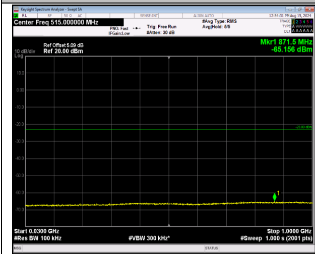
66-66-20MHz-20MHz-16QAM-16QAM-132323-132521-1 RB#0-1RB#99-30~1000MHz-PASS
