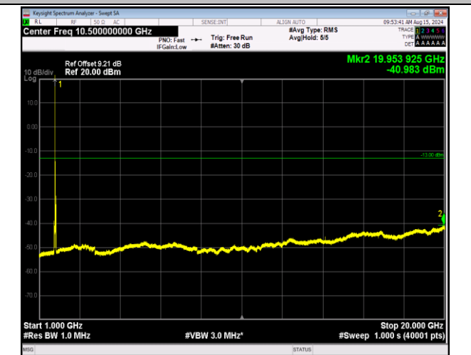
66-66-20MHz-5MHz-QPSK-QPSK-132397-132514-1RB#0- ORB#0-1000~20000MHz-PASS
