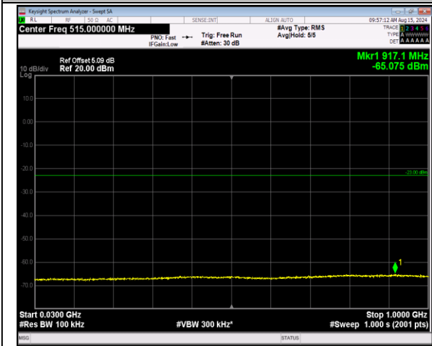
66-66-20MHz-5MHz-QPSK-QPSK-132397-132514-100R B#0-25RB#0-30~1000MHz-PASS
