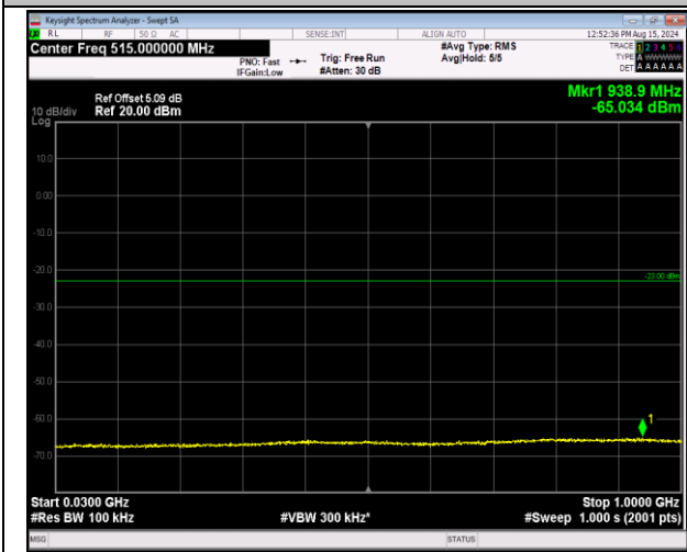
66-66-20MHz-20MHz-QPSK-QPSK-132323-132521-1RB #99-0RB#0-30~1000MHz-PASS
