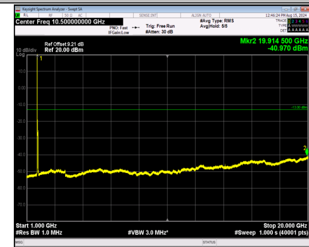
66-66-20MHz-20MHz-QPSK-QPSK-132072-132270-1RB#0 -ORB#0-1000~20000MHz-PASS
