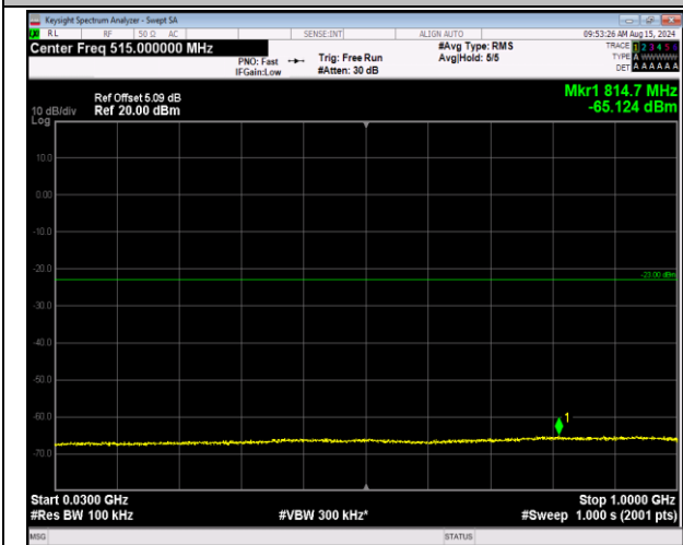
66-66-20MHz-5MHz-QPSK-QPSK-132397-132514-1RB# 0-ORB#0-30~1000MHz-PASS
