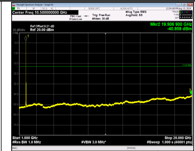
66-66-20MHz-20MHz-QPSK-QPSK-132323-132521-1RB#0 -1RB#99-1000~20000MHz-PASS
