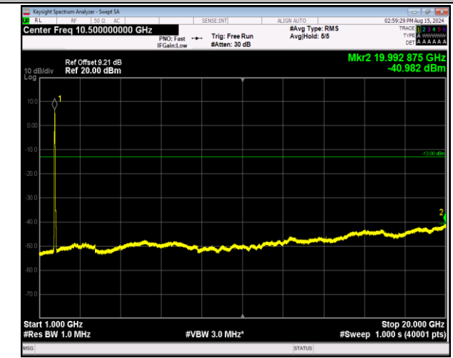
66-66-20MHz-20MHz-64QAM-64QAM-132072-132270-100 RB#0-100RB#0-1000~20000MHz-PASS
