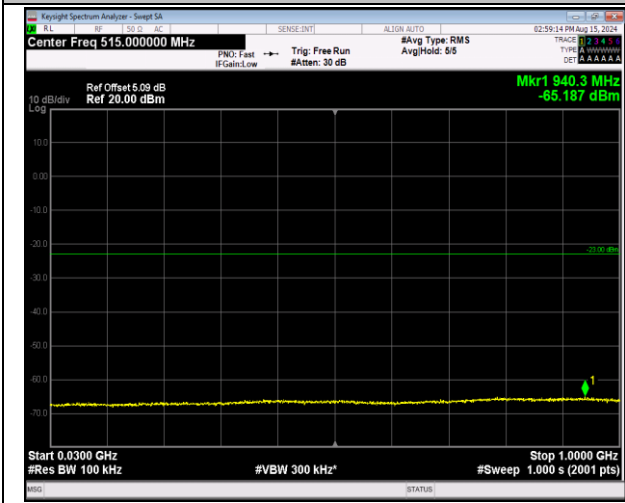
66-66-20MHz-20MHz-64QAM-64QAM-132072-132270-1 00RB#0-100RB#0-30~1000MHz-PASS
