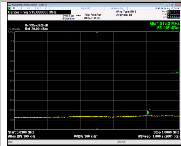
66-66-20MHz-20MHz-QPSK-QPSK-132072-132270-1RB #99-0RB#0-30~1000MHz-PASS
