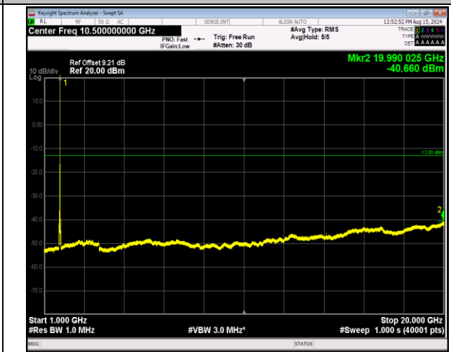
66-66-20MHz-20MHz-QPSK-QPSK-132323-132521-1RB#9 9-0RB#0-1000~20000MHz-PASS
