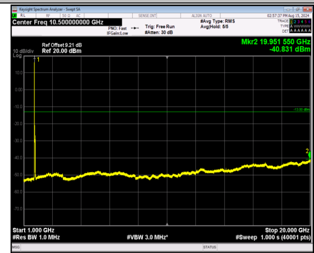
66-66-20MHz-20MHz-64QAM-64QAM-132072-132270-1RB#0-0RB#0-1000~20000MHz-PASS
