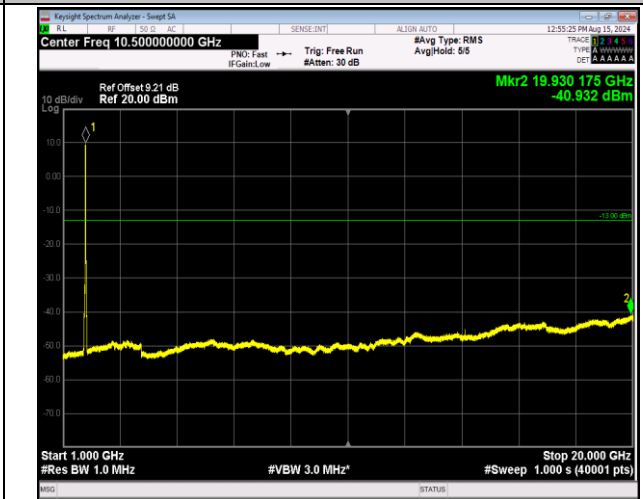
66-66-20MHz-20MHz-QPSK-QPSK-132323-132521-100RB #0-100RB#0-1000~20000MHz-PASS
