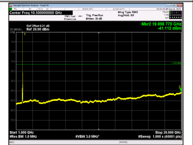
66-66-5MHz-20MHz-QPSK-QPSK-132455-132572-1RB#0- ORB#0-1000~20000MHz-PASS
