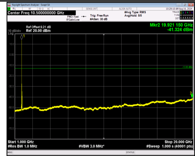
66-66-5MHz-20MHz-QPSK-QPSK-132330-132447-1RB#0- 1RB#99-1000~20000MHz-PASS
