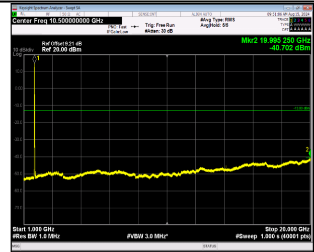
66-66-20MHz-5MHz-QPSK-QPSK-132072-132189-1RB#0- 1RB#24-1000~20000MHz-PASS
