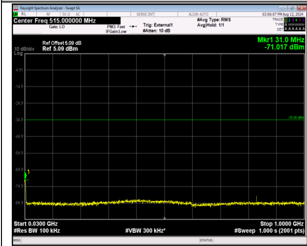
41-41-20MHz-10MHz-QPSK-QPSK-40571-40715-100RB #0-50RB#0-30~1000MHz-PASS
