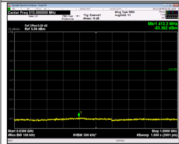
41-41-20MHz-10MHz-64QAM-64QAM-39750-39894-100 RB#0-50RB#0-30~1000MHz-PASS
