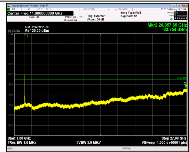
41-41-20MHz-10MHz-QPSK-QPSK-40571-40715-1RB#99- ORB#0-1000~27000MHz-PASS
