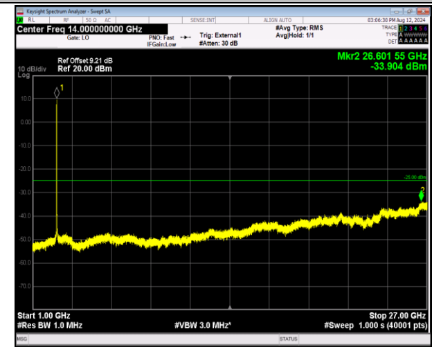
41-41-20MHz-10MHz-QPSK-QPSK-40571-40715-100RB#0 -50RB#0-1000~27000MHz-PASS
