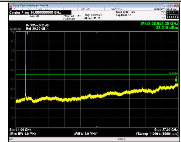
41-41-20MHz-10MHz-QPSK-QPSK-40571-40715-1RB#0-0 RB#0-1000~27000MHz-PASS
