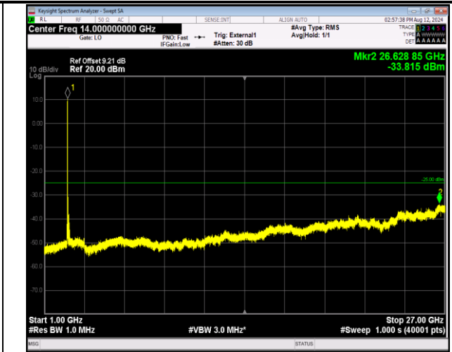
41-41-20MHz-10MHz-QPSK-QPSK-39750-39894-1RB#0-1 RB#49-1000~27000MHz-PASS
