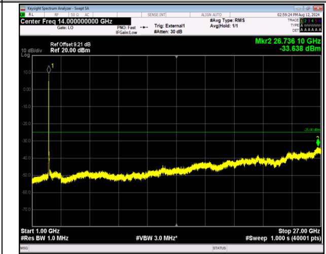
41-41-20MHz-10MHz-QPSK-QPSK-39750-39894-100RB#0 -50RB#0-1000~27000MHz-PASS
