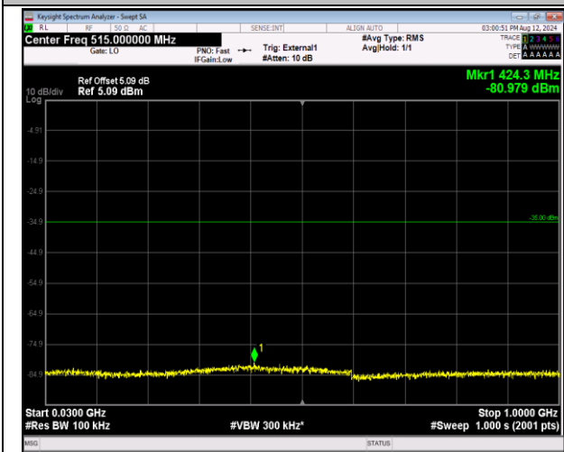
41-41-20MHz-10MHz-QPSK-QPSK-40571-40715-1RB#0 -0RB#0-30~1000MHz-PASS
