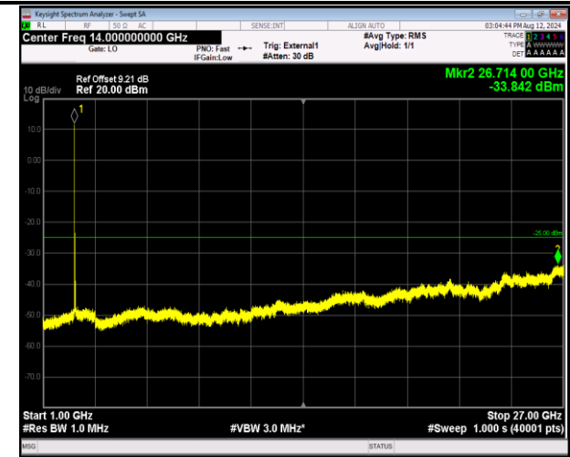
41-41-20MHz-10MHz-QPSK-QPSK-40571-40715-1RB#0-1 RB#49-1000~27000MHz-PASS
