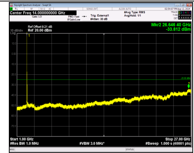
41-41-20MHz-10MHz-QPSK-QPSK-39750-39894-1RB#0-0 RB#0-1000~27000MHz-PASS
