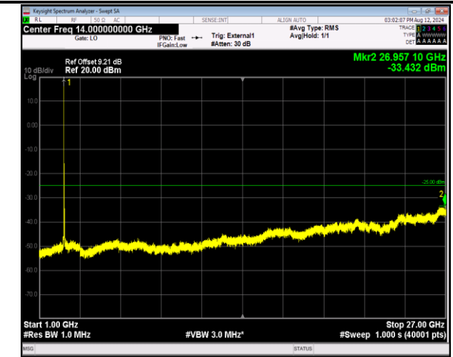
41-41-20MHz-10MHz-16QAM-16QAM-40571-40715-1RB#0 -ORB#0-1000~27000MHz-PASS
