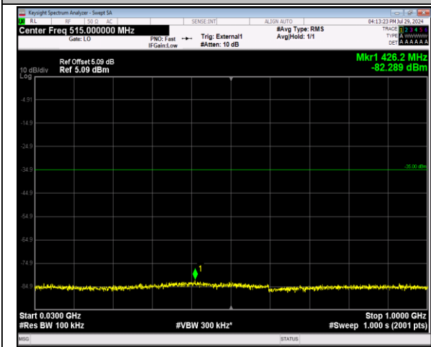
41-41-20MHz-10MHz-64QAM-64QAM-40571-40715-1RB #0-0RB#0-30~1000MHz-PASS
