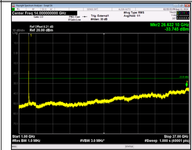
41-41-20MHz-10MHz-QPSK-QPSK-39750-39894-1RB#99- ORB#0-1000~27000MHz-PASS
