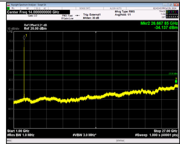
41-41-5MHz-20MHz-64QAM-64QAM-41373-41490-1RB#0- 1RB#99-1000~27000MHz-PASS
