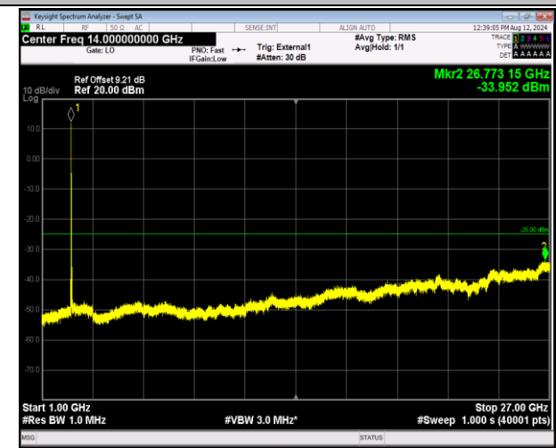
41-41-5MHz-20MHz-16QAM-16QAM-39683-39800-1RB#0- 1RB#99-1000~27000MHz-PASS
