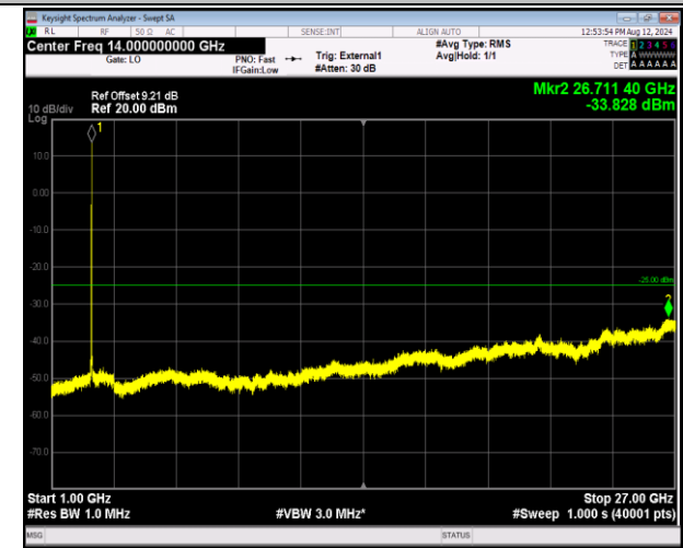
41-41-5MHz-20MHz-QPSK-QPSK-41373-41490-25RB#0-100RB#0-1000~27000MHz-PASS
