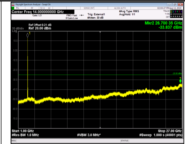
41-41-20MHz-5MHz-QPSK-QPSK-39750-39867-1RB#0-1RB#24-1000~27000MHz-PASS
