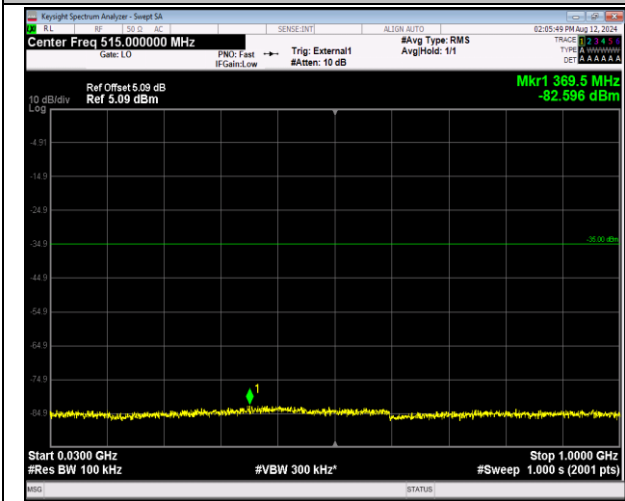
41-41-20MHz-5MHz-QPSK-QPSK-39750-39867-100RB#0-25RB#0-30~1000MHz-PASS
