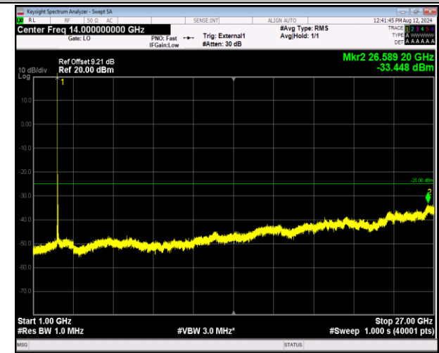
41-41-5MHz-20MHz-QPSK-QPSK-40528-40645-1RB#0-ORB#0-1000~27000MHz-PASS
