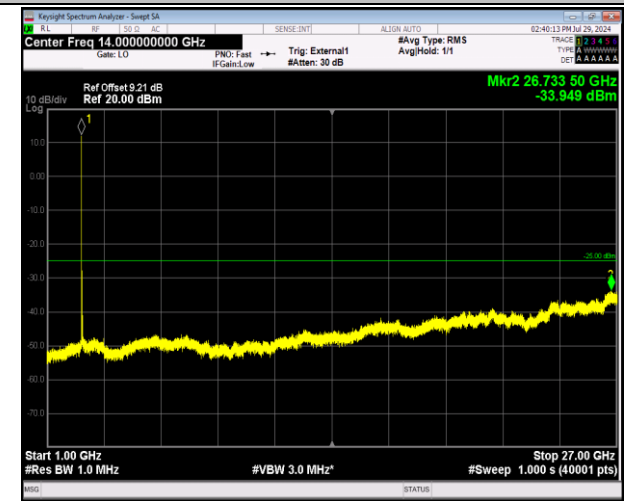
41-41-5MHz-20MHz-64QAM-64QAM-40528-40645-1RB#0- 1RB#99-1000~27000MHz-PASS
