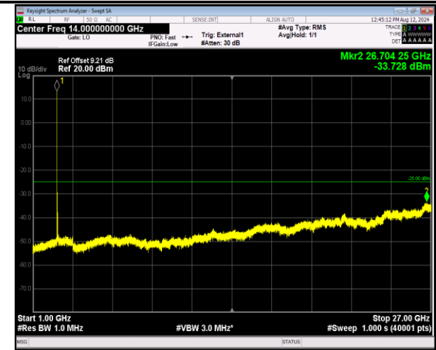
41-41-5MHz-20MHz-QPSK-QPSK-40528-40645-1RB#0-1RB#99-1000~27000MHz-PASS
