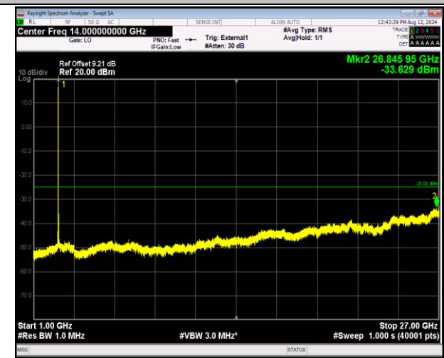
41-41-5MHz-20MHz-QPSK-QPSK-40528-40645-1RB#24-0RB#0-1000~27000MHz-PASS
