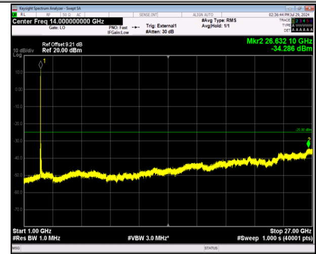
41-41-5MHz-20MHz-64QAM-64QAM-39683-39800-1RB#0-0-1RB#99-1000~27000MHz-PASS
