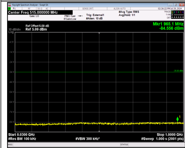
41-41-5MHz-20MHz-64QAM-64QAM-39683-39800-1RB#0-0-1RB#99-30~1000MHz-PASS
