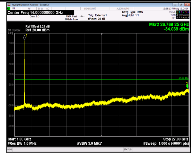
41-41-5MHz-20MHz-QPSK-QPSK-39683-39800-1RB#0-1RB#99-1000~27000MHz-PASS
