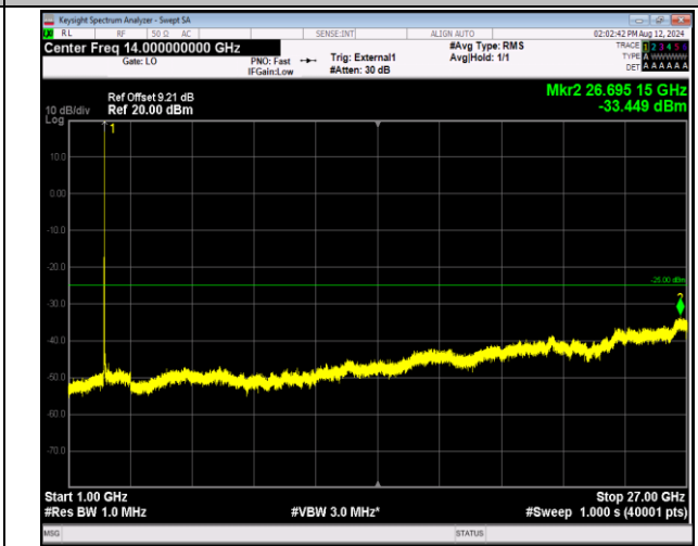
41-41-20MHz-5MHz-QPSK-QPSK-39750-39867-1RB#99-0RB#0-1000~27000MHz-PASS
