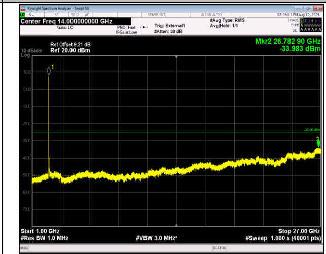
41-41-20MHz-5MHz-QPSK-QPSK-39750-39867-100RB#0-25RB#0-1000~27000MHz-PASS
