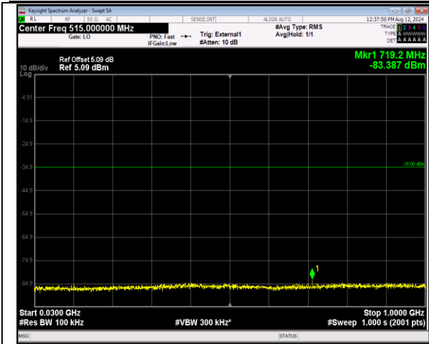
41-41-5MHz-20MHz-QPSK-QPSK-39683-39800-1RB#0-1RB#99-30~1000MHz-PASS
