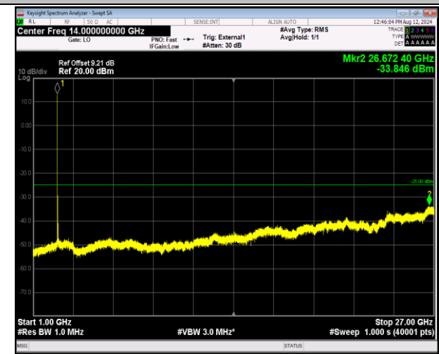
41-41-5MHz-20MHz-16QAM-16QAM-40528-40645-1RB#0- 1RB#99-1000~27000MHz-PASS
