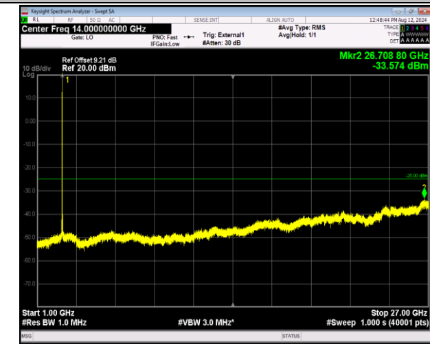
41-41-5MHz-20MHz-QPSK-QPSK-41373-41490-1RB#0-ORB#0-1000~27000MHz-PASS
