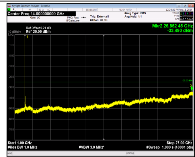
41-41-5MHz-20MHz-QPSK-QPSK-39683-39800-1RB#24-0RB#0-1000~27000MHz-PASS
