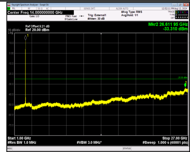
41-41-5MHz-20MHz-QPSK-QPSK-41373-41490-1RB#0-1RB#99-1000~27000MHz-PASS
