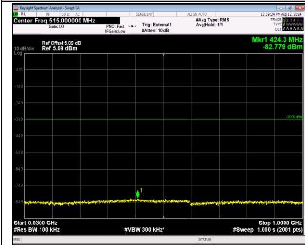
41-41-5MHz-20MHz-QPSK-QPSK-39683-39800-25RB#0-100RB#0-30~1000MHz-PASS
