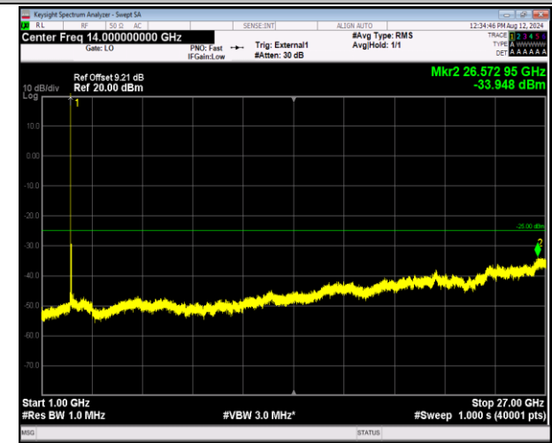
41-41-5MHz-20MHz-QPSK-QPSK-39683-39800-1RB#0-0R B#0-1000~27000MHz-PASS
