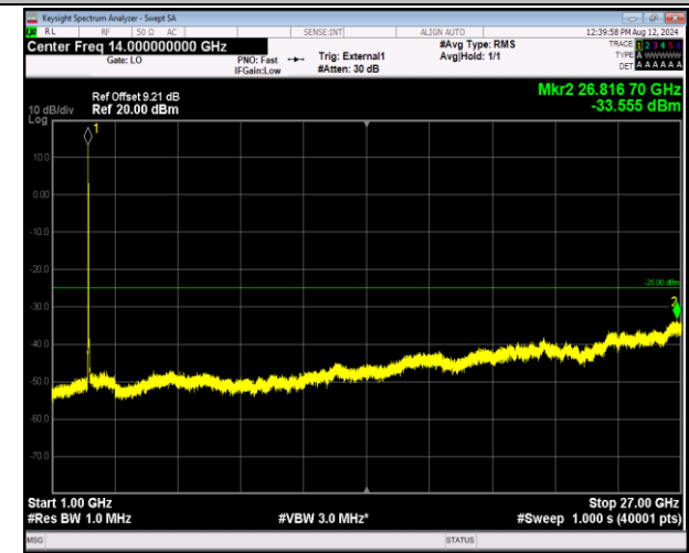
41-41-5MHz-20MHz-QPSK-QPSK-39683-39800-25RB#0-100RB#0-1000~27000MHz-PASS
