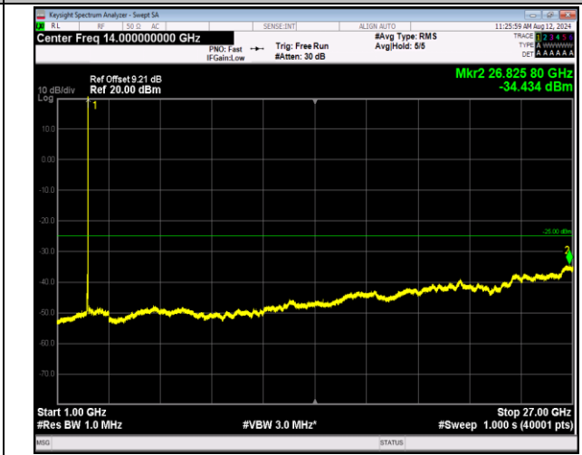
7-7-20MHz-10MHz-QPSK-QPSK-21251-21395-1RB#99-0RB#0-1000~27000MHz-PASS
