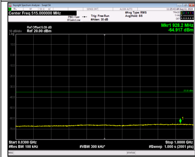
7-7-20MHz-10MHz-QPSK-QPSK-21251-21395-1RB#99-0RB#0-30~1000MHz-PASS
