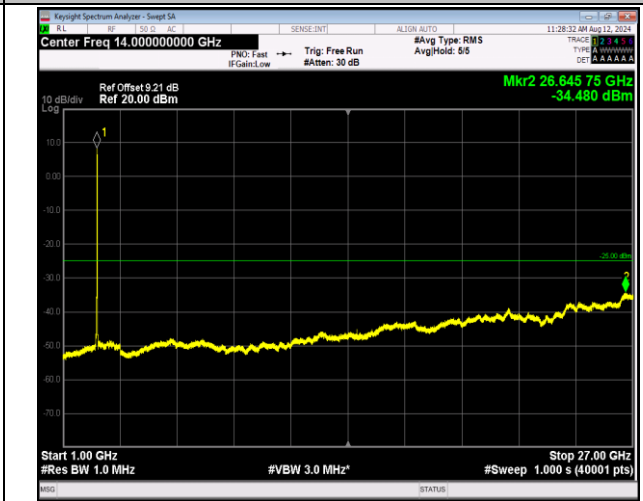
7-7-20MHz-10MHz-QPSK-QPSK-21251-21395-100RB#0-5ORB#0-1000~27000MHz-PASS
