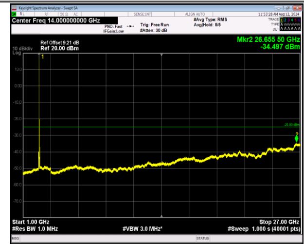
7-7-20MHz-20MHz-QPSK-QPSK-21001-21199-1RB#0-ORB #0-1000~27000MHz-PASS
