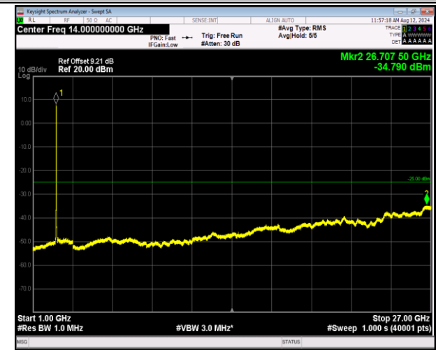
7-7-20MHz-20MHz-QPSK-QPSK-21001-21199-100RB#0-1 00RB#0-1000~27000MHz-PASS
