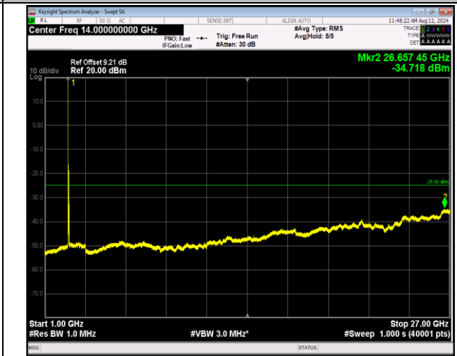
7-7-20MHz-20MHz-QPSK-QPSK-20850-21048-1RB#0-0RB #0-1000~27000MHz-PASS
