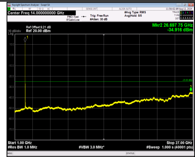
7-7-20MHz-20MHz-QPSK-QPSK-21001-21199-1RB#0-1RB #99-1000~27000MHz-PASS
