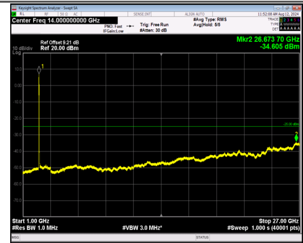
7-7-20MHz-20MHz-QPSK-QPSK-20850-21048-100RB#0-1 00RB#0-1000~27000MHz-PASS
