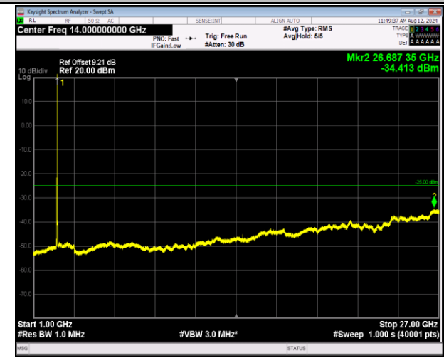
7-7-20MHz-20MHz-QPSK-QPSK-20850-21048-1RB#99-0R B#0-1000~27000MHz-PASS
