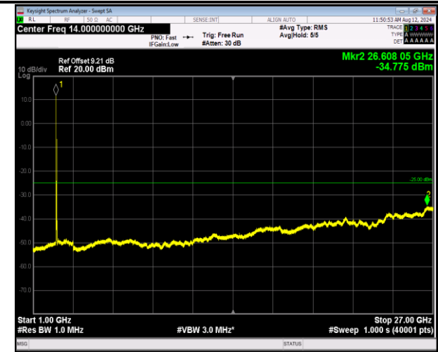
7-7-20MHz-20MHz-QPSK-QPSK-20850-21048-1RB#0-1RB #99-1000~27000MHz-PASS
