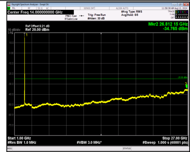
7-7-20MHz-20MHz-QPSK-QPSK-21152-21350-1RB#0-ORB #0-1000~27000MHz-PASS
