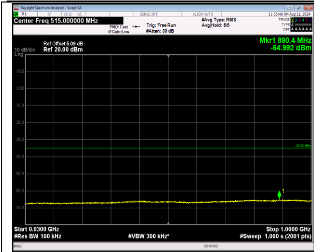
7-7-20MHz-20MHz-QPSK-QPSK-21001-21199-1RB#0-1 RB#99-30~1000MHz-PASS
