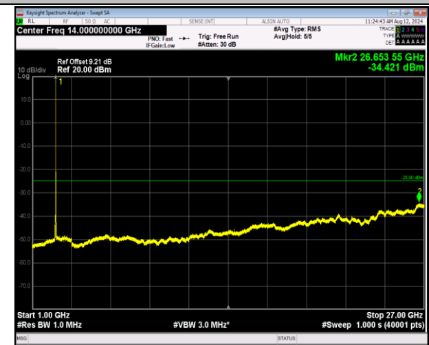
7-7-20MHz-10MHz-QPSK-QPSK-21251-21395-1RB#0-0RB #0-1000~27000MHz-PASS
