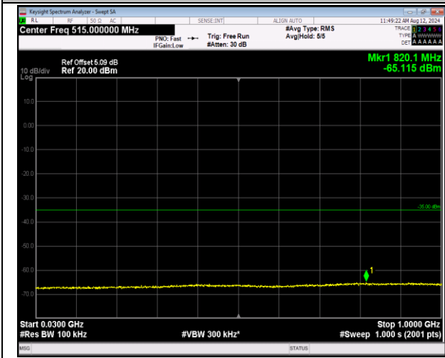
7-7-20MHz-20MHz-QPSK-QPSK-20850-21048-1RB#99-0R 0RB#0-30~1000MHz-PASS
