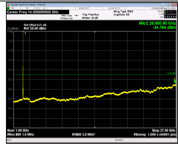
7-7-20MHz-20MHz-QPSK-QPSK-21001-21199-1RB#99-0R B#0-1000~27000MHz-PASS
