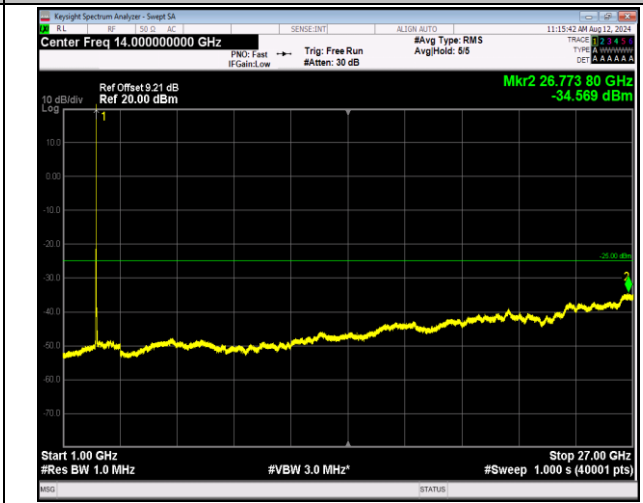
7-7-20MHz-10MHz-QPSK-QPSK-20850-20994-1RB#99-0R B#0-1000~27000MHz-PASS
