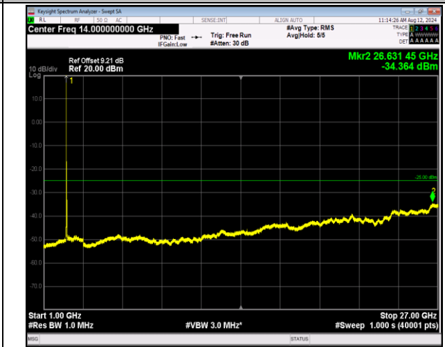
7-7-20MHz-10MHz-QPSK-QPSK-20850-20994-1RB#0-0RB #0-1000~27000MHz-PASS
