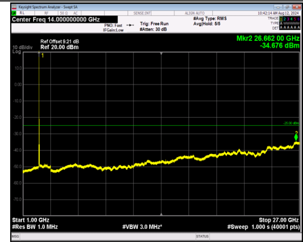
7-7-10MHz-20MHz-QPSK-QPSK-21006-21150-1RB#0-0RB #0-1000~27000MHz-PASS
