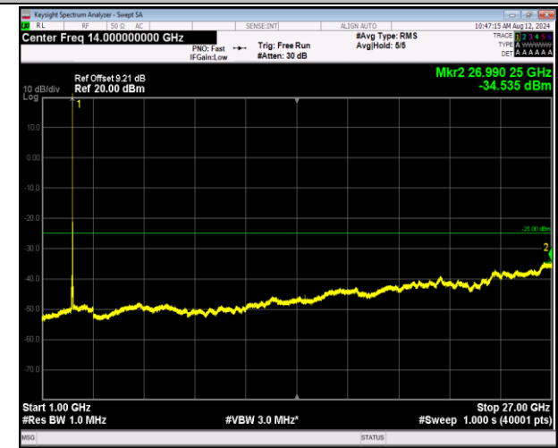
7-7-10MHz-20MHz-QPSK-QPSK-21206-21350-1RB#0-0RB #0-1000~27000MHz-PASS
