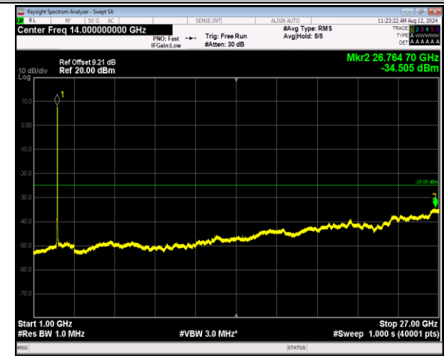
7-7-20MHz-10MHz-QPSK-QPSK-21051-21195-100RB#0-5ORB#0-1000~27000MHz-PASS
