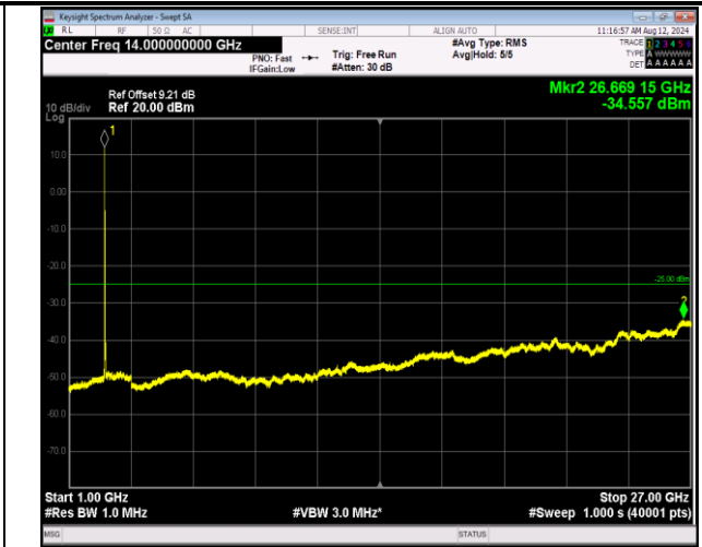
7-7-20MHz-10MHz-QPSK-QPSK-20850-20994-1RB#0-1RB #49-1000~27000MHz-PASS
