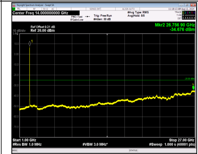
7-7-20MHz-10MHz-QPSK-QPSK-20850-20994-100RB#0-5 ORB#0-1000~27000MHz-PASS
