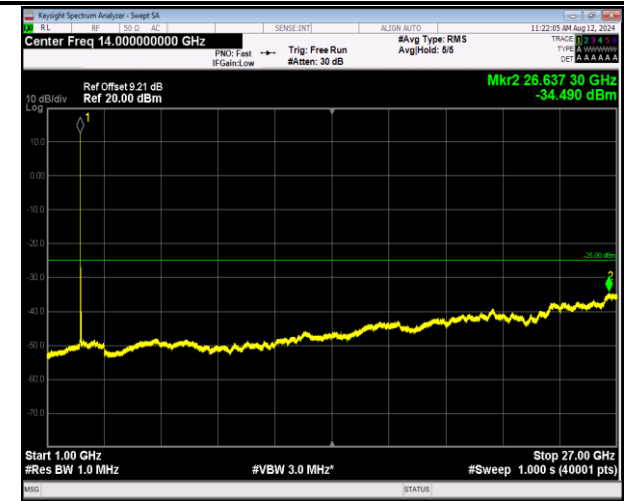
7-7-20MHz-10MHz-QPSK-QPSK-21051-21195-1RB#0-1RB #49-1000~27000MHz-PASS
