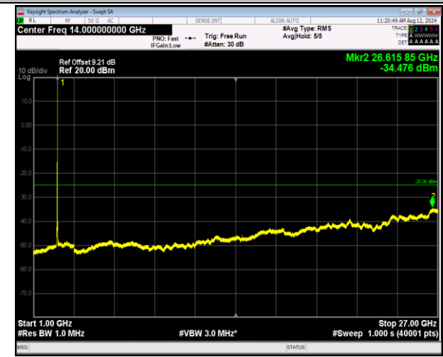
7-7-20MHz-10MHz-QPSK-QPSK-21051-21195-1RB#99-0R B#0-1000~27000MHz-PASS
