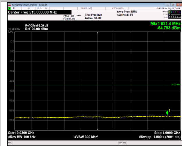
7-7-10MHz-20MHz-QPSK-QPSK-20805-20949-50RB#0-100RB#0-30~1000MHz-PASS
