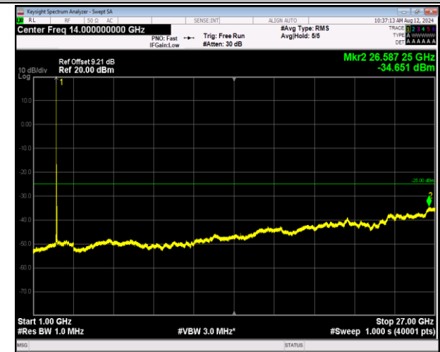
7-7-10MHz-20MHz-QPSK-QPSK-20805-20949-1RB#0-ORB #0-1000~27000MHz-PASS
