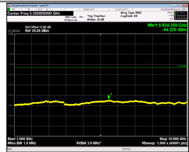
5-5-10MHz-10MHz-QPSK-QPSK-20501-20600-50RB#0-50RB#0-1000~10000MHz-PASS
