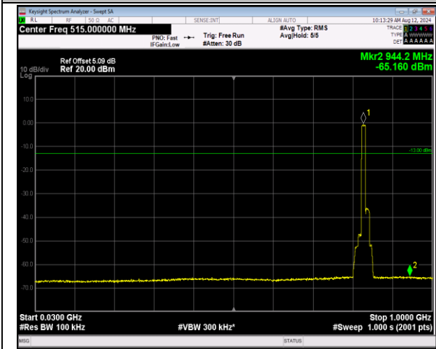
5-5-10MHz-10MHz-QPSK-QPSK-20476-20575-50RB#0-0-50RB#0-30~1000MHz-PASS
