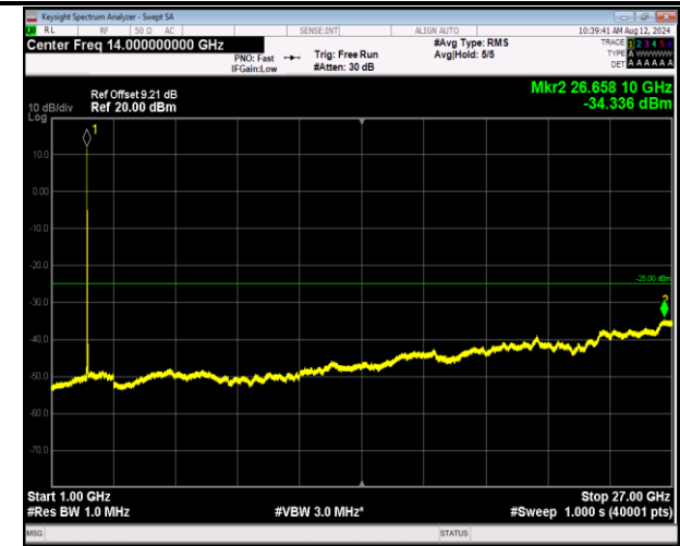
7-7-10MHz-20MHz-QPSK-QPSK-20805-20949-1RB#0-1RB #99-1000~27000MHz-PASS
