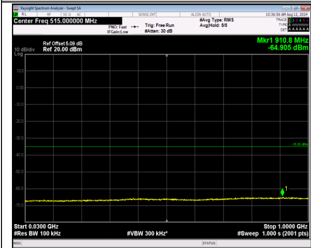
7-7-10MHz-20MHz-QPSK-QPSK-20805-20949-1RB#0-0 RB#0-30~1000MHz-PASS
