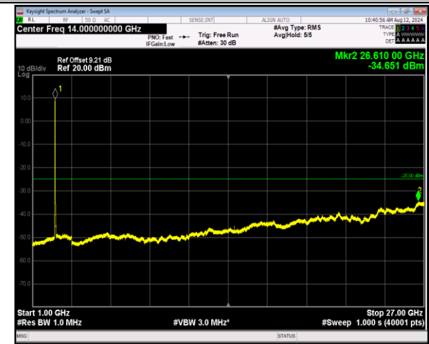
7-7-10MHz-20MHz-QPSK-QPSK-20805-20949-50RB#0-100RB#0-1000~27000MHz-PASS
