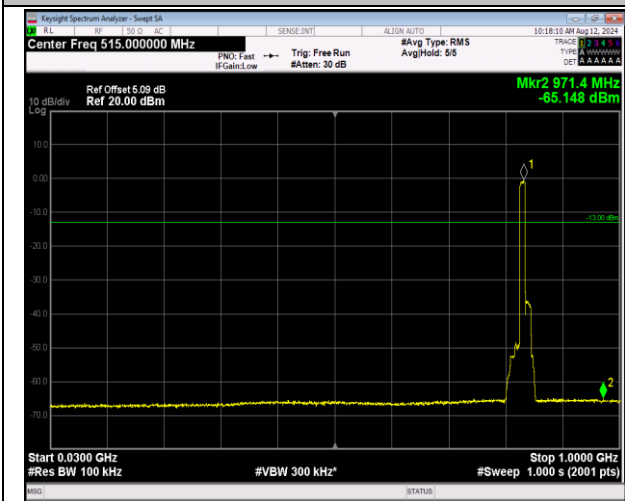
5-5-10MHz-10MHz-QPSK-QPSK-20501-20600-50RB#0-0-50RB#0-30~1000MHz-PASS
