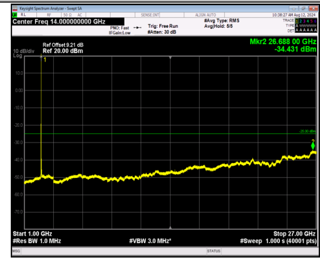
7-7-10MHz-20MHz-QPSK-QPSK-20805-20949-1RB#49-0RB#0-1000~27000MHz-PASS
