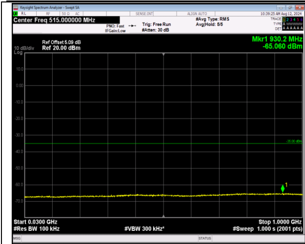
7-7-10MHz-20MHz-QPSK-QPSK-20805-20949-1RB#0-1 RB#99-30~1000MHz-PASS
