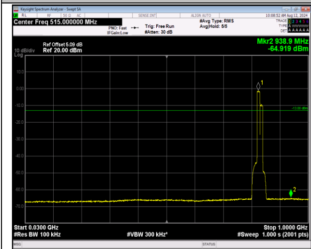
5-5-10MHz-10MHz-QPSK-QPSK-20450-20549-50RB#0-0-50RB#0-30~1000MHz-PASS
