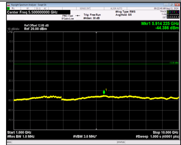
5-5-3MHz-5MHz-QPSK-QPSK-20586-20625-15RB#0-25RB #0-1000~10000MHz-PASS
