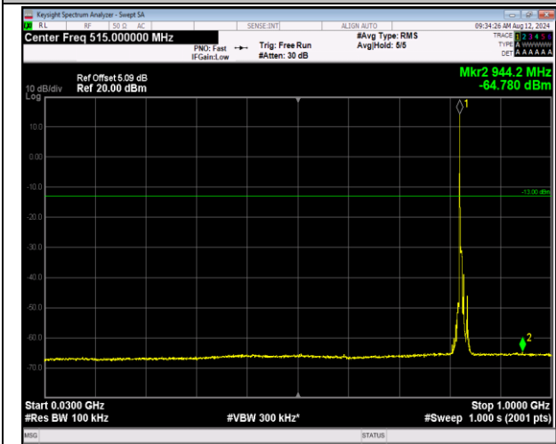
5-5-5MHz-3MHz-QPSK-QPSK-20425-20464-1RB#0-0RB#0-30~1000MHz-PASS
