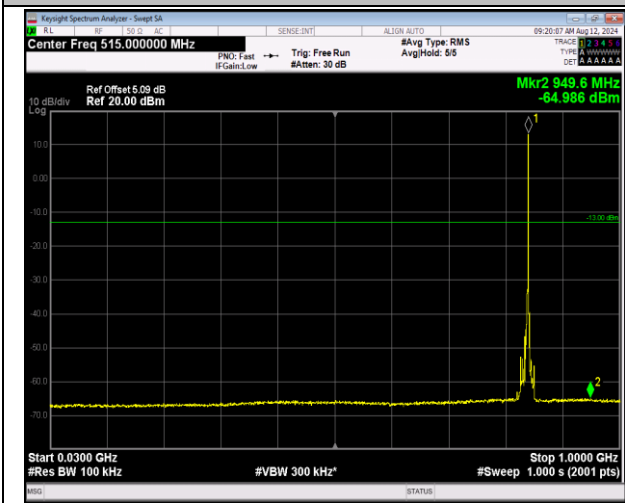
5-5-3MHz-5MHz-QPSK-QPSK-20586-20625-1RB#14-0R B#0-30~1000MHz-PASS
