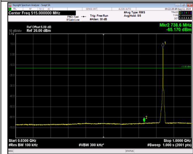
5-5-3MHz-5MHz-QPSK-QPSK-20586-20625-15RB#0-25 RB#0-30~1000MHz-PASS
