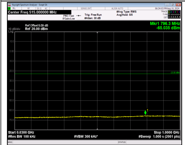
2-2-5MHz-20MHz-QPSK-QPSK-18808-18925-1RB#0-0R B#0-30~1000MHz-PASS
