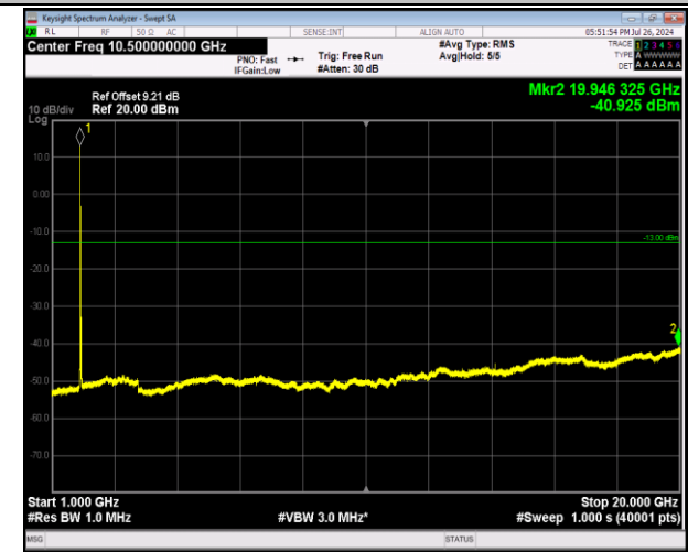
2-2-5MHz-20MHz-64QAM-64QAM-18633-18750-1RB#0-1R B#99-1000~20000MHz-PASS
