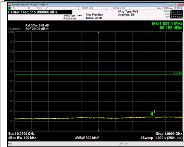
2-2-5MHz-20MHz-QPSK-QPSK-18983-19100-1RB#0-1R B#99-30~1000MHz-PASS
