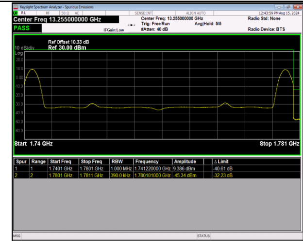
66-66-20MHz-20MHz-QPSK@QPSK-QPSK@QPSK-1323
