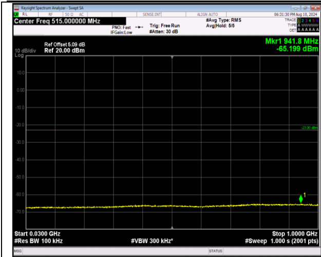
2-2-5MHz-20MHz-QPSK-QPSK-18633-18750-1RB#0-1R B#99-30~1000MHz-PASS
