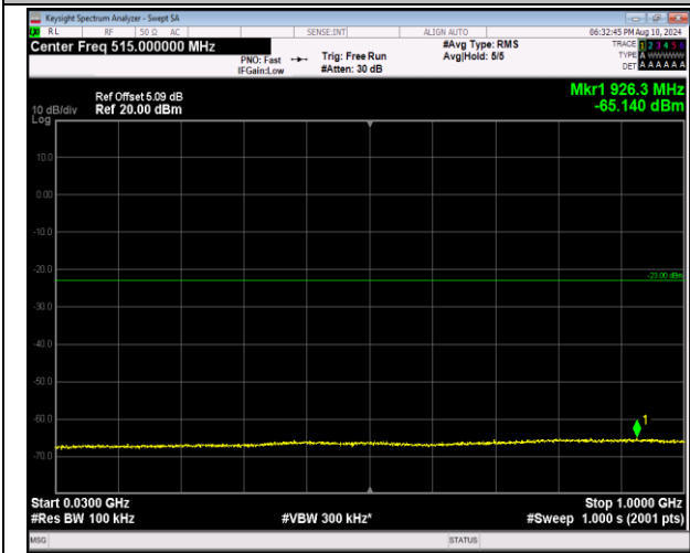
2-2-5MHz-20MHz-QPSK-QPSK-18633-18750-25RB#0-1 00RB#0-30~1000MHz-PASS
