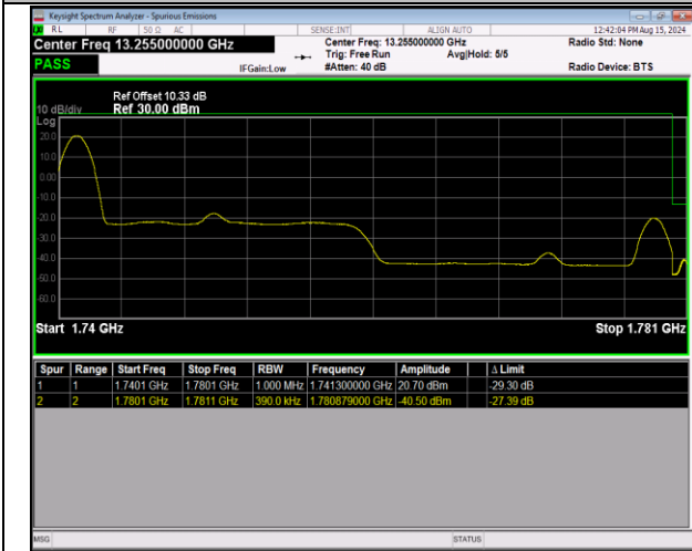
66-66-20MHz-20MHz-QPSK@QPSK-QPSK@QPSK-132
