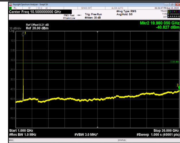
2-2-5MHz-20MHz-QPSK-QPSK-18808-18925-1RB#0-1RB# 99-1000~20000MHz-PASS
