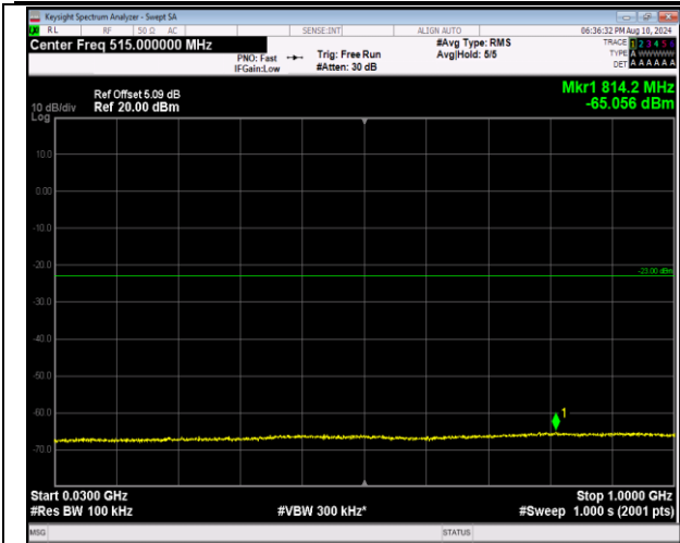
2-2-5MHz-20MHz-QPSK-QPSK-18808-18925-1RB#0-1R B#99-30~1000MHz-PASS
