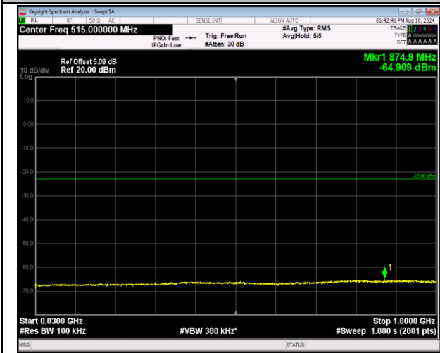
2-2-5MHz-20MHz-QPSK-QPSK-18983-19100-25RB#0-1 00RB#0-30~1000MHz-PASS
