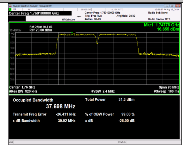
66-66-20MHz-20MHz-QPSK-QPSK-132374-132572-100R B#0-100RB#0-PASS
