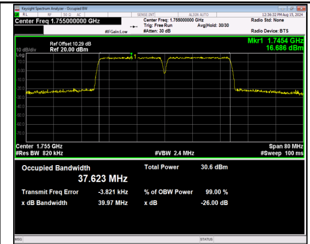
66-66-20MHz-20MHz-16QAM-16QAM-132323-132521-10 ORB#0-100RB#0-PASS
