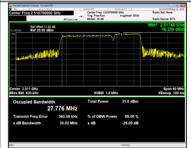
41-41-20MHz-10MHz-QPSK-QPSK-39750-39894-100RB#0-50RB#0-PASS
