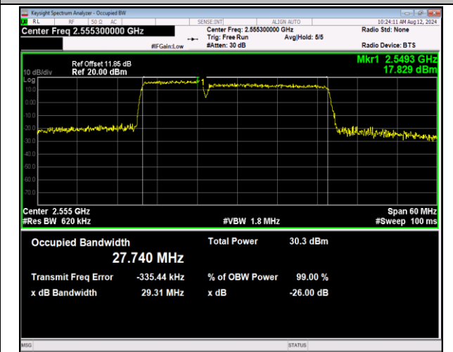
7-7-10MHz-20MHz-QPSK-QPSK-21206-21350-50RB#0-1 00RB#0-PASS
