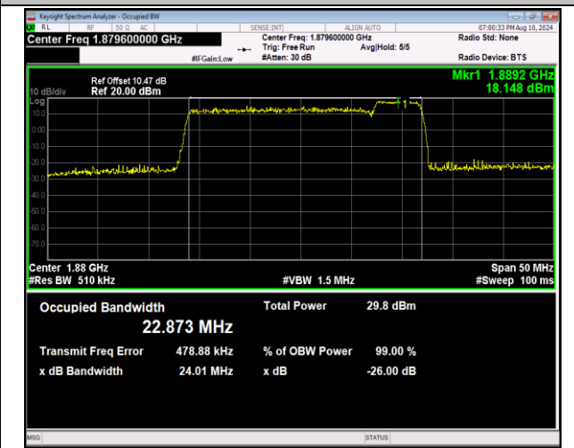
2-2-20MHz-5MHz-QPSK-QPSK-18875-18992-100RB#0-25RB#0-PASS
