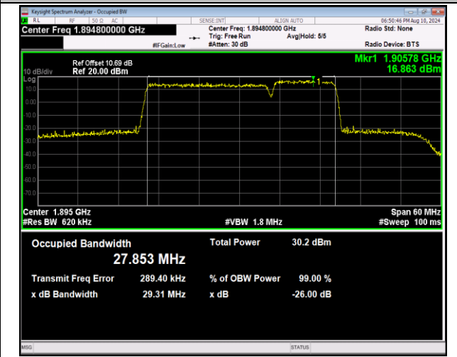
2-2-20MHz-10MHz-QPSK-QPSK-19001-19145-100RB#0-50RB#0-PASS
