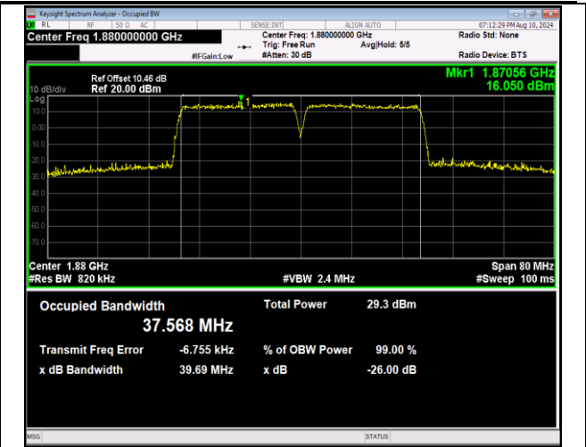
2-2-20MHz-20MHz-16QAM-16QAM-18801-18999-100RB#0-100RB#0-PASS
