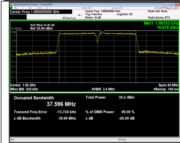
2-2-20MHz-20MHz-QPSK-QPSK-18801-18999-100RB#0-100RB#0-PASS
