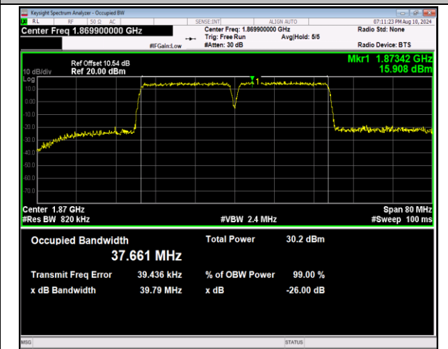
2-2-20MHz-20MHz-QPSK-QPSK-18700-18898-100RB#0-100RB#0-PASS
