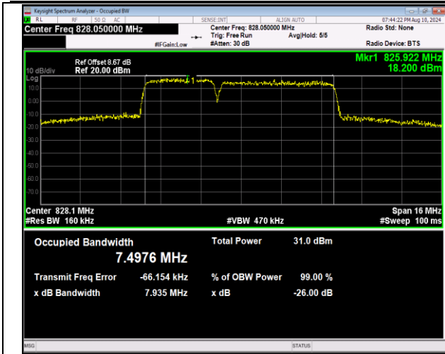
5-5-3MHz-5MHz-QPSK-QPSK-20416-20455-15RB#0-25R B#0-PASS
