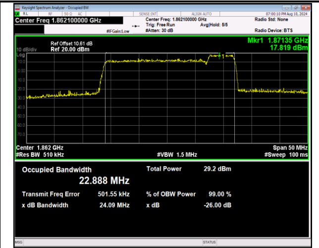
2-2-20MHz-5MHz-16QAM-16QAM-18700-18817-100RB#0-25RB#0-PASS
