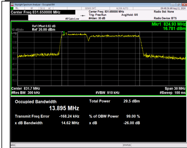
5-5-5MHz-10MHz-QPSK-QPSK-20428-20500-25RB#0-50 RB#0-PASS
