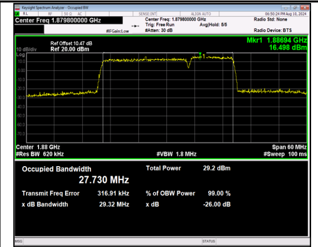
2-2-20MHz-10MHz-16QAM-16QAM-18851-18995-100RB#0-50RB#0-PASS
