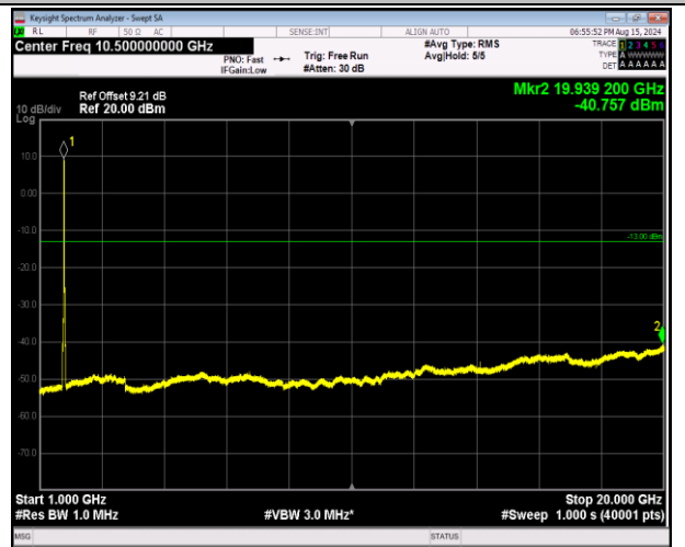
66-66-20MHz-20MHz-QPSK-QPSK-132323-132521-100RB #0-100RB#0-1000~20000MHz-PASS
