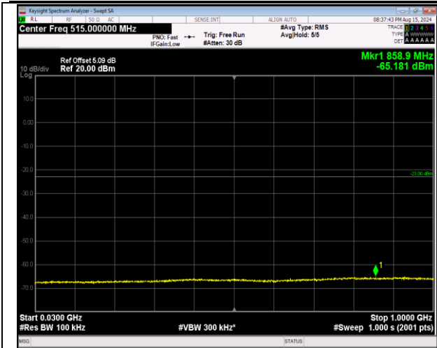
66-66-20MHz-20MHz-64QAM-64QAM-132072-132270-1 RB#99-0RB#0-30~1000MHz-PASS
