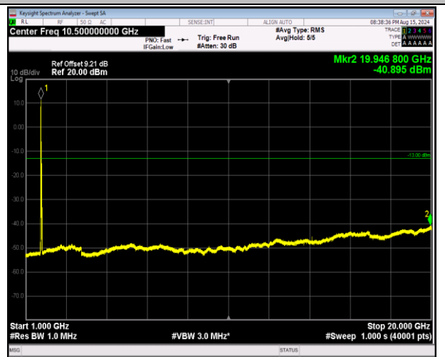
66-66-20MHz-20MHz-64QAM-64QAM-132072-132270-1RB#0-1RB#99-1000~20000MHz-PASS
