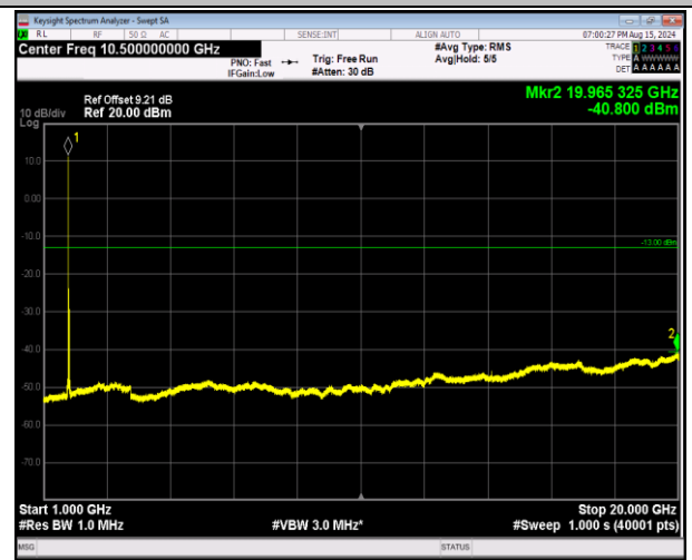
66-66-20MHz-20MHz-16QAM-16QAM-132374-132572-1RB #0-1RB#99-1000~20000MHz-PASS
