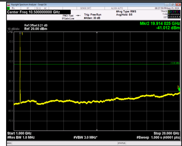
66-66-20MHz-20MHz-64QAM-64QAM-132072-132270-1RB #99-0RB#0-1000~20000MHz-PASS
