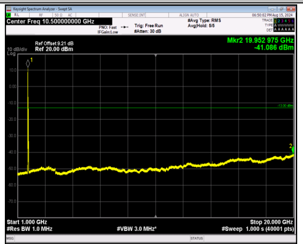
66-66-20MHz-20MHz-16QAM-16QAM-132072-132270-1RB #0-1RB#99-1000~20000MHz-PASS
