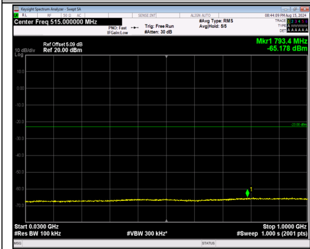
66-66-20MHz-20MHz-64QAM-64QAM-132374-132572-1 00RB#0-100RB#0-30~1000MHz-PASS
