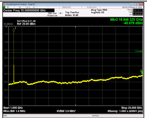
66-66-20MHz-20MHz-16QAM-16QAM-132323-132521-1RB #0-1RB#99-1000~20000MHz-PASS
