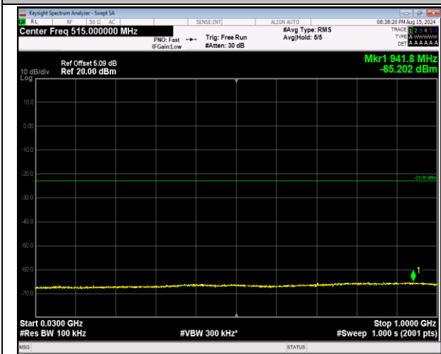
66-66-20MHz-20MHz-64QAM-64QAM-132072-132270-1RB#0-1RB#99-30~1000MHz-PASS
