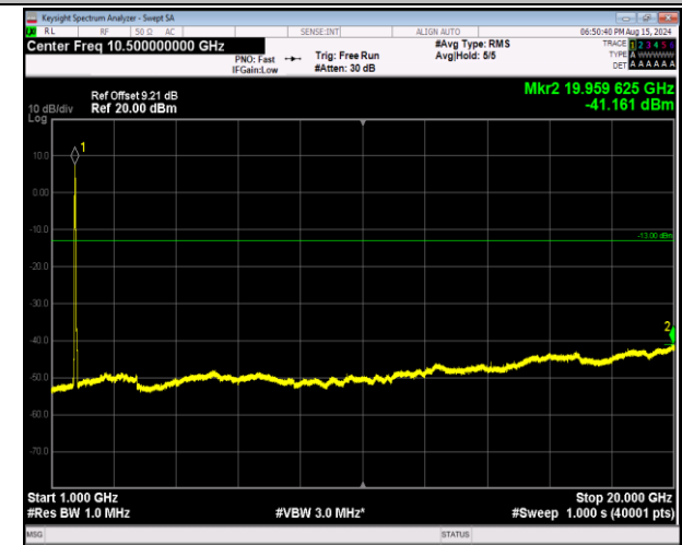
66-66-20MHz-20MHz-QPSK-QPSK-132072-132270-100RB #0-100RB#0-1000~20000MHz-PASS
