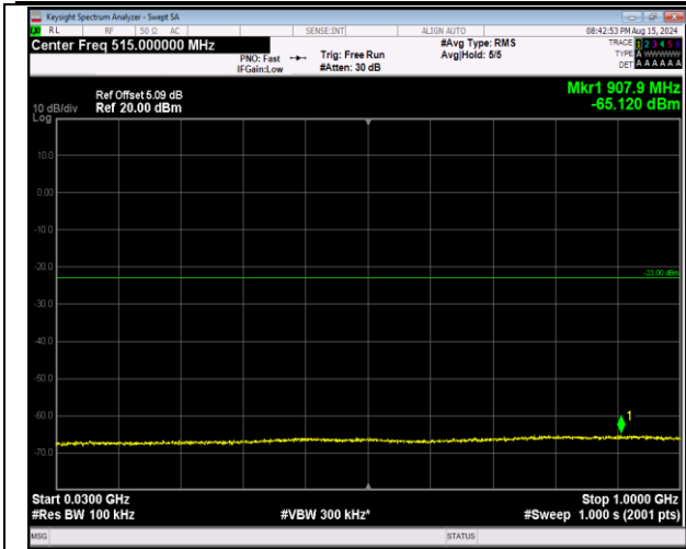
66-66-20MHz-20MHz-64QAM-64QAM-132374-132572-1 RB#99-0RB#0-30~1000MHz-PASS
