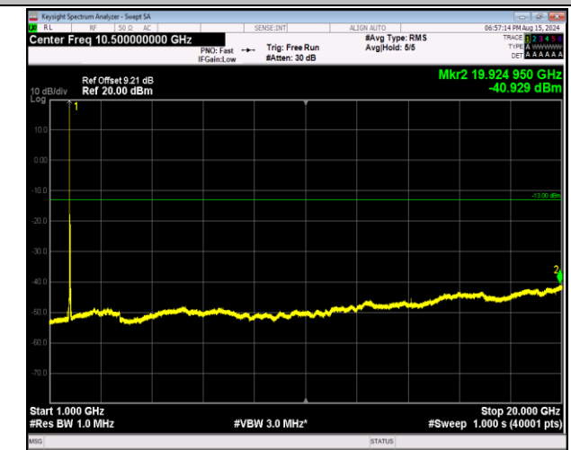
66-66-20MHz-20MHz-QPSK-QPSK-132374-132572-1RB#0 -0RB#0-1000~20000MHz-PASS
