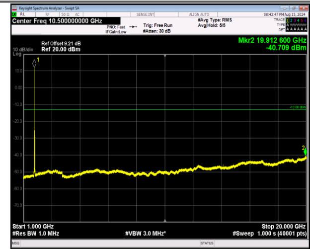
66-66-20MHz-20MHz-64QAM-64QAM-132374-132572-1RB #0-1RB#99-1000~20000MHz-PASS
