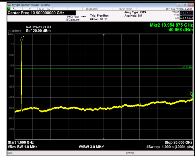
66-66-20MHz-20MHz-QPSK-QPSK-132072-132270-1RB#0 -1RB#99-1000~20000MHz-PASS
