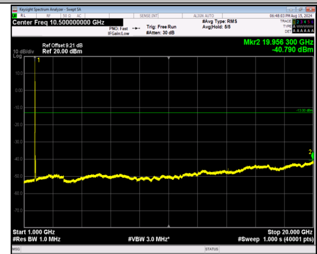
66-66-20MHz-20MHz-QPSK-QPSK-132072-132270-1RB#9 9-0RB#0-1000~20000MHz-PASS
