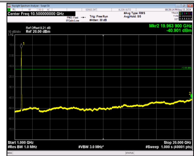
66-66-20MHz-20MHz-64QAM-64QAM-132072-132270-100 RB#0-100RB#0-1000~20000MHz-PASS
