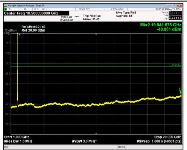
66-66-20MHz-20MHz-QPSK-QPSK-132323-132521-1RB#9 9-0RB#0-1000~20000MHz-PASS
