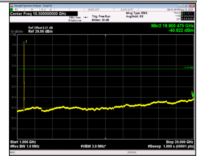
66-66-20MHz-20MHz-64QAM-64QAM-132323-132521-100 RB#0-100RB#0-1000~20000MHz-PASS
