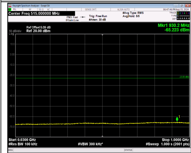
66-66-20MHz-20MHz-QPSK-QPSK-132072-132270-1RB #99-0RB#0-30~1000MHz-PASS
