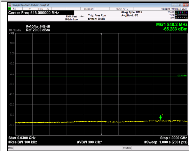
66-66-20MHz-20MHz-QPSK-QPSK-132323-132521-1RB #0-0RB#0-30~1000MHz-PASS
