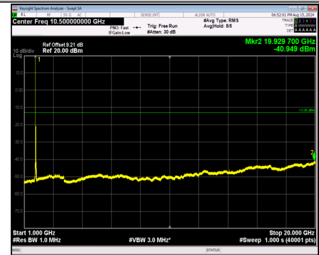
66-66-20MHz-20MHz-QPSK-QPSK-132323-132521-1RB#0 -0RB#0-1000~20000MHz-PASS
