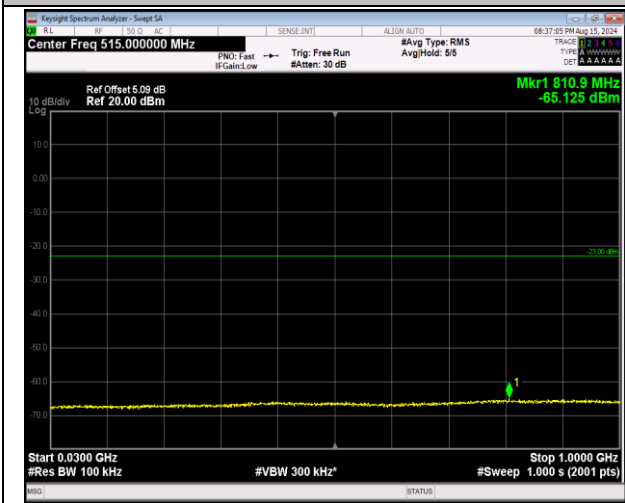
66-66-20MHz-20MHz-64QAM-64QAM-132072-132270-1RB#0-0RB#0-30~1000MHz-PASS
