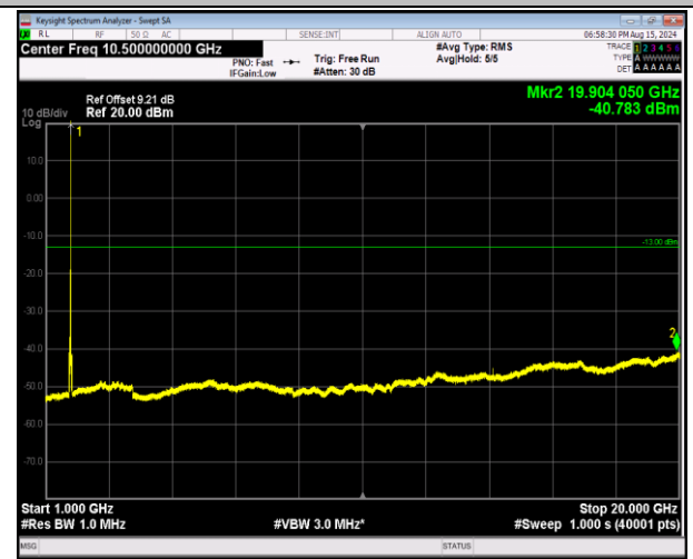
66-66-20MHz-20MHz-QPSK-QPSK-132374-132572-1RB#9 9-0RB#0-1000~20000MHz-PASS
