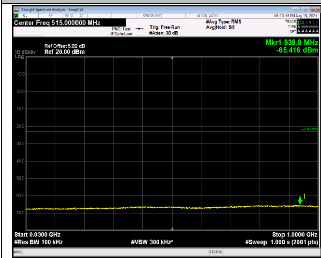
66-66-20MHz-20MHz-16QAM-16QAM-132072-132270-1 RB#0-1RB#99-30~1000MHz-PASS
