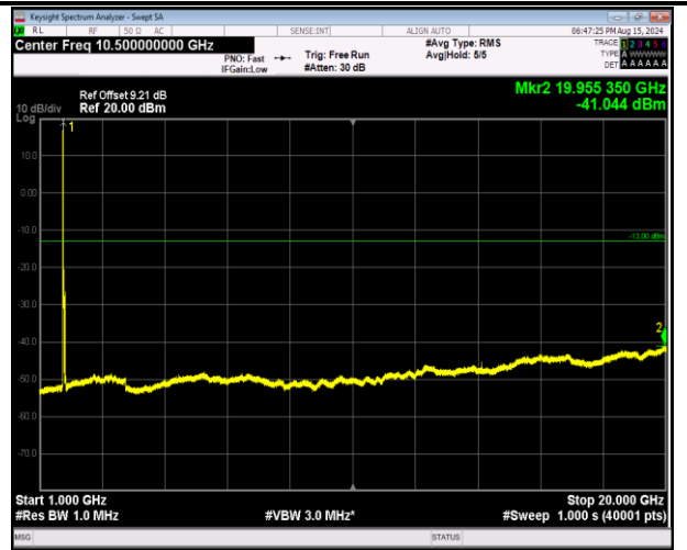
66-66-20MHz-20MHz-16QAM-16QAM-132072-132270-1RB #0-ORB#0-1000~20000MHz-PASS
