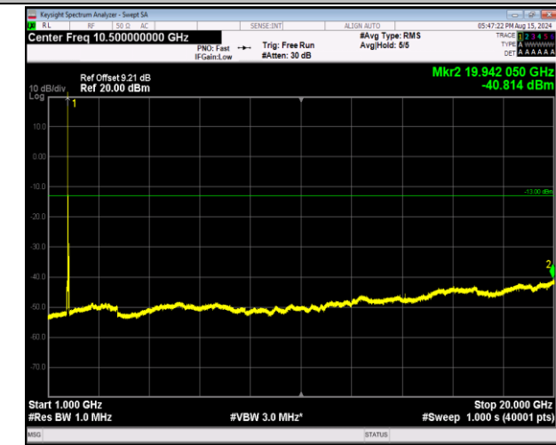
66-66-20MHz-5MHz-QPSK-QPSK-132397-132514-1RB#0- ORB#0-1000~20000MHz-PASS
