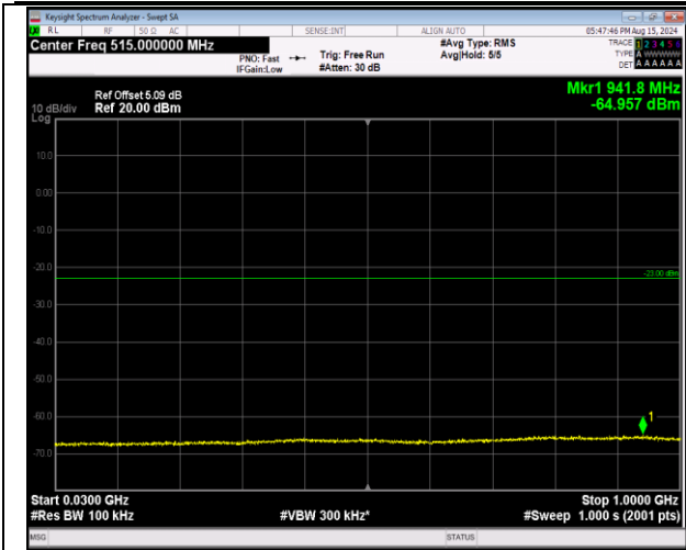
66-66-20MHz-5MHz-16QAM-16QAM-132397-132514-1R B#0-ORB#0-30~1000MHz-PASS
