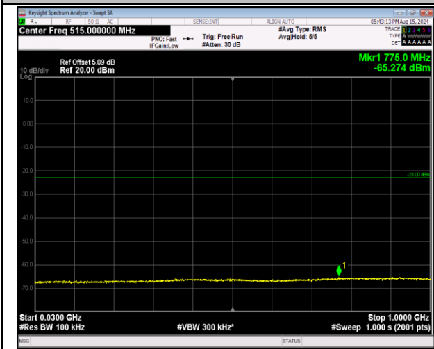
66-66-20MHz-5MHz-QPSK-QPSK-132072-132189-1RB# 99-0RB#0-30~1000MHz-PASS
