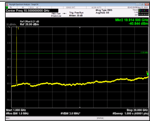
66-66-20MHz-5MHz-QPSK-QPSK-132072-132189-1RB#99 -0RB#0-1000~20000MHz-PASS
