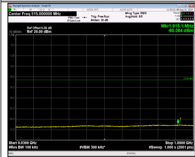
66-66-5MHz-20MHz-16QAM-16QAM-132455-132572-1R B#0-1RB#99-30~1000MHz-PASS
