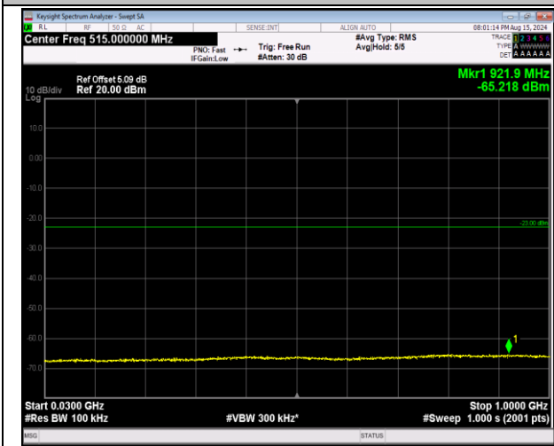
66-66-20MHz-5MHz-64QAM-64QAM-132072-132189-1R B#0-ORB#0-30~1000MHz-PASS
