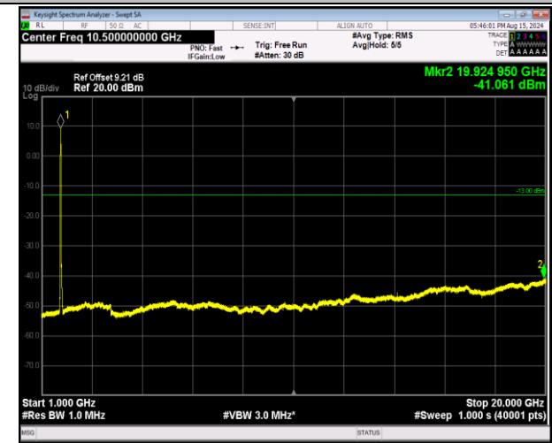
66-66-20MHz-5MHz-QPSK-QPSK-132072-132189-100RB# 0-25RB#0-1000~20000MHz-PASS
