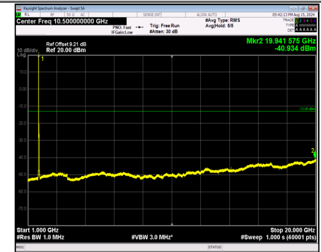
66-66-20MHz-5MHz-QPSK-QPSK-132072-132189-1RB#0- ORB#0-1000~20000MHz-PASS
