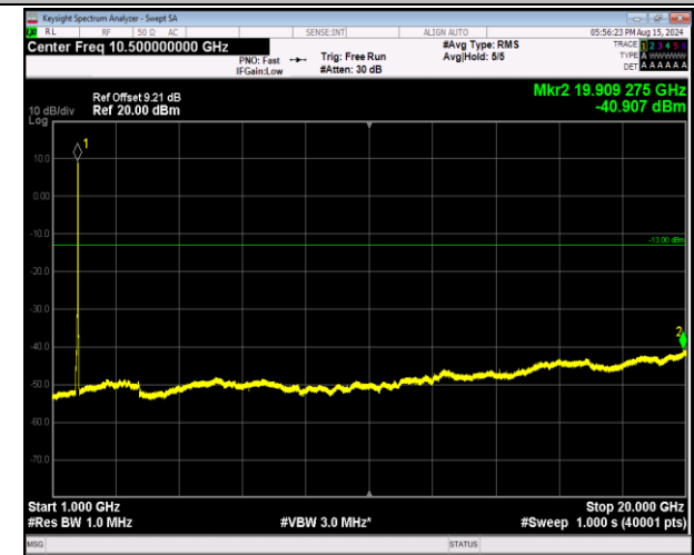
66-66-20MHz-5MHz-QPSK-QPSK-132522-132639-100RB# 0-25RB#0-1000~20000MHz-PASS
