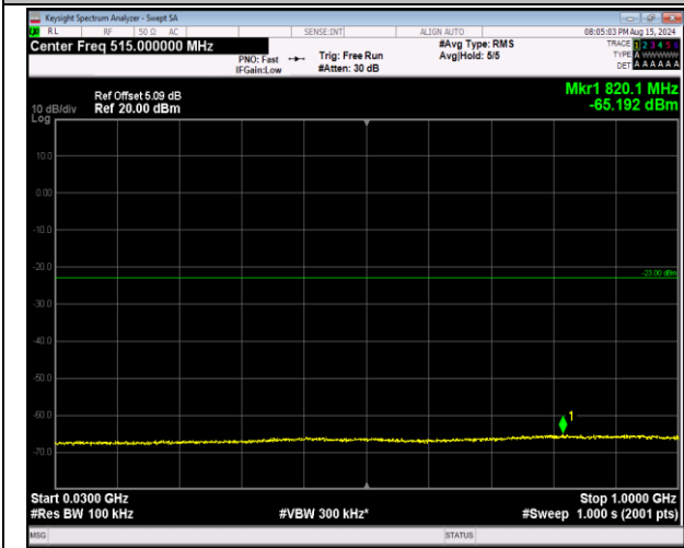
66-66-20MHz-5MHz-64QAM-64QAM-132397-132514-1R B#0-1RB#24-30~1000MHz-PASS
