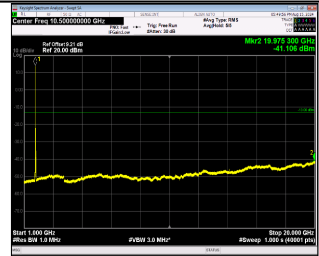
66-66-20MHz-5MHz-QPSK-QPSK-132397-132514-1RB#0- 1RB#24-1000~20000MHz-PASS
