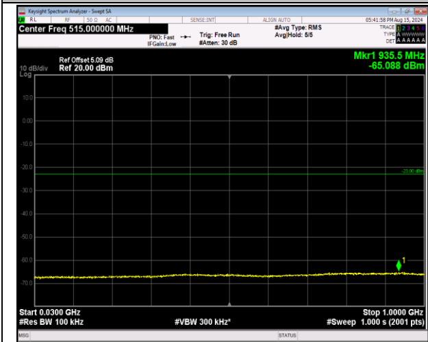
66-66-20MHz-5MHz-QPSK-QPSK-132072-132189-1RB# 0-ORB#0-30~1000MHz-PASS
