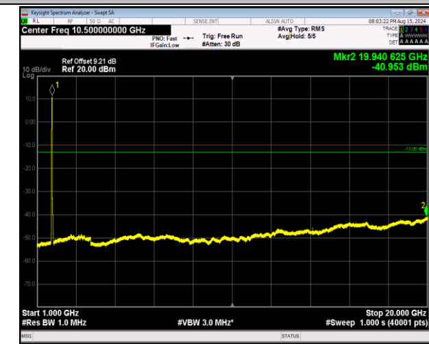
66-66-20MHz-5MHz-64QAM-64QAM-132072-132189-100R B#0-25RB#0-1000~20000MHz-PASS
