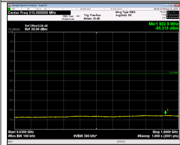
66-66-20MHz-5MHz-64QAM-64QAM-132522-132639-1R B#0-ORB#0-30~1000MHz-PASS
