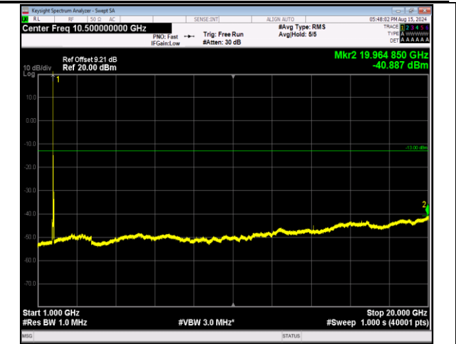
66-66-20MHz-5MHz-16QAM-16QAM-132397-132514-1RB# 0-ORB#0-1000~20000MHz-PASS
