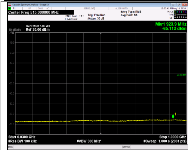
66-66-5MHz-20MHz-64QAM-64QAM-132455-132572-1R B#24-ORB#0-30~1000MHz-PASS
