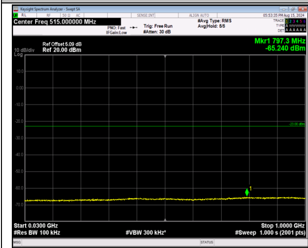
66-66-20MHz-5MHz-QPSK-QPSK-132522-132639-1RB# 99-0RB#0-30~1000MHz-PASS
