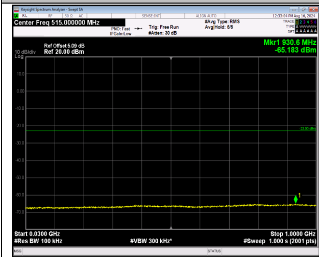
66-66-5MHz-20MHz-64QAM-64QAM-132455-132572-1R B#0-0RB#0-30~1000MHz-PASS
