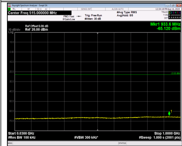
66-66-5MHz-20MHz-64QAM-64QAM-132455-132572-1R B#0-1RB#99-30~1000MHz-PASS
