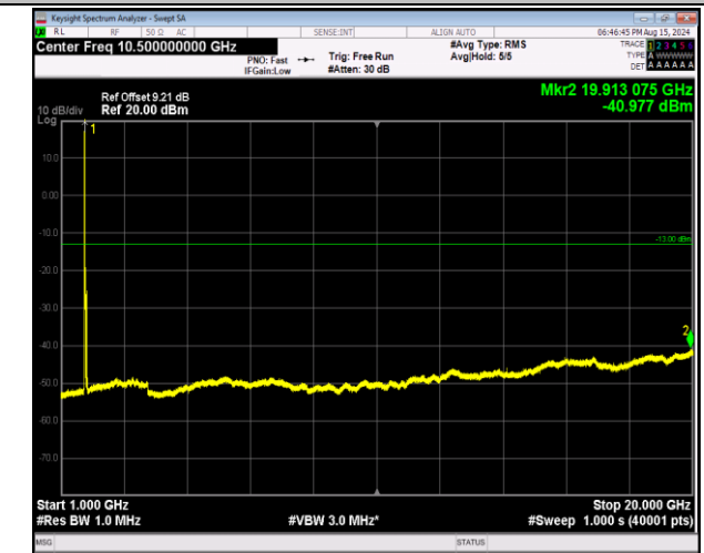
66-66-20MHz-20MHz-QPSK-QPSK-132072-132270-1RB#0 -ORB#0-1000~20000MHz-PASS
