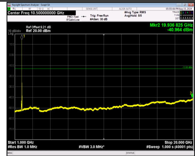
66-66-20MHz-5MHz-QPSK-QPSK-132522-132639-1RB#0- 1RB#24-1000~20000MHz-PASS
