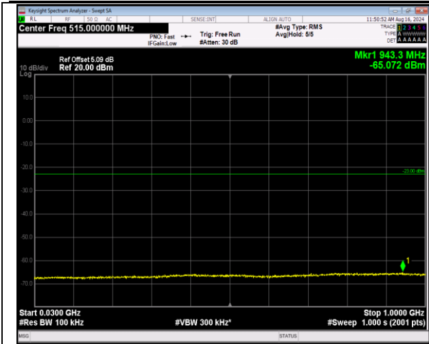
66-66-5MHz-20MHz-16QAM-16QAM-132455-132572-1R B#0-ORB#0-30~1000MHz-PASS
