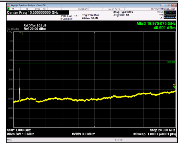
66-66-20MHz-5MHz-QPSK-QPSK-132397-132514-1RB#99 -0RB#0-1000~20000MHz-PASS
