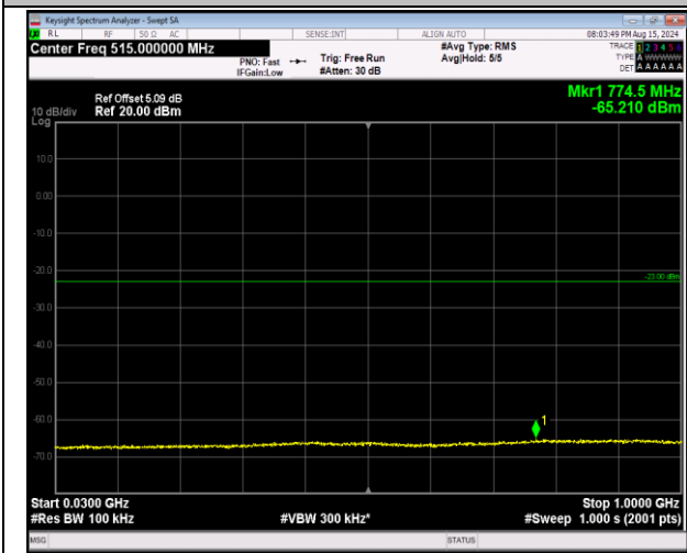
66-66-20MHz-5MHz-64QAM-64QAM-132397-132514-1R B#0-ORB#0-30~1000MHz-PASS
