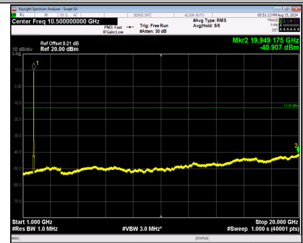
66-66-20MHz-5MHz-QPSK-QPSK-132397-132514-100RB# 0-25RB#0-1000~20000MHz-PASS
