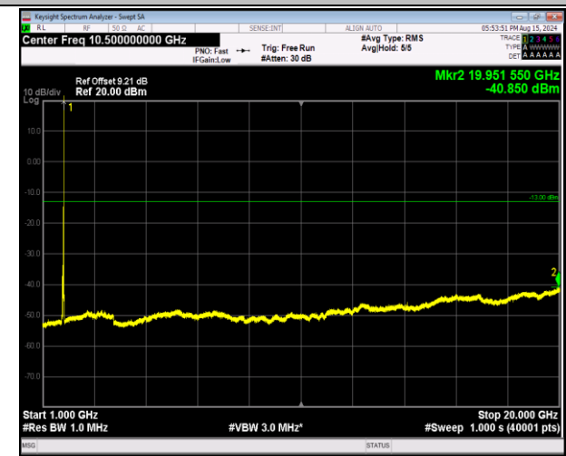
66-66-20MHz-5MHz-QPSK-QPSK-132522-132639-1RB#99 -0RB#0-1000~20000MHz-PASS
