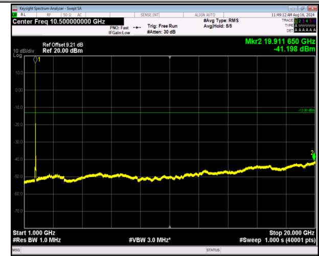
66-66-5MHz-20MHz-QPSK-QPSK-132330-132447-25RB#0-100RB#0-1000~20000MHz-PASS
