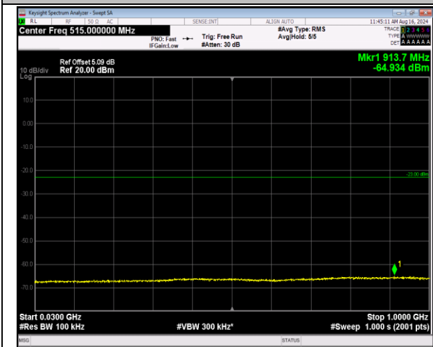
66-66-5MHz-20MHz-QPSK-QPSK-132330-132447-1RB# 0-ORB#0-30~1000MHz-PASS
