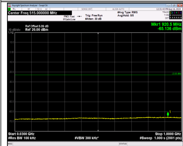
66-66-5MHz-20MHz-64QAM-64QAM-132330-132447-1R B#0-1RB#99-30~1000MHz-PASS
