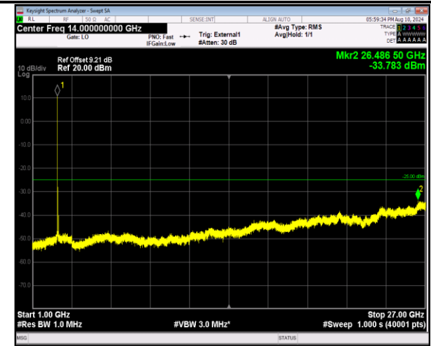
41-41-20MHz-20MHz-QPSK-QPSK-41292-41490-1RB#0-1 RB#99-1000~27000MHz-PASS
