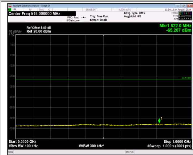
66-66-5MHz-20MHz-QPSK-QPSK-132455-132572-1RB# 0-ORB#0-30~1000MHz-PASS
