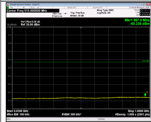
66-66-5MHz-20MHz-QPSK-QPSK-132330-132447-1RB#24-0RB#0-30~1000MHz-PASS
