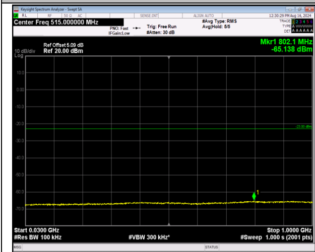
66-66-5MHz-20MHz-64QAM-64QAM-132330-132447-1R B#0-0RB#0-30~1000MHz-PASS
