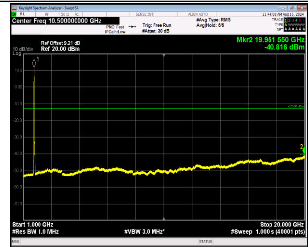
66-66-5MHz-20MHz-QPSK-QPSK-132005-132122-25RB#0 -100RB#0-1000~20000MHz-PASS
