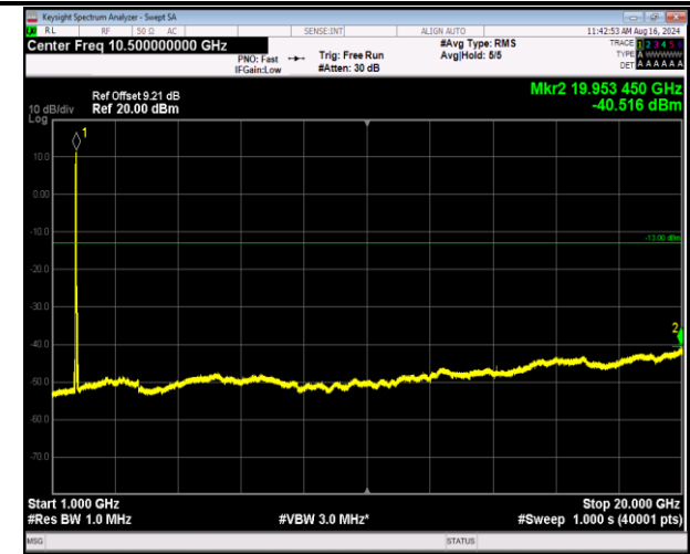
66-66-5MHz-20MHz-QPSK-QPSK-132005-132122-1RB#0- 1RB#99-1000~20000MHz-PASS
