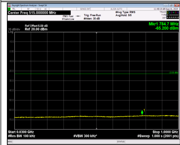
66-66-5MHz-20MHz-16QAM-16QAM-132330-132447-1R B#0-1RB#99-30~1000MHz-PASS
