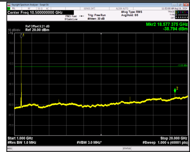
66-66-5MHz-20MHz-QPSK-QPSK-132455-132572-1RB#0- 1RB#99-1000~20000MHz-PASS
