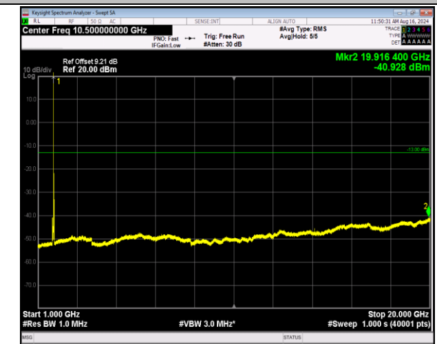
66-66-5MHz-20MHz-QPSK-QPSK-132455-132572-1RB#0- ORB#0-1000~20000MHz-PASS
