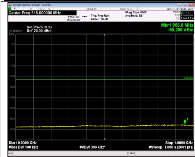
66-66-5MHz-20MHz-QPSK-QPSK-132330-132447-1RB#0-1RB#99-30~1000MHz-PASS
