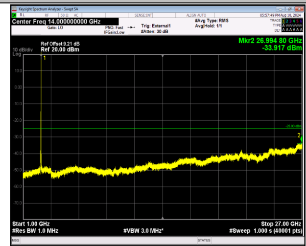
41-41-20MHz-20MHz-QPSK-QPSK-41292-41490-1RB#99- 0RB#0-1000~27000MHz-PASS
