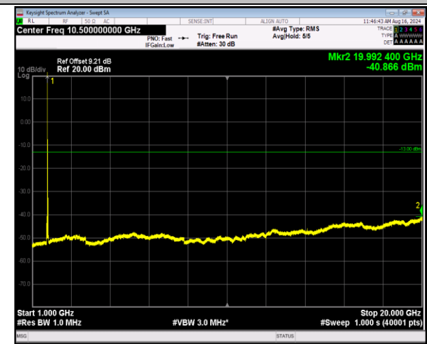
66-66-5MHz-20MHz-QPSK-QPSK-132330-132447-1RB#24-0RB#0-1000~20000MHz-PASS
