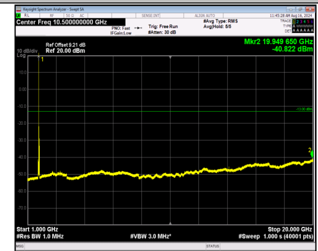
66-66-5MHz-20MHz-QPSK-QPSK-132330-132447-1RB#0-ORB#0-1000~20000MHz-PASS
