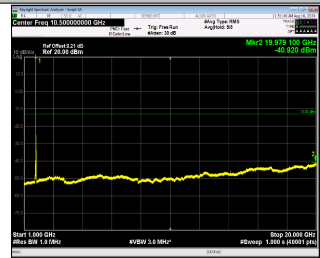
66-66-5MHz-20MHz-QPSK-QPSK-132455-132572-1RB#24 -0RB#0-1000~20000MHz-PASS
