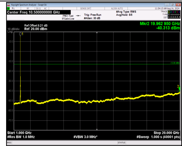
66-66-5MHz-20MHz-QPSK-QPSK-132455-132572-25RB#0 -100RB#0-1000~20000MHz-PASS
