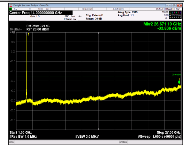
41-41-20MHz-20MHz-QPSK-QPSK-41292-41490-1RB#0-0 RB#0-1000~27000MHz-PASS
