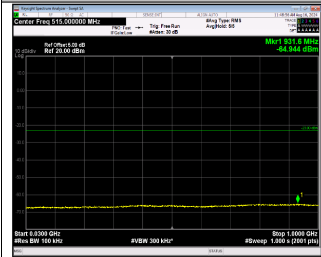
66-66-5MHz-20MHz-QPSK-QPSK-132330-132447-25RB#0-100RB#0-30~1000MHz-PASS
