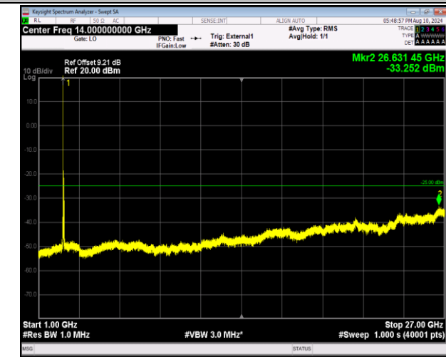
41-41-20MHz-20MHz-QPSK-QPSK-40521-40719-1RB#0-0 RB#0-1000~27000MHz-PASS
