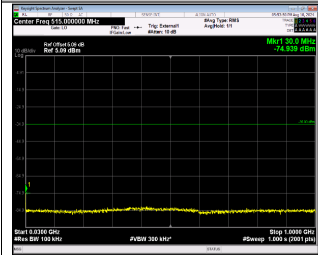
41-41-20MHz-20MHz-QPSK-QPSK-40521-40719-100RB #0-100RB#0-30~1000MHz-PASS
