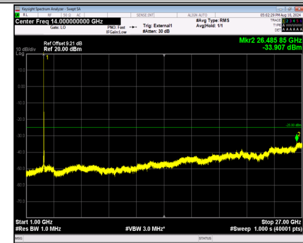
41-41-20MHz-10MHz-QPSK-QPSK-41391-41535-1RB#0-0 RB#0-1000~27000MHz-PASS
