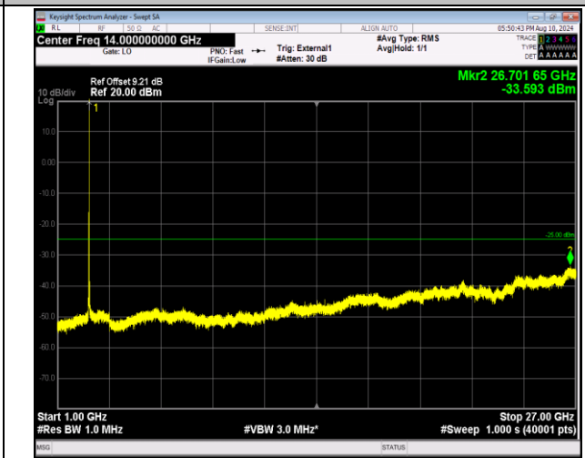
41-41-20MHz-20MHz-QPSK-QPSK-40521-40719-1RB#99- 0RB#0-1000~27000MHz-PASS
