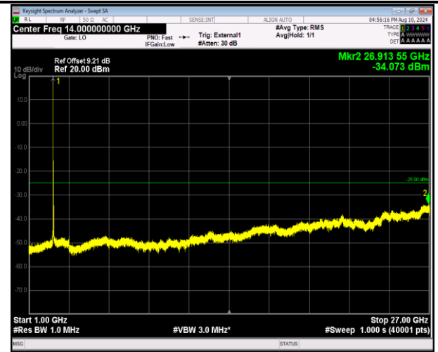
41-41-20MHz-10MHz-16QAM-16QAM-40571-40715-1RB#0 -ORB#0-1000~27000MHz-PASS
