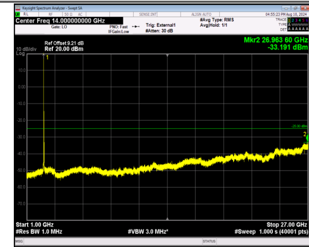
41-41-20MHz-10MHz-QPSK-QPSK-40571-40715-1RB#0-0 RB#0-1000~27000MHz-PASS
