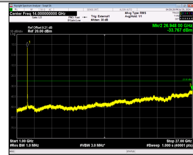
41-41-20MHz-10MHz-64QAM-64QAM-40571-40715-100RB #0-50RB#0-1000~27000MHz-PASS
