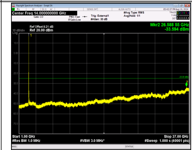
41-41-20MHz-20MHz-QPSK-QPSK-39750-39948-1RB#99- 0RB#0-1000~27000MHz-PASS
