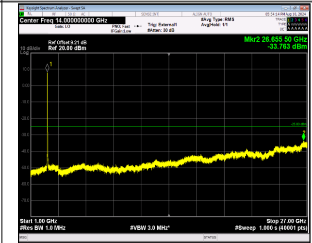
41-41-20MHz-20MHz-QPSK-QPSK-40521-40719-100RB#0 -100RB#0-1000~27000MHz-PASS
