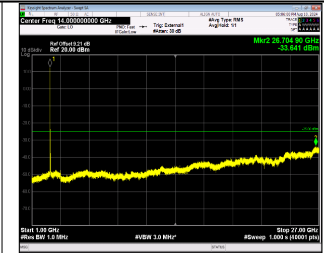
41-41-20MHz-10MHz-QPSK-QPSK-41391-41535-1RB#0-1 RB#49-1000~27000MHz-PASS
