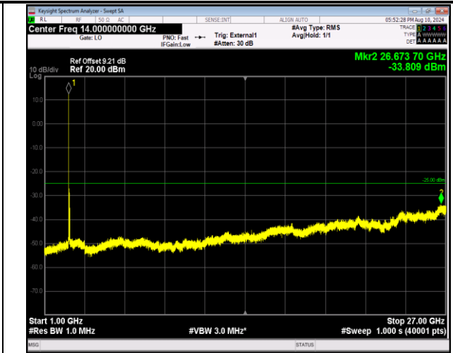
41-41-20MHz-20MHz-QPSK-QPSK-40521-40719-1RB#0-1 RB#99-1000~27000MHz-PASS
