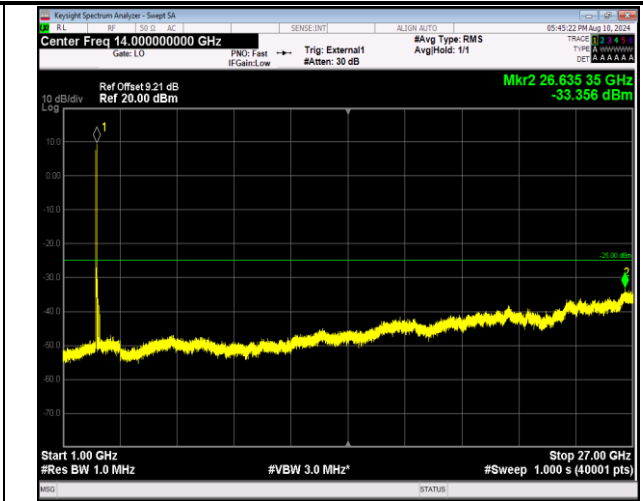
41-41-20MHz-20MHz-QPSK-QPSK-39750-39948-1RB#0-1 RB#99-1000~27000MHz-PASS
