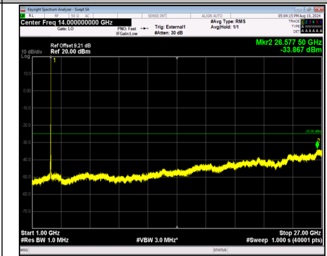
41-41-20MHz-10MHz-QPSK-QPSK-41391-41535-1RB#99- 0RB#0-1000~27000MHz-PASS
