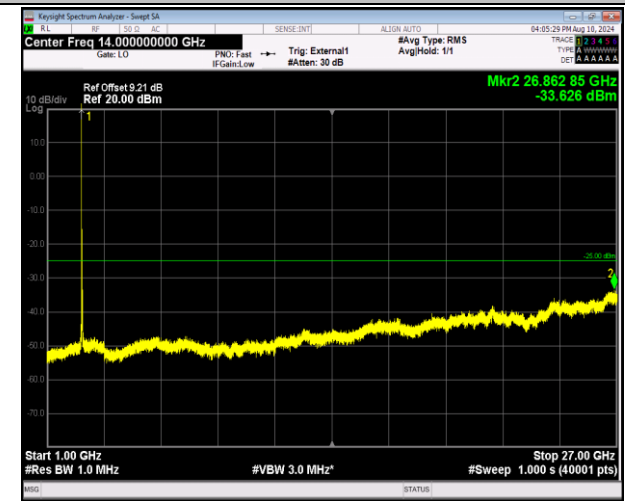
41-41-20MHz-5MHz-QPSK-QPSK-40595-40712-1RB#0-ORB#0-1000~27000MHz-PASS
