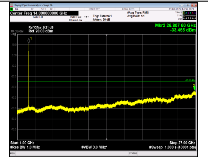
41-41-5MHz-20MHz-64QAM-64QAM-41373-41490-1RB#0- 1RB#99-1000~27000MHz-PASS
