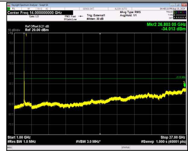
41-41-20MHz-10MHz-QPSK-QPSK-39750-39894-1RB#0-0 RB#0-1000~27000MHz-PASS
