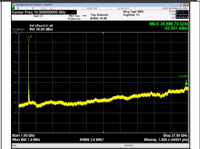
41-41-20MHz-10MHz-QPSK-QPSK-39750-39894-1RB#0-1 RB#49-1000~27000MHz-PASS
