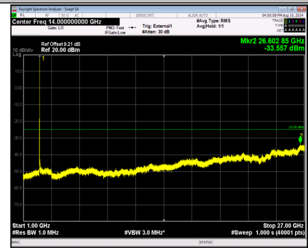
41-41-20MHz-5MHz-QPSK-QPSK-39750-39867-1RB#99-0RB#0-1000~27000MHz-PASS
