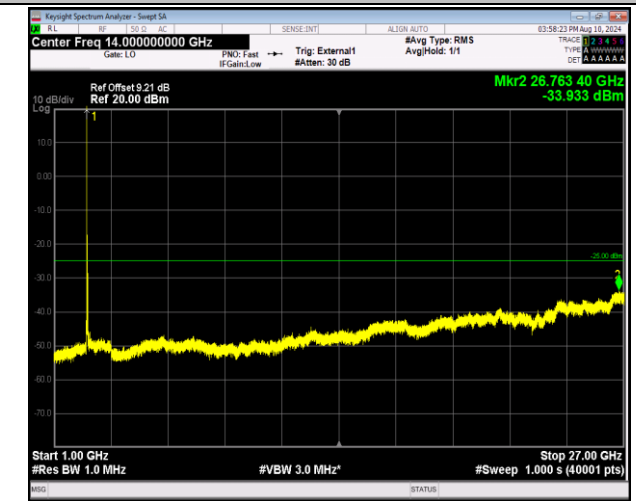
41-41-20MHz-5MHz-QPSK-QPSK-39750-39867-1RB#0-ORB#0-1000~27000MHz-PASS
