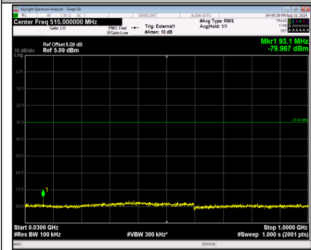
41-41-20MHz-10MHz-QPSK-QPSK-39750-39894-1RB#9 9-0RB#0-30~1000MHz-PASS
