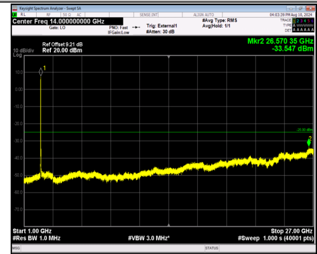
41-41-20MHz-5MHz-QPSK-QPSK-39750-39867-100RB#0-25RB#0-1000~27000MHz-PASS
