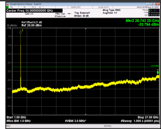
41-41-20MHz-5MHz-QPSK-QPSK-39750-39867-1RB#0-1RB#24-1000~27000MHz-PASS
