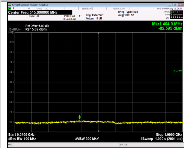
41-41-20MHz-10MHz-QPSK-QPSK-39750-39894-100RB #0-50RB#0-30~1000MHz-PASS
