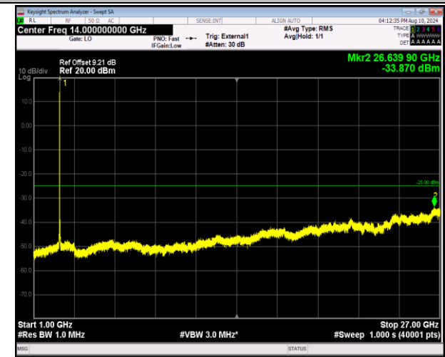
41-41-20MHz-5MHz-QPSK-QPSK-41440-41557-1RB#0-ORB#0-1000~27000MHz-PASS
