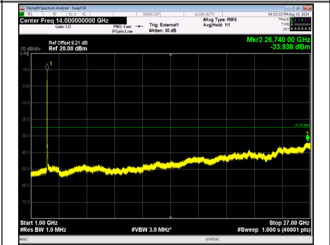
41-41-20MHz-10MHz-QPSK-QPSK-39750-39894-100RB#0 -50RB#0-1000~27000MHz-PASS
