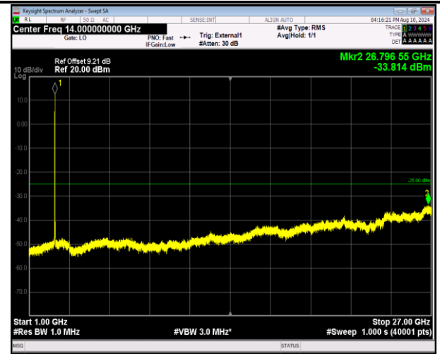
41-41-20MHz-5MHz-QPSK-QPSK-41440-41557-1RB#0-1RB#24-1000~27000MHz-PASS
