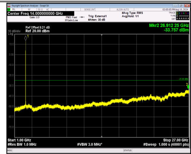
41-41-5MHz-20MHz-16QAM-16QAM-41373-41490-1RB#0- 1RB#99-1000~27000MHz-PASS
