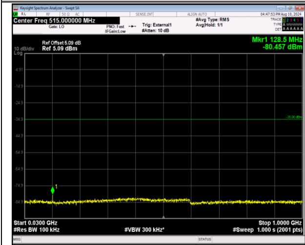
41-41-20MHz-10MHz-QPSK-QPSK-39750-39894-1RB#0 -ORB#0-30~1000MHz-PASS
