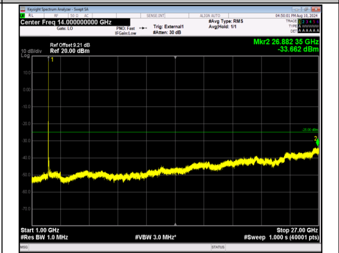
41-41-20MHz-10MHz-QPSK-QPSK-39750-39894-1RB#99- 0RB#0-1000~27000MHz-PASS
