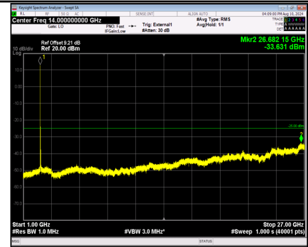
41-41-20MHz-5MHz-QPSK-QPSK-40595-40712-1RB#0-1RB#24-1000~27000MHz-PASS
