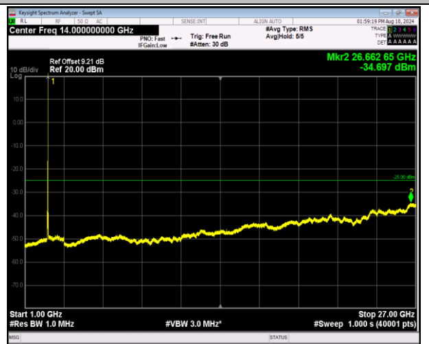
7-7-20MHz-20MHz-QPSK-QPSK-21001-21199-1RB#99-0R B#0-1000~27000MHz-PASS
