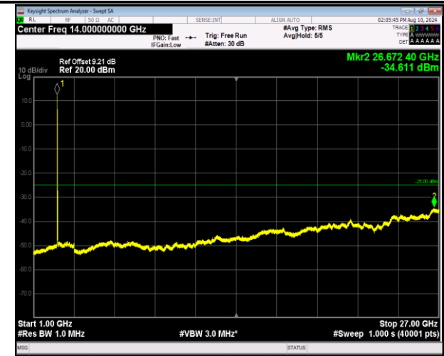
7-7-20MHz-20MHz-QPSK-QPSK-21152-21350-1RB#0-1RB #99-1000~27000MHz-PASS
