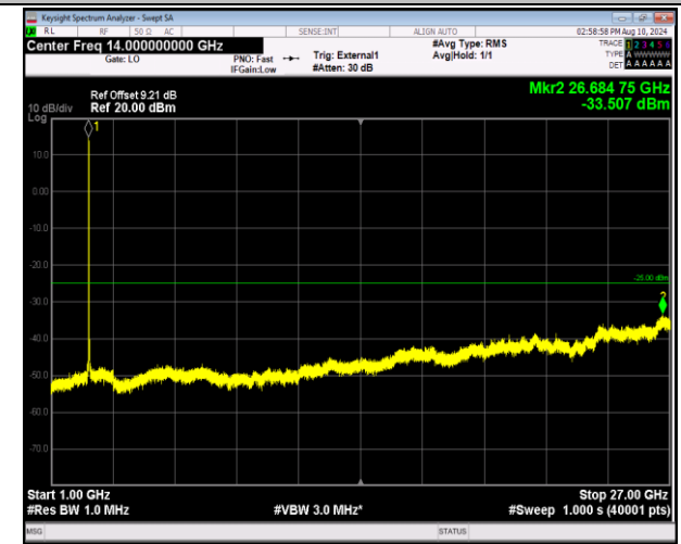
41-41-5MHz-20MHz-QPSK-QPSK-40528-40645-25RB#0-100RB#0-1000~27000MHz-PASS
