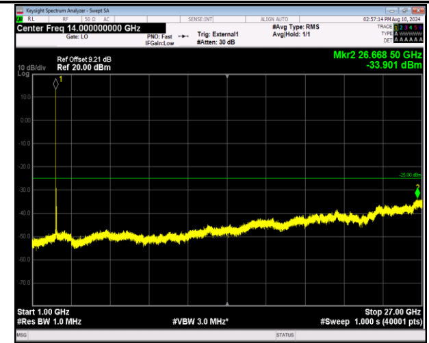
41-41-5MHz-20MHz-QPSK-QPSK-40528-40645-1RB#0-1RB#99-1000~27000MHz-PASS
