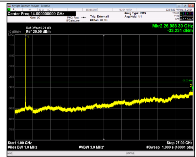
41-41-5MHz-20MHz-QPSK-QPSK-40528-40645-1RB#24-0RB#0-1000~27000MHz-PASS
