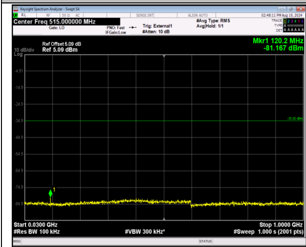
41-41-5MHz-20MHz-QPSK-QPSK-39683-39800-1RB#24-0-0RB#0-30~1000MHz-PASS
