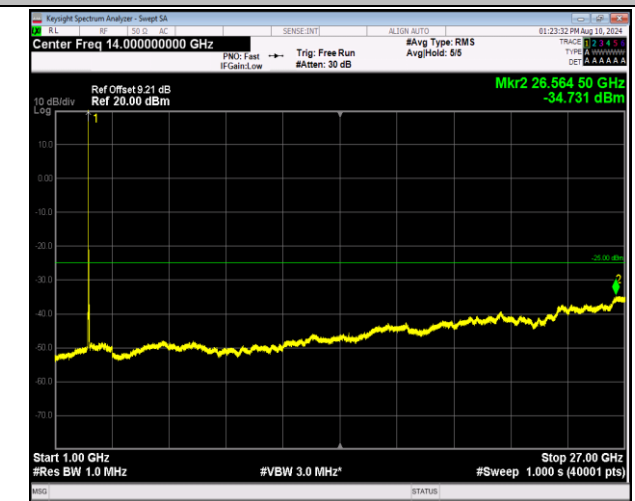
7-7-20MHz-10MHz-QPSK-QPSK-21051-21195-1RB#0-ORB #0-1000~27000MHz-PASS
