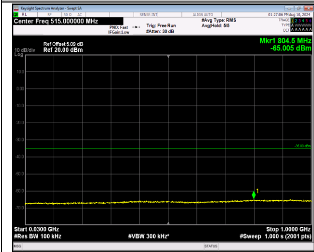
7-7-20MHz-10MHz-QPSK-QPSK-21051-21195-100RB#0- 50RB#0-30~1000MHz-PASS
