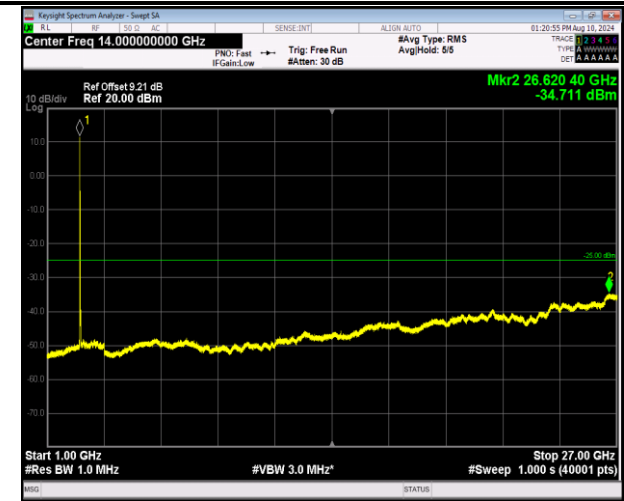
7-7-20MHz-10MHz-QPSK-QPSK-20850-20994-1RB#0-1RB #49-1000~27000MHz-PASS
