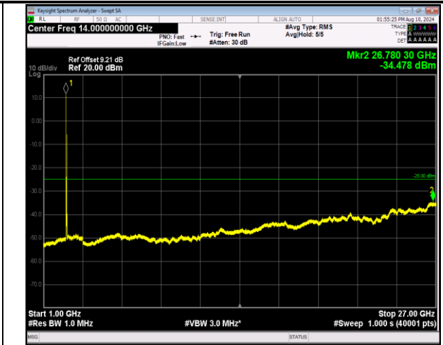
7-7-20MHz-20MHz-QPSK-QPSK-20850-21048-1RB#0-1RB #99-1000~27000MHz-PASS
