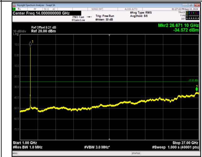
7-7-20MHz-10MHz-QPSK-QPSK-21051-21195-100RB#0-5 ORB#0-1000~27000MHz-PASS
