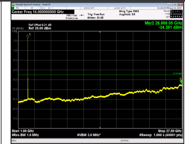
7-7-20MHz-10MHz-QPSK-QPSK-21051-21195-1RB#0-1RB #49-1000~27000MHz-PASS
