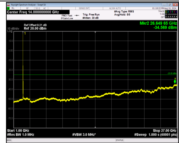
7-7-20MHz-10MHz-QPSK-QPSK-20850-20994-1RB#0-0RB #0-1000~27000MHz-PASS
