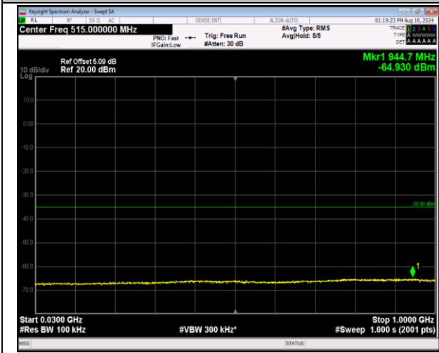
7-7-20MHz-10MHz-QPSK-QPSK-20850-20994-1RB#99-0 RB#0-30~1000MHz-PASS
