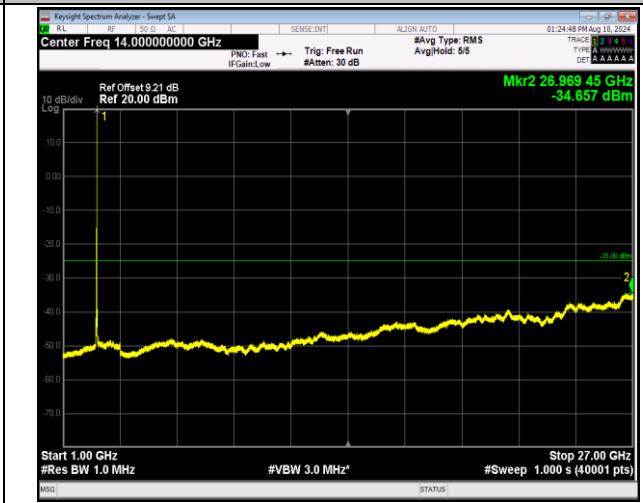
7-7-20MHz-10MHz-QPSK-QPSK-21051-21195-1RB#99-0R B#0-1000~27000MHz-PASS
