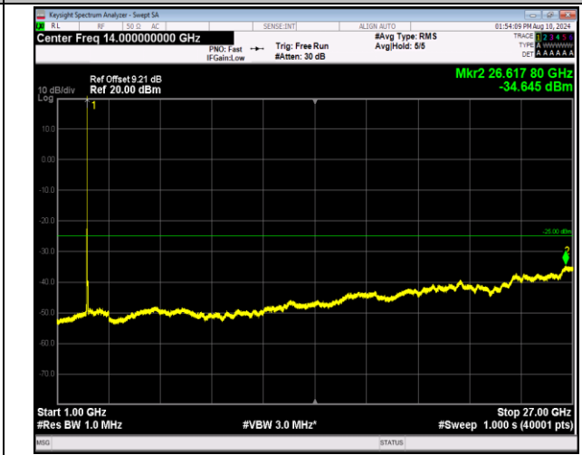
7-7-20MHz-20MHz-QPSK-QPSK-20850-21048-1RB#99-0RB#0-1000~27000MHz-PASS
