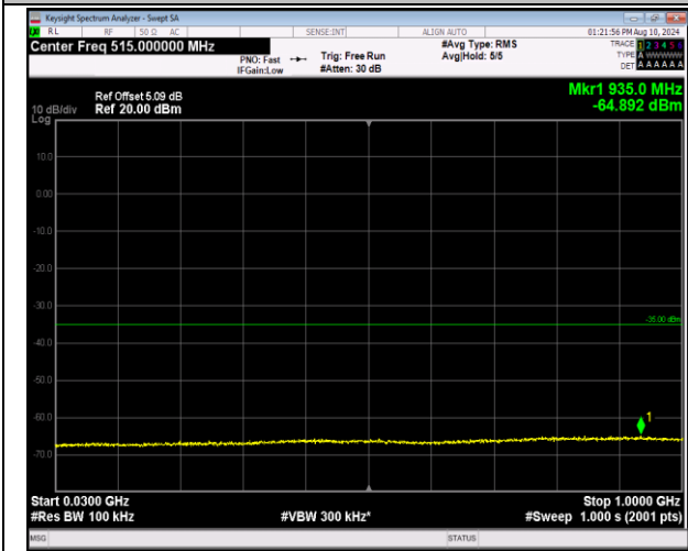
7-7-20MHz-10MHz-QPSK-QPSK-20850-20994-100RB#0 -50RB#0-30~1000MHz-PASS
