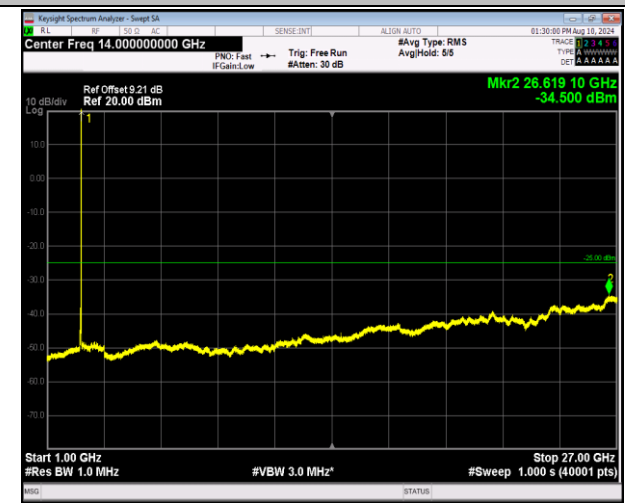
7-7-20MHz-10MHz-QPSK-QPSK-21251-21395-1RB#99-0RB#0-1000~27000MHz-PASS
