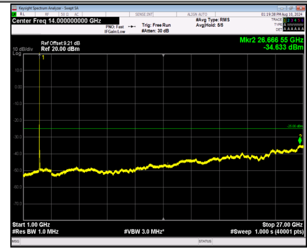
7-7-20MHz-10MHz-QPSK-QPSK-20850-20994-1RB#99-0R B#0-1000~27000MHz-PASS
