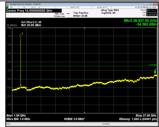
7-7-20MHz-10MHz-QPSK-QPSK-21251-21395-100RB#0-50RB#0-1000~27000MHz-PASS
