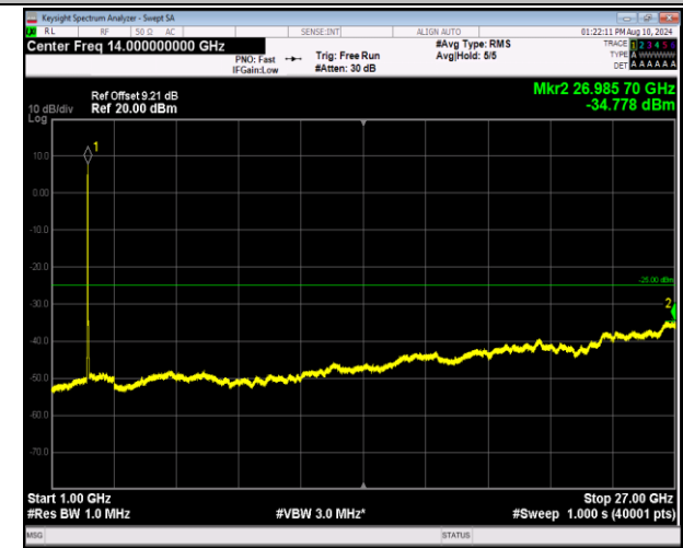
7-7-20MHz-10MHz-QPSK-QPSK-20850-20994-100RB#0-5 ORB#0-1000~27000MHz-PASS
