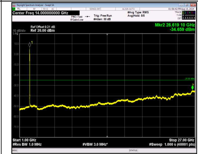
7-7-20MHz-20MHz-QPSK-QPSK-20850-21048-100RB#0-100RB#0-1000~27000MHz-PASS
