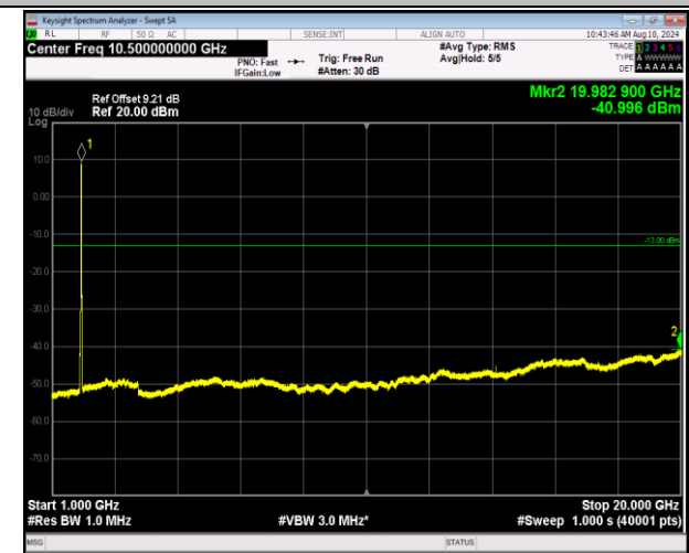
2-2-20MHz-20MHz-QPSK-QPSK-18902-19100-100RB#0-1 00RB#0-1000~20000MHz-PASS
