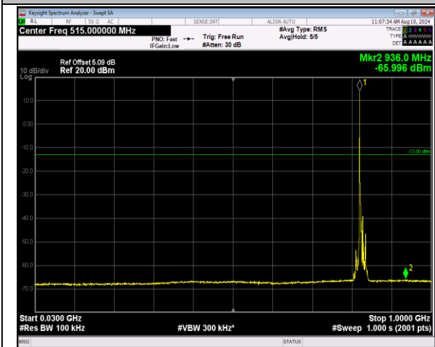
5-5-3MHz-5MHz-QPSK-QPSK-20416-20455-1RB#0-0RB #0-30~1000MHz-PASS
