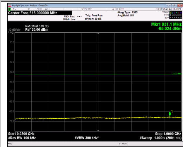
2-2-20MHz-20MHz-QPSK-QPSK-18902-19100-1RB#99-0R 0RB#0-30~1000MHz-PASS
