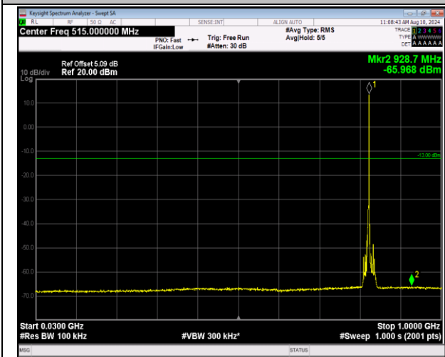
5-5-3MHz-5MHz-QPSK-QPSK-20416-20455-1RB#14-0R B#0-30~1000MHz-PASS
