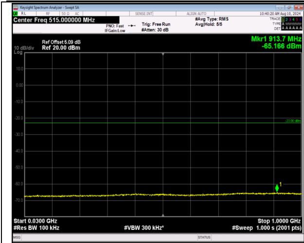
2-2-20MHz-20MHz-16QAM-16QAM-18902-19100-1RB#0 -ORB#0-30~1000MHz-PASS
