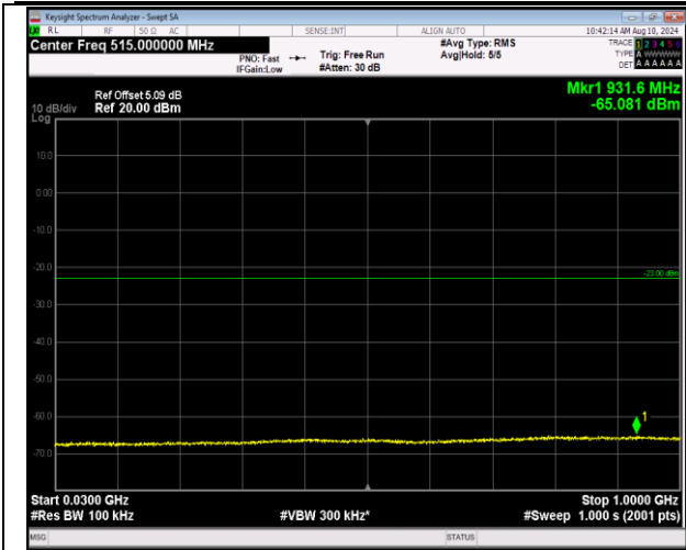
2-2-20MHz-20MHz-QPSK-QPSK-18902-19100-1RB#0-1 RB#99-30~1000MHz-PASS
