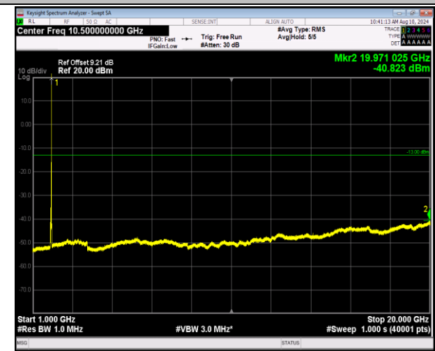
2-2-20MHz-20MHz-QPSK-QPSK-18902-19100-1RB#99-0R B#0-1000~20000MHz-PASS
