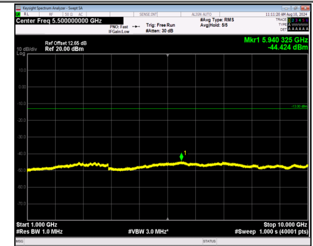
5-5-3MHz-5MHz-QPSK-QPSK-20416-20455-15RB#0-25RB #0-1000~10000MHz-PASS
