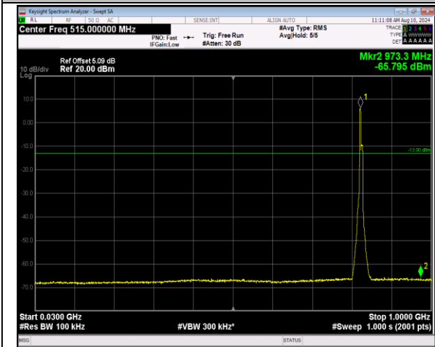
5-5-3MHz-5MHz-QPSK-QPSK-20416-20455-15RB#0-25 RB#0-30~1000MHz-PASS
