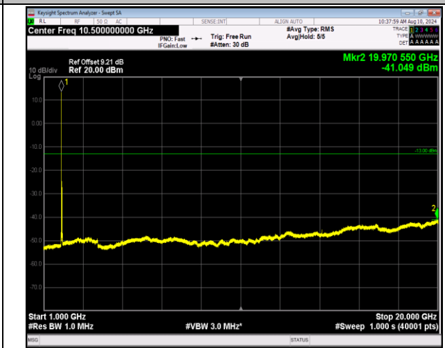
2-2-20MHz-20MHz-16QAM-16QAM-18801-18999-1RB#0-1RB#99-1000~20000MHz-PASS
