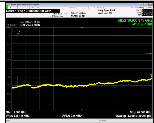
2-2-20MHz-20MHz-QPSK-QPSK-18801-18999-100RB#0-100RB#0-1000~20000MHz-PASS
