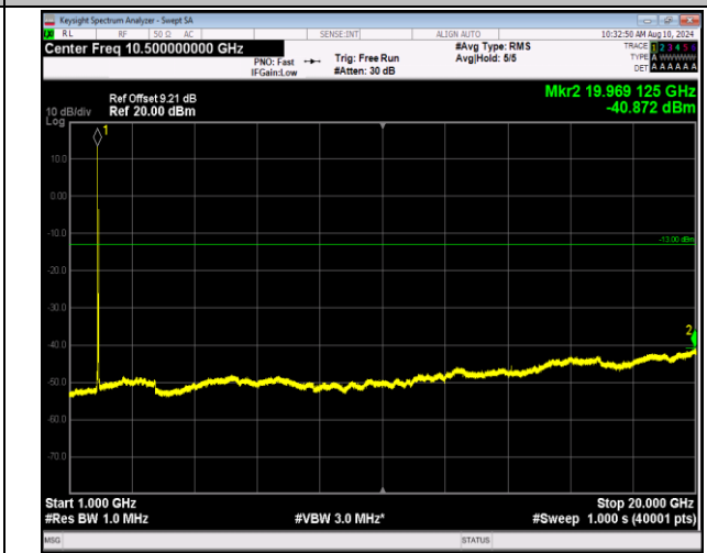
2-2-20MHz-20MHz-16QAM-16QAM-18700-18898-1RB#0-1 RB#99-1000~20000MHz-PASS
