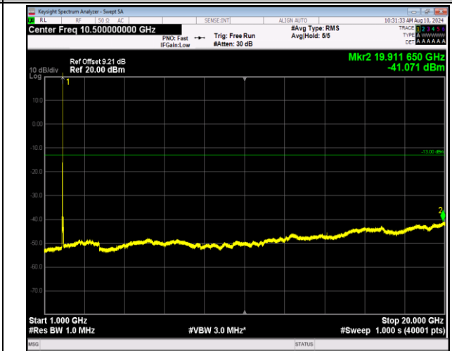
2-2-20MHz-20MHz-16QAM-16QAM-18700-18898-1RB#99- ORB#0-1000~20000MHz-PASS
