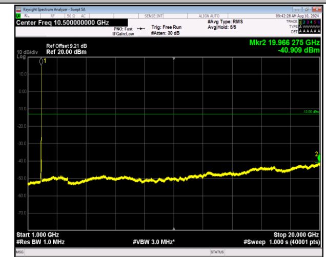
2-2-5MHz-20MHz-QPSK-QPSK-18808-18925-25RB#0-100 RB#0-1000~20000MHz-PASS
