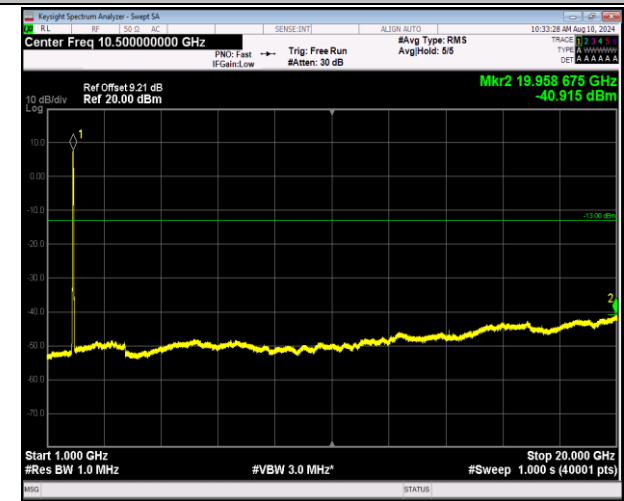
2-2-20MHz-20MHz-QPSK-QPSK-18700-18898-100RB#0-1 00RB#0-1000~20000MHz-PASS
