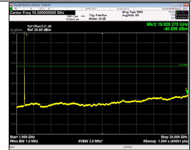
2-2-20MHz-20MHz-QPSK-QPSK-18801-18999-1RB#0-ORB #0-1000~20000MHz-PASS
