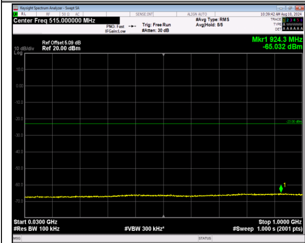
2-2-20MHz-20MHz-QPSK-QPSK-18902-19100-1RB#0-0 RB#0-30~1000MHz-PASS
