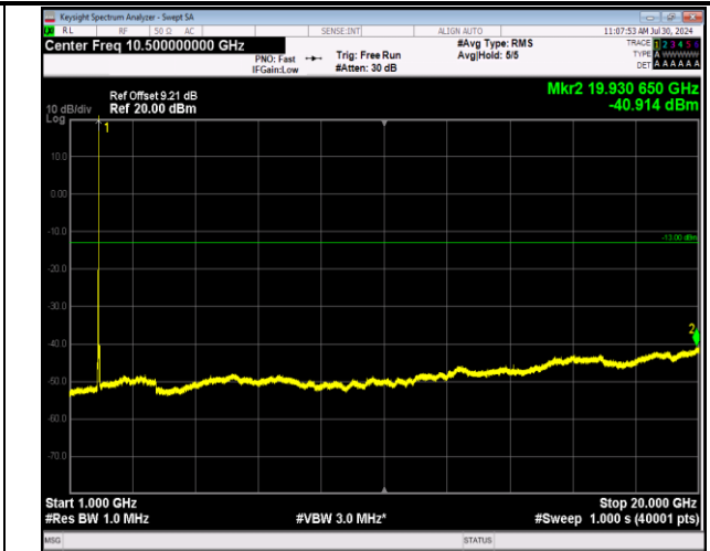
2-2-20MHz-20MHz-64QAM-64QAM-18801-18999-1RB#99- ORB#0-1000~20000MHz-PASS
