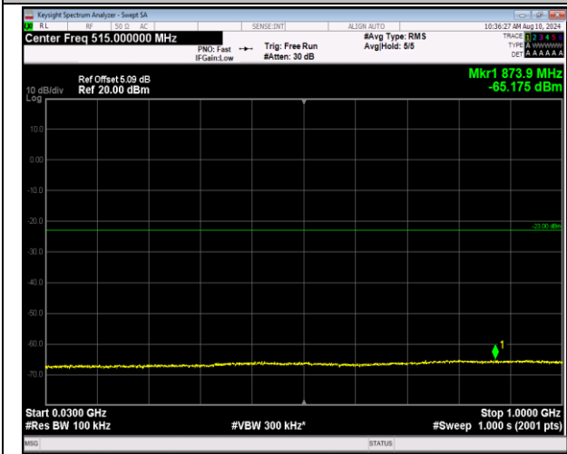
2-2-20MHz-20MHz-16QAM-16QAM-18801-18999-1RB#99-9-ORB#0-30~1000MHz-PASS
