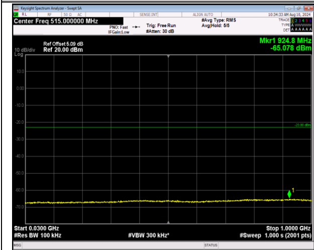
2-2-20MHz-20MHz-QPSK-QPSK-18801-18999-1RB#0-0 RB#0-30~1000MHz-PASS
