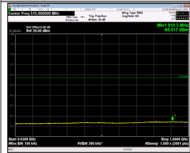
2-2-20MHz-20MHz-QPSK-QPSK-18700-18898-1RB#99-0R B#0-30~1000MHz-PASS
