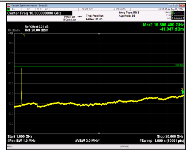
2-2-20MHz-20MHz-QPSK-QPSK-18700-18898-1RB#99-0R B#0-1000~20000MHz-PASS
