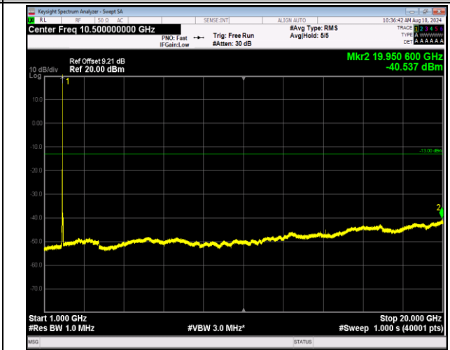
2-2-20MHz-20MHz-16QAM-16QAM-18801-18999-1RB#99-ORB#0-1000~20000MHz-PASS
