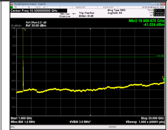
2-2-20MHz-20MHz-16QAM-16QAM-18801-18999-1RB#0-0 RB#0-1000~20000MHz-PASS
