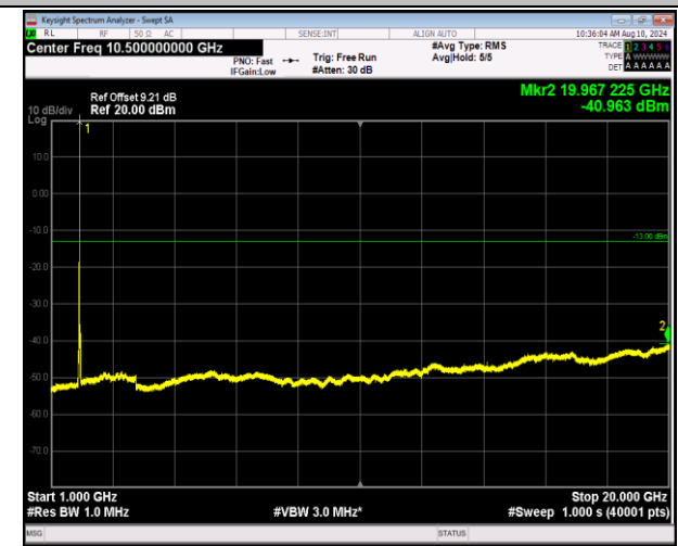
2-2-20MHz-20MHz-QPSK-QPSK-18801-18999-1RB#99-0RB#0-1000~20000MHz-PASS
