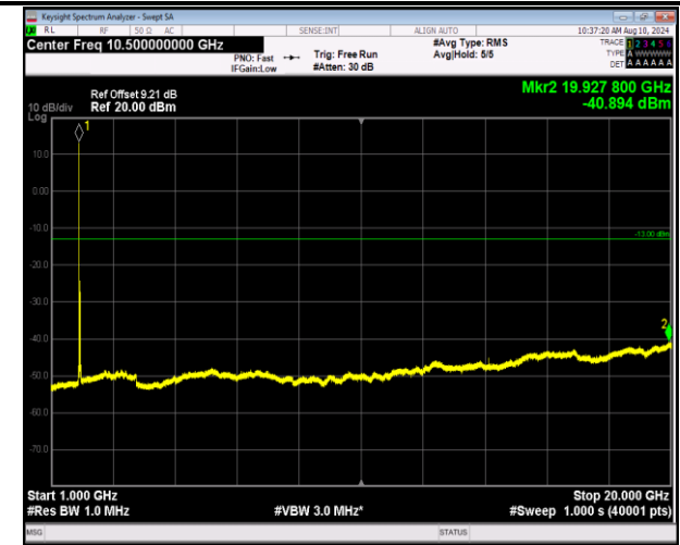
2-2-20MHz-20MHz-QPSK-QPSK-18801-18999-1RB#0-1RB #99-1000~20000MHz-PASS
