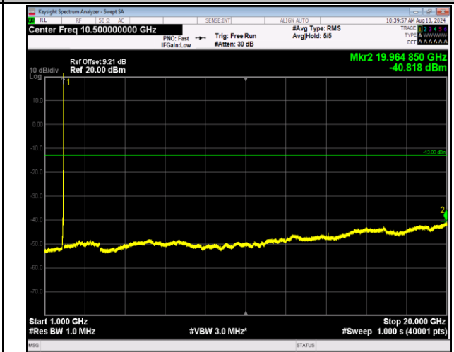
2-2-20MHz-20MHz-QPSK-QPSK-18902-19100-1RB#0-ORB #0-1000~20000MHz-PASS
