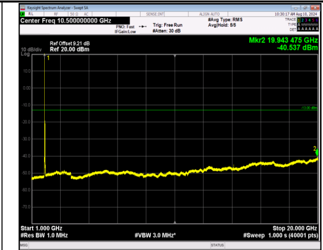
2-2-20MHz-20MHz-16QAM-16QAM-18700-18898-1RB#0-0 RB#0-1000~20000MHz-PASS
