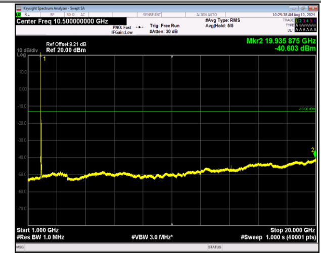
2-2-20MHz-20MHz-QPSK-QPSK-18700-18898-1RB#0-0RB #0-1000~20000MHz-PASS
