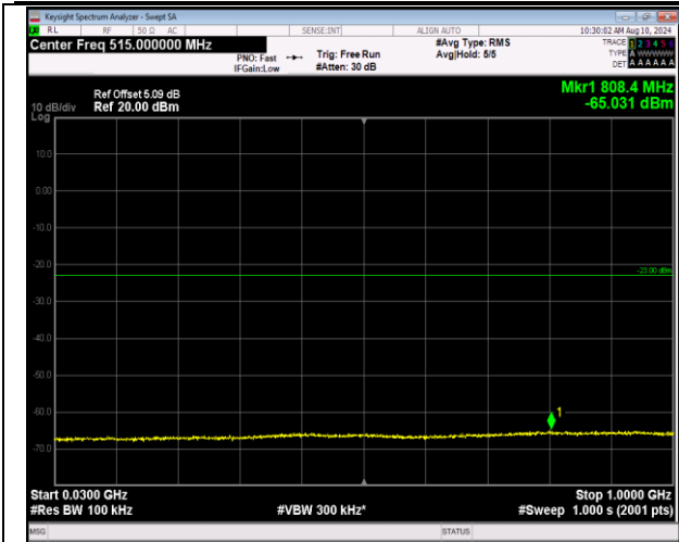
2-2-20MHz-20MHz-16QAM-16QAM-18700-18898-1RB#0 -ORB#0-30~1000MHz-PASS
