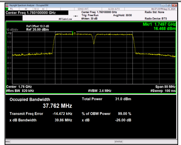
66-66-20MHz-20MHz-QPSK-QPSK-132374-132572-100R B#0-100RB#0-PASS
