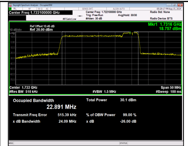
66-66-20MHz-5MHz-16QAM-16QAM-132072-132189-100 RB#0-25RB#0-PASS
