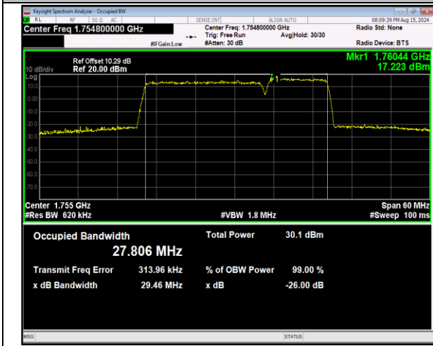
66-66-20MHz-10MHz-64QAM-64QAM-132373-132517-10 ORB#0-50RB#0-PASS
