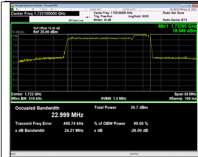
66-66-20MHz-5MHz-QPSK-QPSK-132072-132189-100RB #0-25RB#0-PASS
