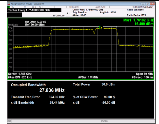
66-66-20MHz-10MHz-16QAM-16QAM-132373-132517-10 ORB#0-50RB#0-PASS
