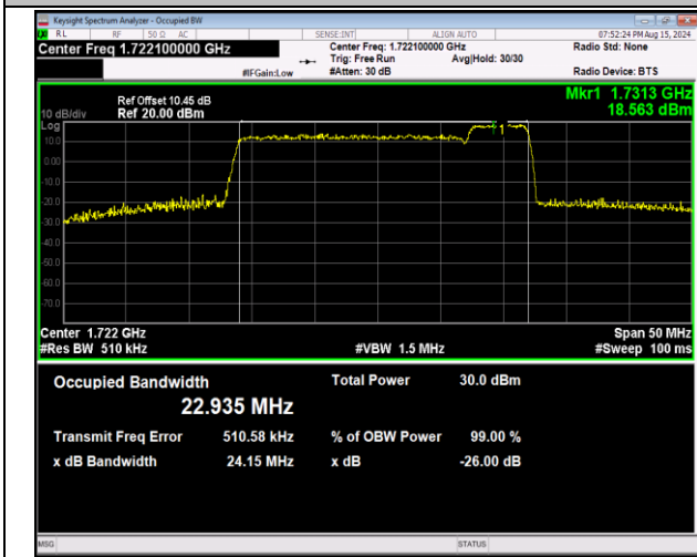
66-66-20MHz-5MHz-64QAM-64QAM-132072-132189-100 RB#0-25RB#0-PASS
