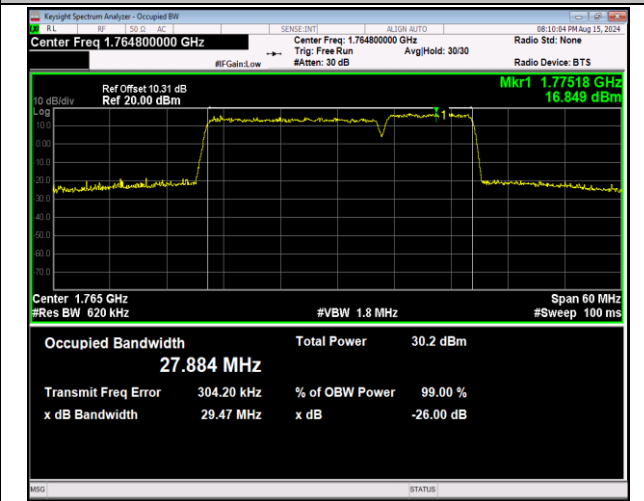
66-66-20MHz-10MHz-64QAM-64QAM-132473-132617-10 ORB#0-50RB#0-PASS
