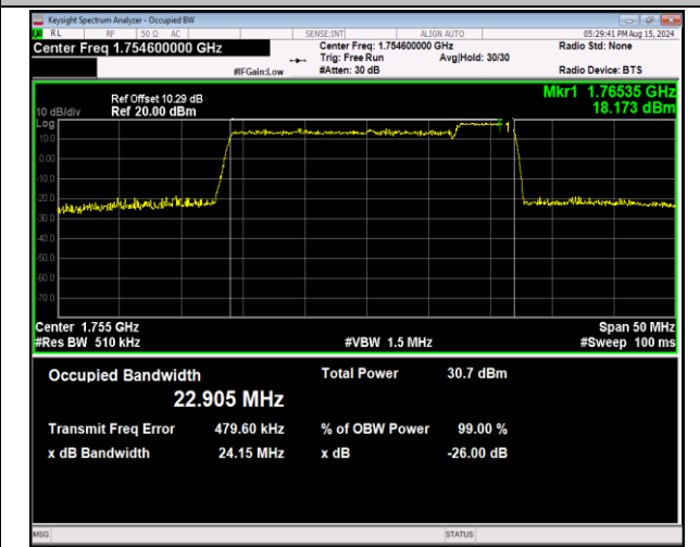
66-66-20MHz-5MHz-QPSK-QPSK-132397-132514-100RB #0-25RB#0-PASS
