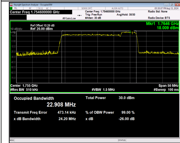
66-66-20MHz-5MHz-16QAM-16QAM-132397-132514-100 RB#0-25RB#0-PASS
