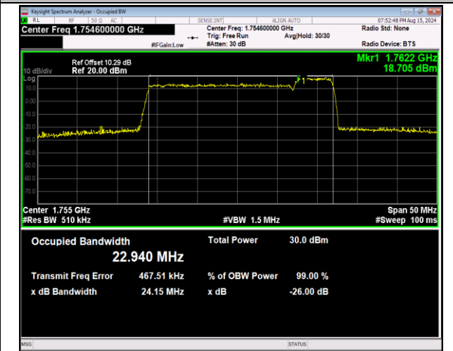
66-66-20MHz-5MHz-64QAM-64QAM-132397-132514-100 RB#0-25RB#0-PASS
