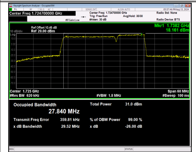
66-66-20MHz-10MHz-QPSK-QPSK-132072-132216-100RB#0-50RB#0-PASS
