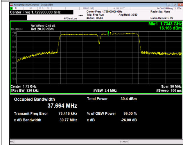
66-66-20MHz-20MHz-16QAM-16QAM-132072-132270-10 ORB#0-100RB#0-PASS
