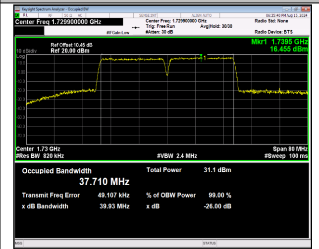
66-66-20MHz-20MHz-QPSK-QPSK-132072-132270-100R B#0-100RB#0-PASS
