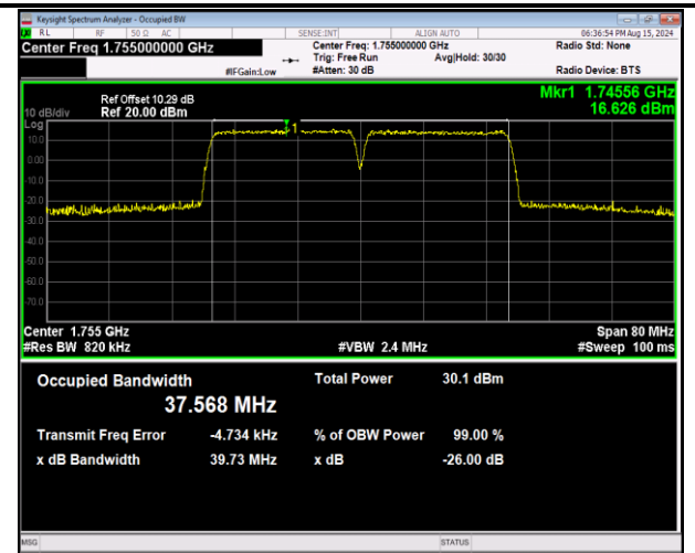
66-66-20MHz-20MHz-16QAM-16QAM-132323-132521-10 ORB#0-100RB#0-PASS
