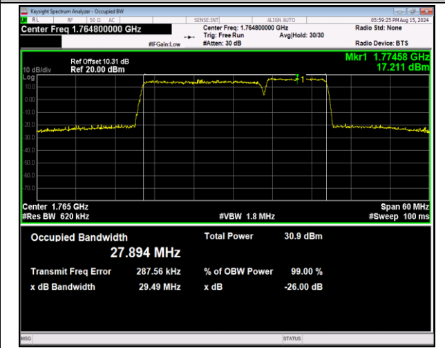
66-66-20MHz-10MHz-QPSK-QPSK-132473-132617-100R B#0-50RB#0-PASS
