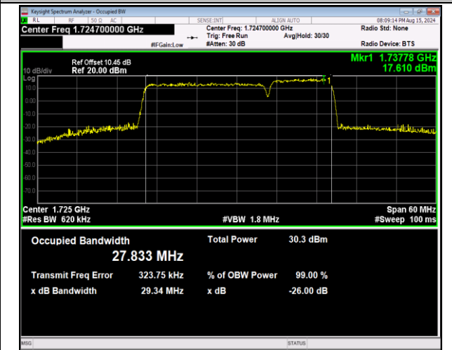
66-66-20MHz-10MHz-64QAM-64QAM-132072-132216-10ORB#0-50RB#0-PASS
