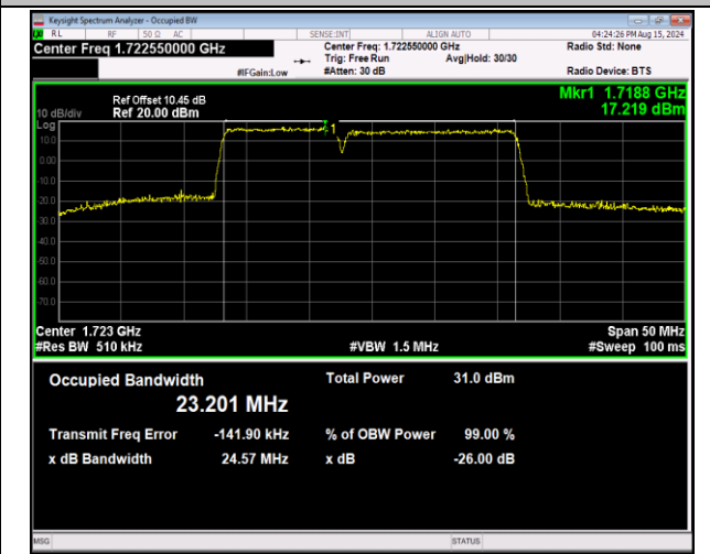
66-66-10MHz-15MHz-QPSK-QPSK-132025-132145-50RB#0-75RB#0-PASS
