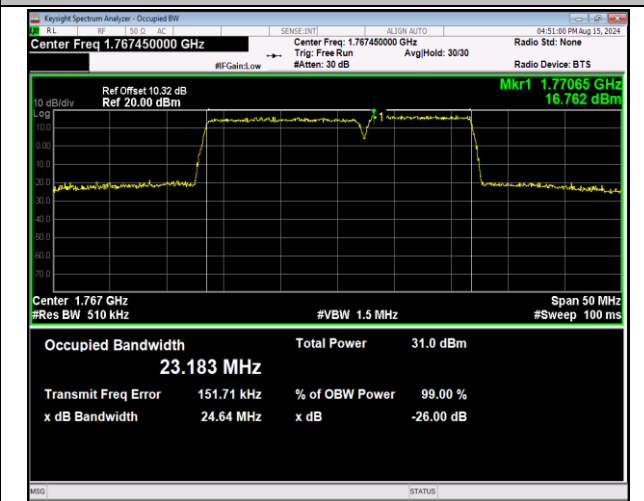
66-66-15MHz-10MHz-QPSK-QPSK-132499-132619-75RB #0-50RB#0-PASS
