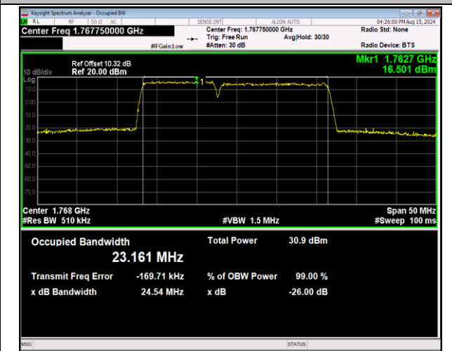
66-66-10MHz-15MHz-QPSK-QPSK-132477-132597-50RB #0-75RB#0-PASS
