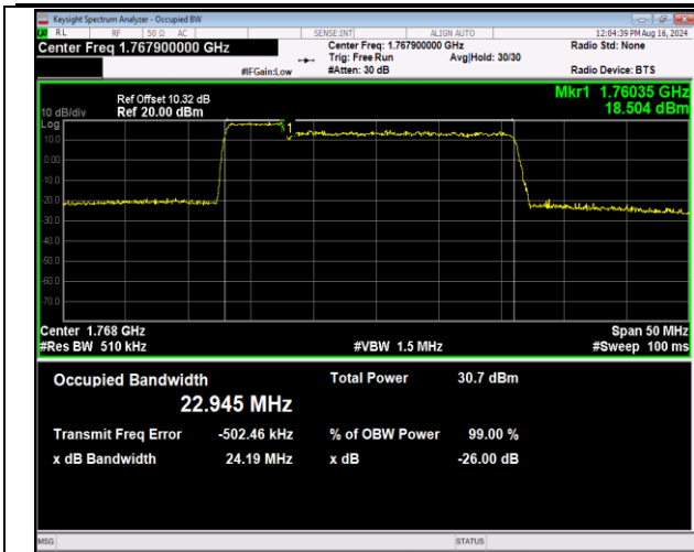
66-66-5MHz-20MHz-QPSK-QPSK-132455-132572-25RB#0-100RB#0-PASS
