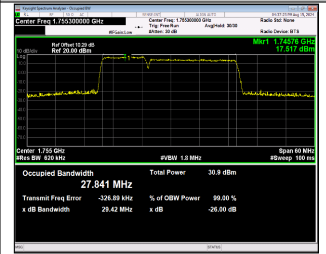
66-66-10MHz-20MHz-QPSK-QPSK-132328-132472-50RB #0-100RB#0-PASS
