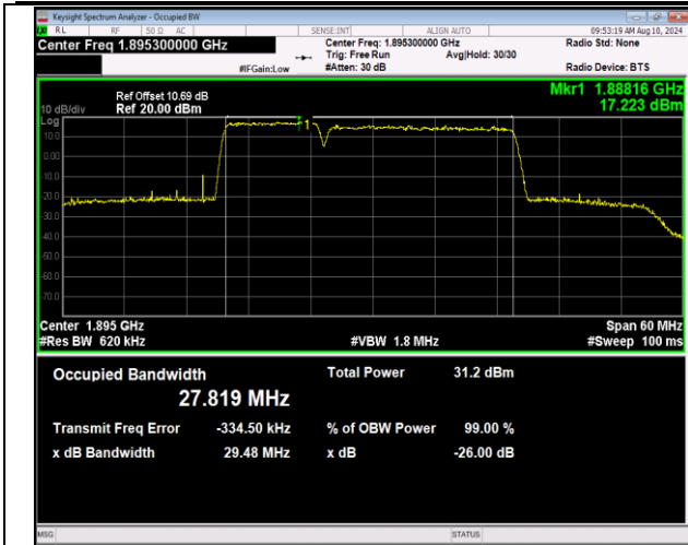
2-2-10MHz-20MHz-QPSK-QPSK-18956-19100-50RB#0-1 00RB#0-PASS
