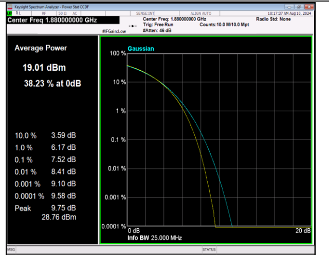
2-2-20MHz-20MHz-16QAM-16QAM-18801-18999-100RB#0-0-100RB#0-PASS
