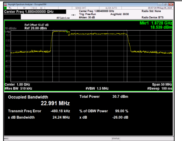
2-2-5MHz-20MHz-QPSK-QPSK-18808-18925-25RB#0-10 ORB#0-PASS
