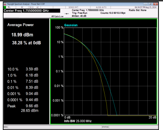
66-66-20MHz-20MHz-16QAM-16QAM-132323-132521-10 ORB#0-100RB#0-PASS
