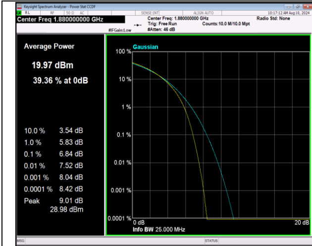
2-2-20MHz-20MHz-QPSK-QPSK-18801-18999-100RB#0-100RB#0-PASS
