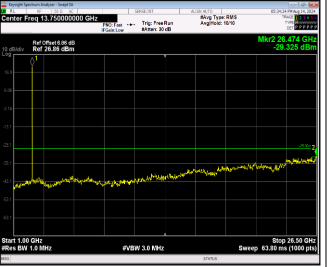
Band41-20MHz-QPSK-41490-1RB#0-Range2:1000~26500MHz
