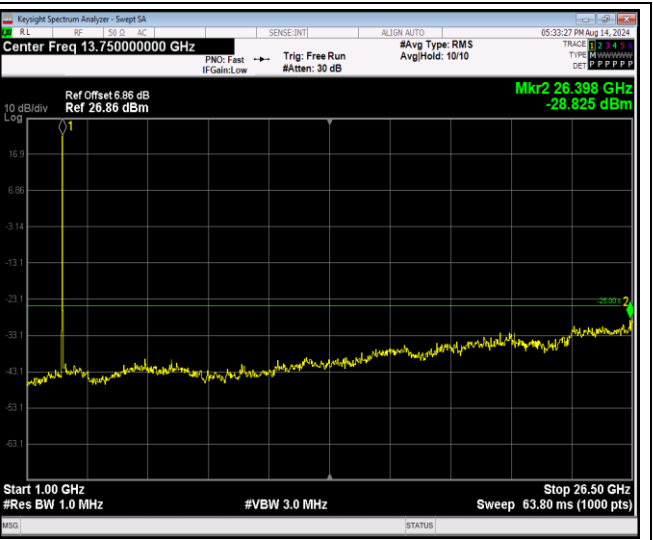
Band41-20MHz-QPSK-40620-1RB#0-Range2:1000~26500MHz
