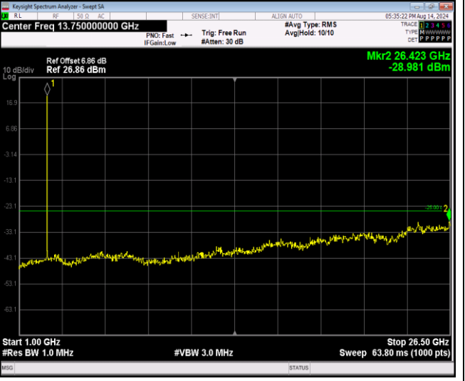
Band41-20MHz-QPSK-41490-1RB#0-Range2:1000~26500MHz
