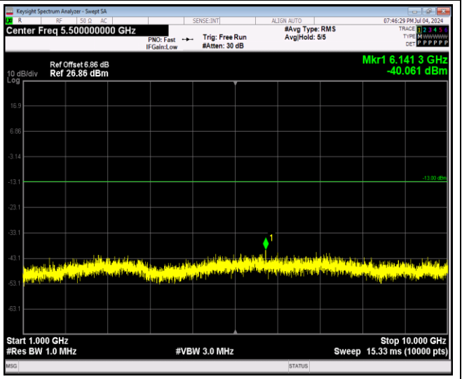
Band13-5MHz-QPSK-23230-1RB#0-Range4:1000~10000MHz
