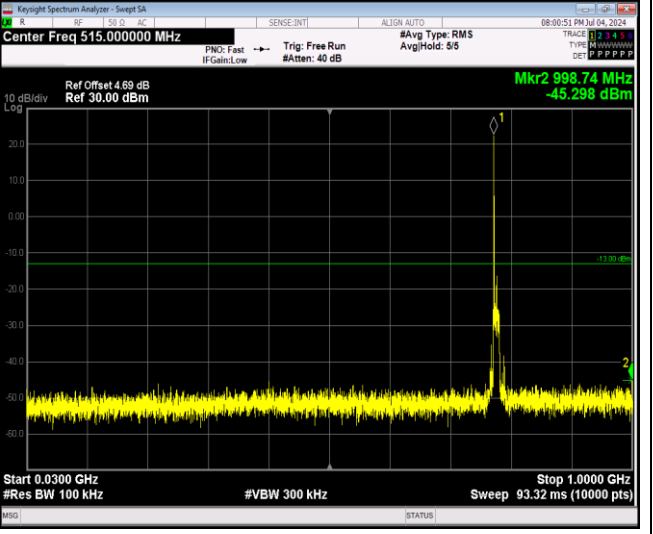
Band13-10MHz-QPSK-23230-1RB#0-Range3:30~10 00MHz
