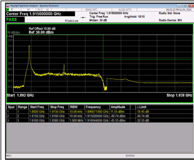
Band25-20MHz-QPSK-26590-100RB#0
