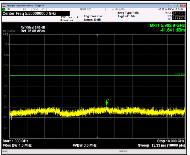
Band13-5MHz-QPSK-23255-1RB#0-Range2:1000~10000MHz
