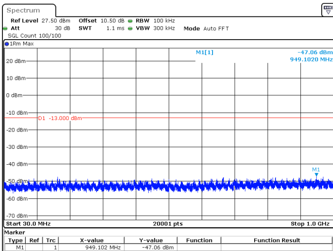
40MHz_30kHz_3530MHz_DFT-s-OFDM QPSK_RB100@0 -47.06 dBm
