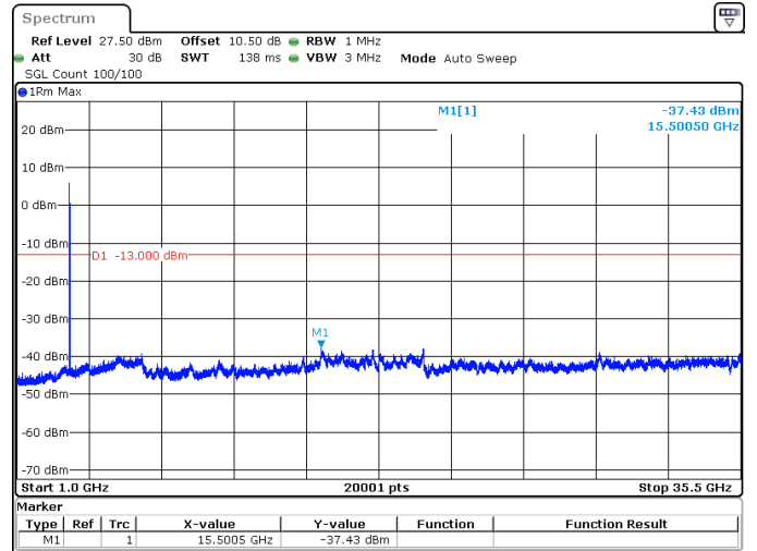
40MHz_30kHz_3530MHz_DFT-s-OFDM QPSK_RB1@0 -37.43 dBm
