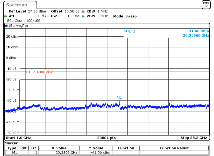
20MHz_15kHz_3500MHz_DFT-s-OFDM QPSK_RB1@105 -41.06 dBm
