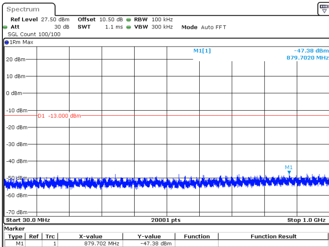
10MHz_15kHz_3455MHz_DFT-s-OFDM QPSK_RB50@0 -47.38 dBm
