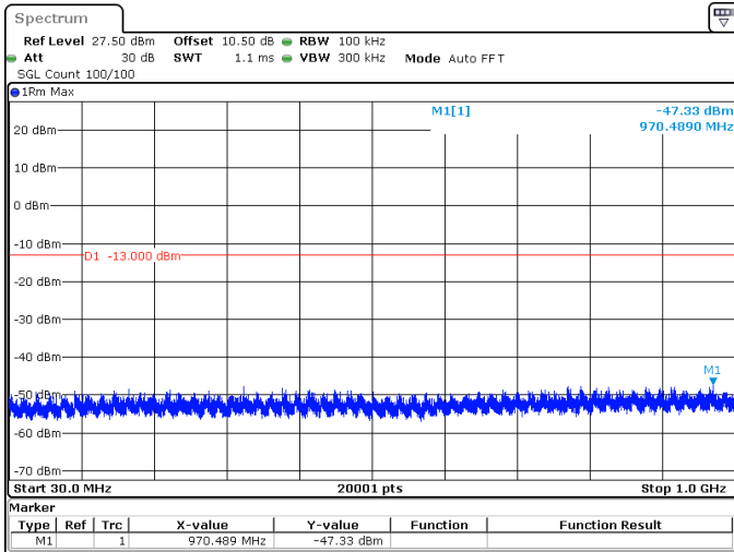
40MHz_30kHz_3530MHz_DFT-s-OFDM QPSK_RB1@0 -47.33 dBm
