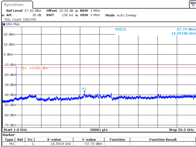
10MHz_15kHz_3455MHz_DFT-s-OFDM QPSK_RB1@51 -37.73 dBm
