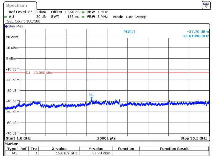
40MHz_30kHz_3530MHz_DFT-s-OFDM QPSK_RB1@105 -37.70 dBm
