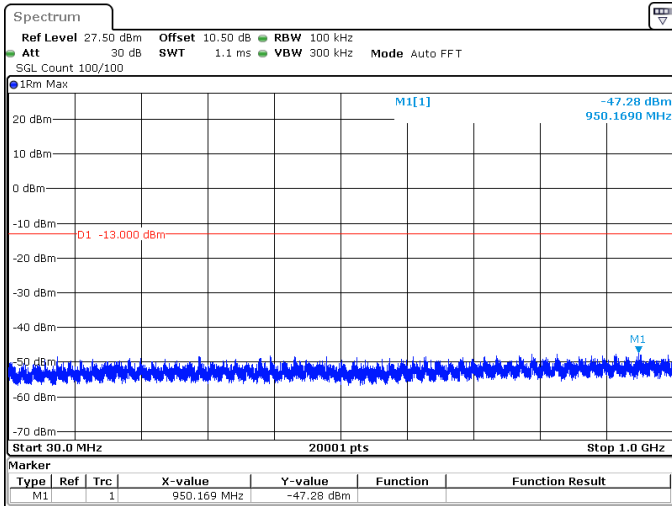
10MHz_15kHz_3455MHz_DFT-s-OFDM QPSK_RB1@0 -47.28 dBm
