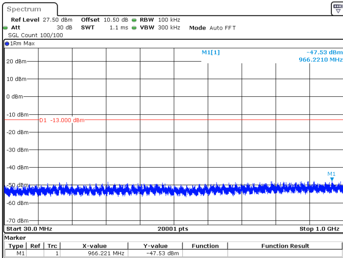
40MHz_30kHz_3530MHz_DFT-s-OFDM QPSK_RB1@105 -47.53 dBm
