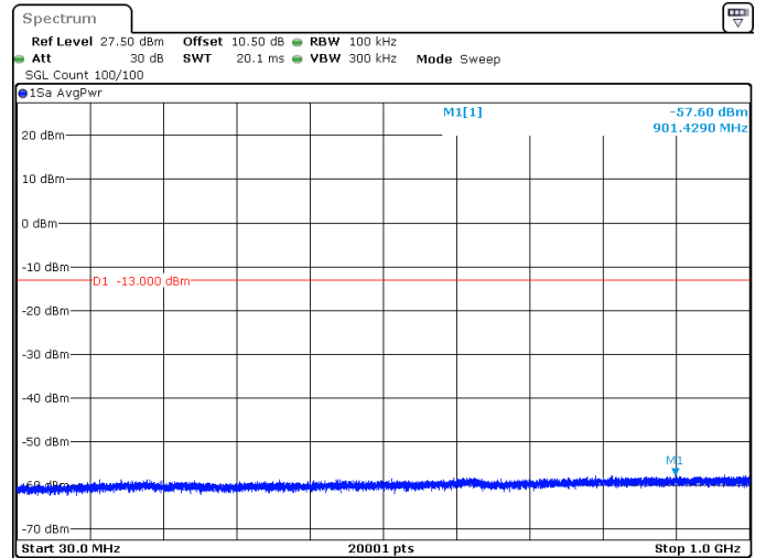
20MHz_15kHz_3500MHz_DFT-s-OFDM QPSK_RB1@0 -57.60 dBm
