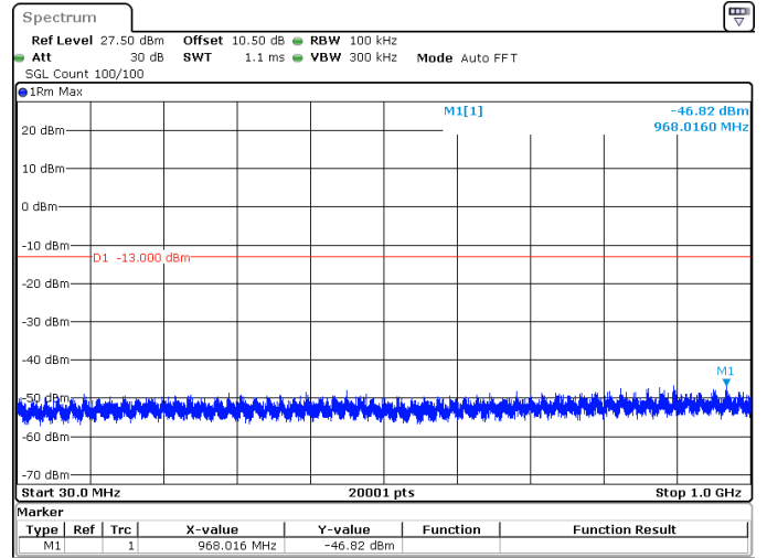
10MHz_15kHz_3455MHz_DFT-s-OFDM QPSK_RB1@51 -46.82 dBm
