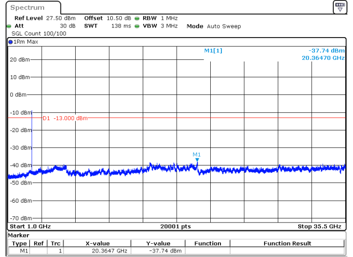
10MHz_15kHz_3455MHz_DFT-s-OFDM QPSK_RB1@0 -37.74 dBm
