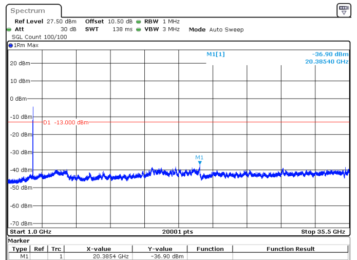
40MHz_30kHz_3530MHz_DFT-s-OFDM QPSK_RB100@0 -36.90 dBm
