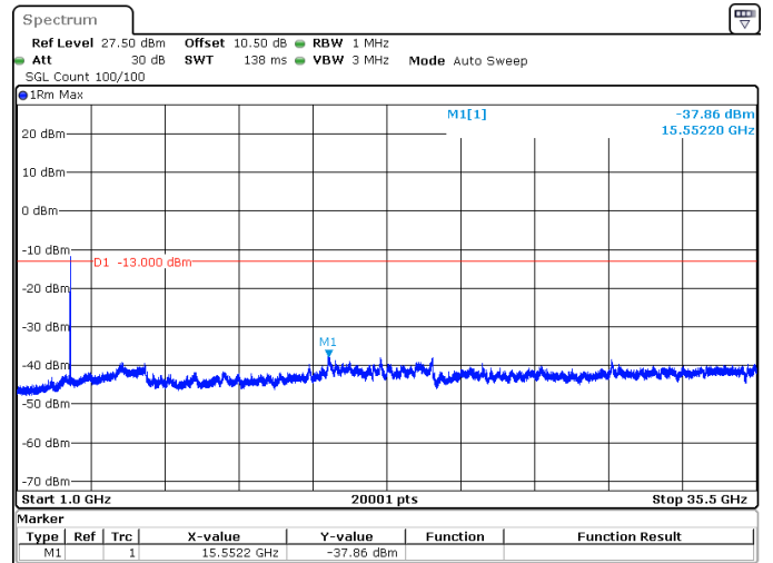
20MHz_30kHz_3460MHz_DFT-s-OFDM QPSK_RB1@50 -37.86 dBm
