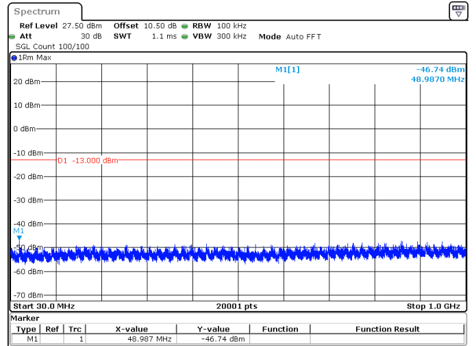
20MHz_30kHz_3460MHz_DFT-s-OFDM QPSK_RB1@0 -46.74 dBm
