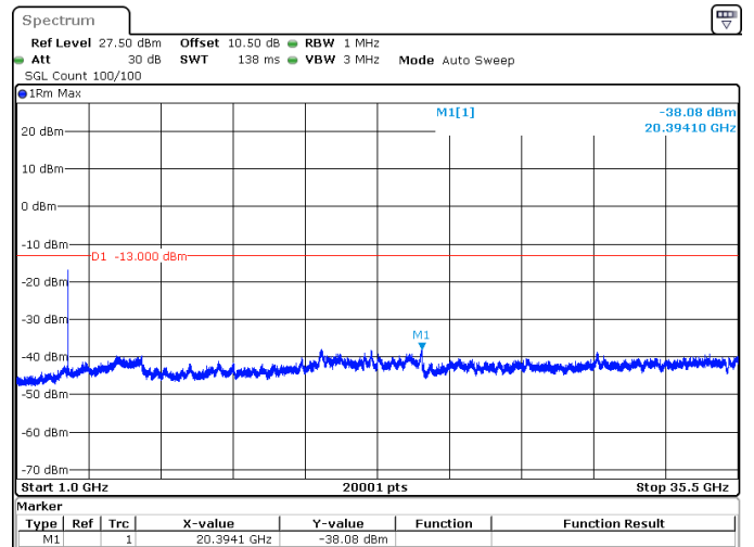
10MHz_15kHz_3455MHz_DFT-s-OFDM QPSK_RB50@0 -38.08 dBm
