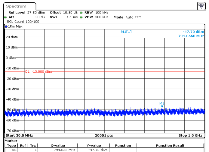
20MHz_30kHz_3460MHz_DFT-s-OFDM QPSK_RB50@0 -47.70 dBm
