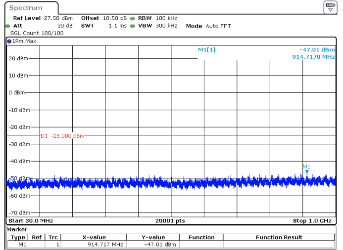
90MHz_30kHz_2644.98MHz_DFT-s-OFDM QPSK_RB1@244 -47.01 dBm
