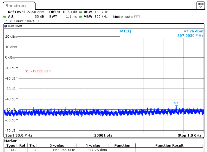
5MHz_15kHz_1712.5MHz_DFT-s-OFDM QPSK_RB25@0 -47.76 dBm
