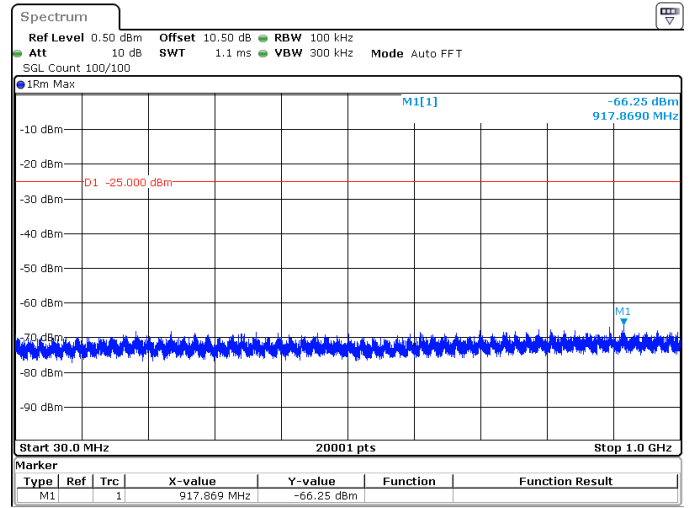
5MHz_15kHz_2502.5MHz_DFT-s-OFDM QPSK_RB1@0 -66.25 dBm
