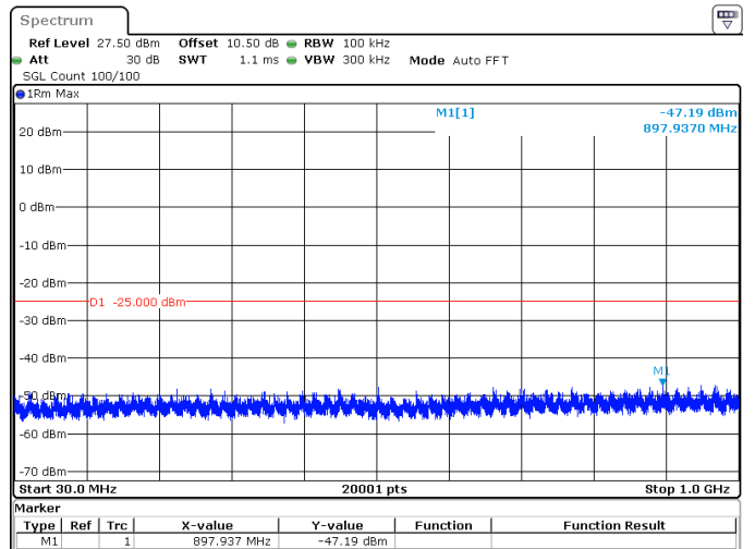
90MHz_30kHz_2644.98MHz_DFT-s-OFDM QPSK_RB243@0 -47.19 dBm
