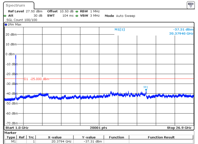
80MHz_30kHz_2536.02MHz_DFT-s-OFDM QPSK_RB216@0 -37.31 dBm
