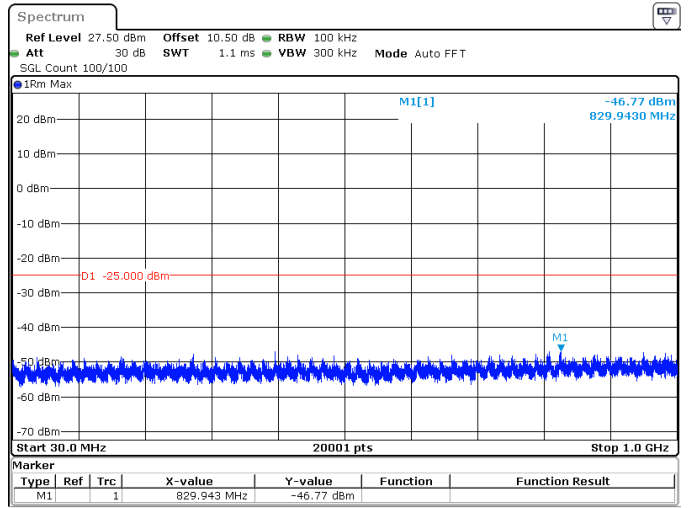
100MHz_30kHz_2592.99MHz_DFT-s-OFDM QPSK_RB1@0 -46.77 dBm
