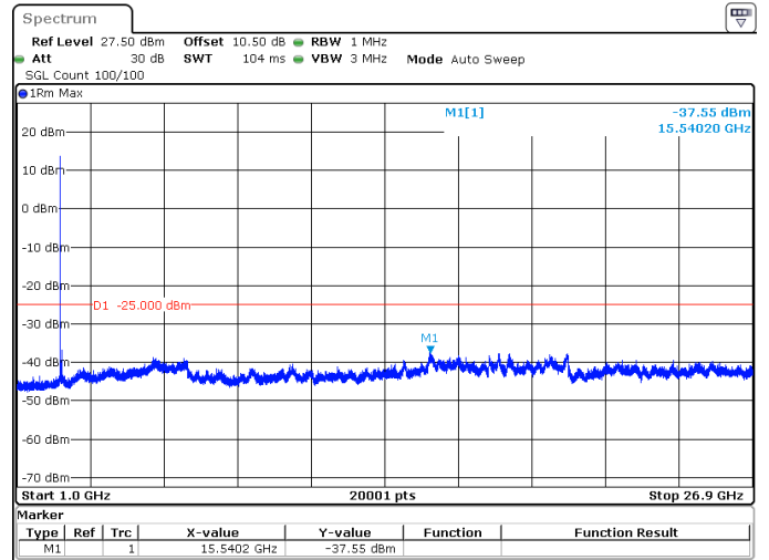
80MHz_30kHz_2536.02MHz_DFT-s-OFDM QPSK_RB1@0 -37.55 dBm
