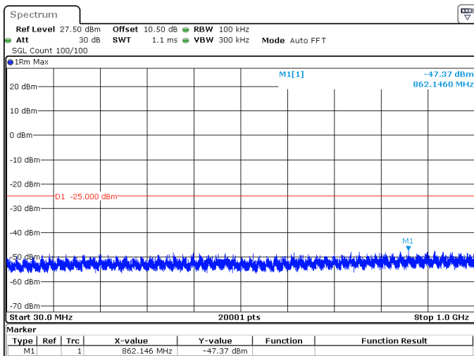
80MHz_30kHz_2592.99MHz_DFT-s-OFDM QPSK_RB216@0 -47.37 dBm
