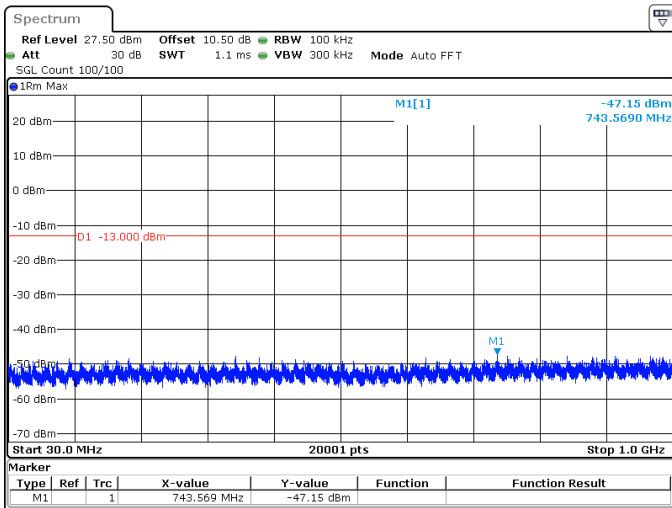
5MHz_15kHz_1712.5MHz_DFT-s-OFDM QPSK_RB1@0 -47.15 dBm
