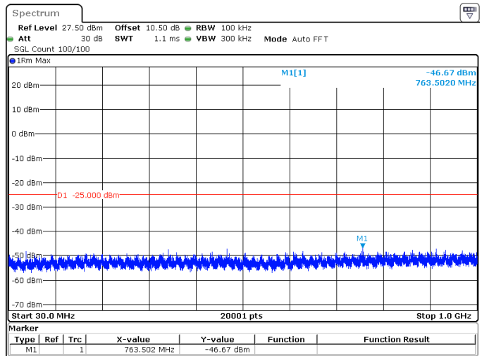
100MHz_30kHz_2592.99MHz_DFT-s-OFDM QPSK_RB270@0 -46.67 dBm
