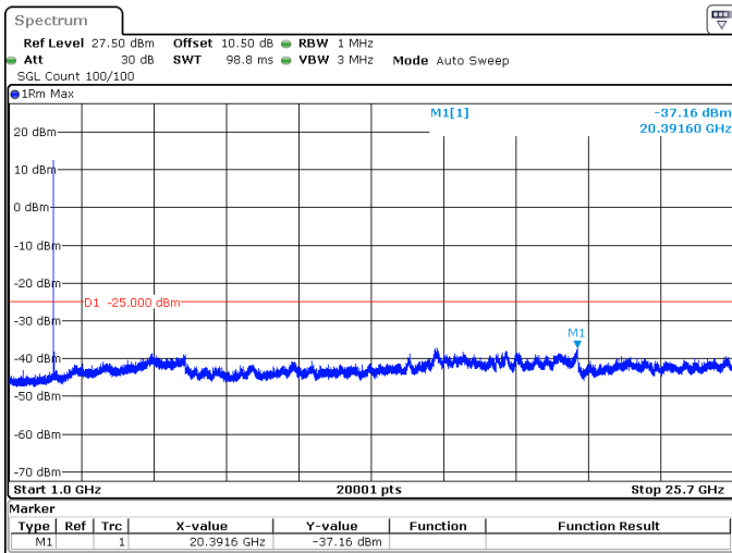
5MHz_15kHz_2502.5MHz_DFT-s-OFDM QPSK_RB1@0 -37.16 dBm
