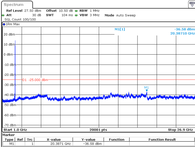
90MHz_30kHz_2644.98MHz_DFT-s-OFDM QPSK_RB1@244 -36.58 dBm
