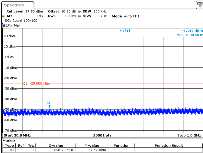
90MHz_30kHz_2644.98MHz_DFT-s-OFDM QPSK_RB1@0 -47.47 dBm
