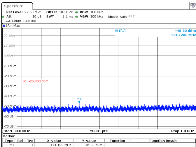
5MHz_15kHz_2502.5MHz_DFT-s-OFDM QPSK_RB25@0 -46.83 dBm
