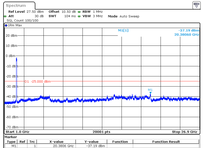
90MHz_30kHz_2592.99MHz_DFT-s-OFDM QPSK_RB243@0 -37.19 dBm
