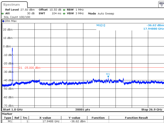
90MHz_30kHz_2644.98MHz_DFT-s-OFDM QPSK_RB243@0 -36.62 dBm
