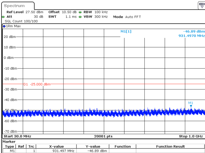
90MHz_30kHz_2592.99MHz_DFT-s-OFDM QPSK_RB243@0 -46.89 dBm
