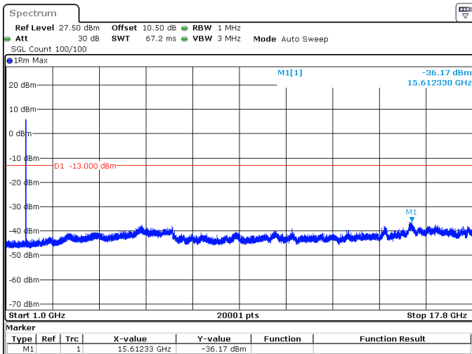
5MHz_15kHz_1712.5MHz_DFT-s-OFDM QPSK_RB25@0 -36.17 dBm
