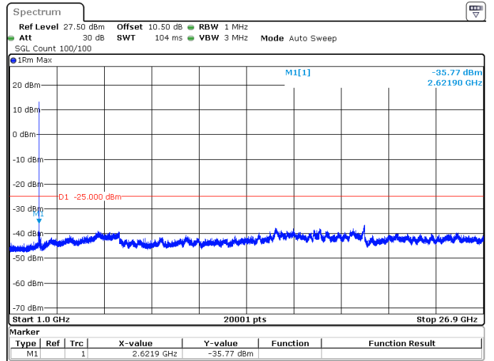
90MHz_30kHz_2644.98MHz_DFT-s-OFDM QPSK_RB1@0 -35.77 dBm
