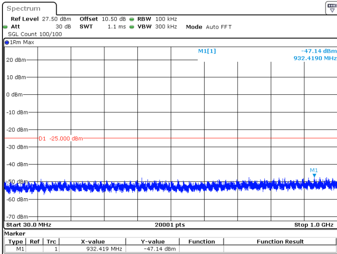
90MHz_30kHz_2592.99MHz_DFT-s-OFDM QPSK_RB1@0 -47.14 dBm
