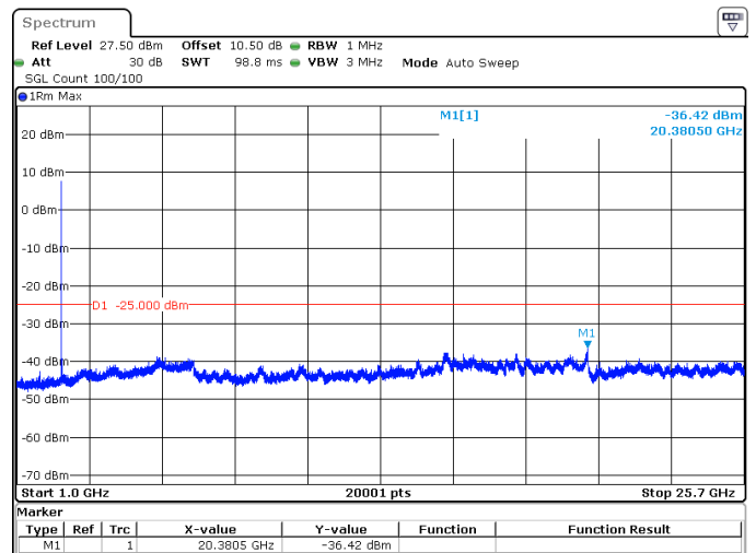
5MHz_15kHz_2502.5MHz_DFT-s-OFDM QPSK_RB25@0 -36.42 dBm
