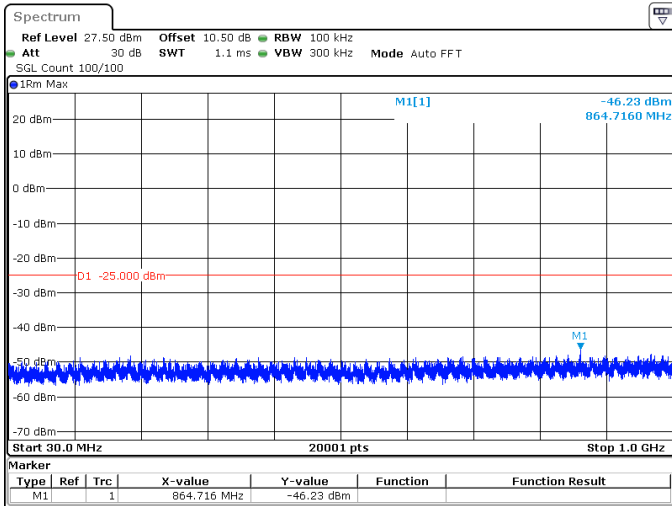
20MHz_30kHz_2592.99MHz_DFT-s-OFDM QPSK_RB1@0 -46.23 dBm
