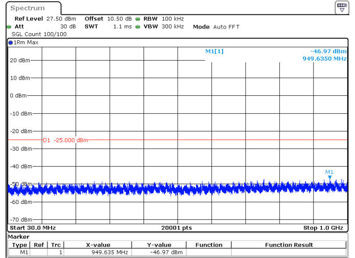
20MHz_30kHz_2679.99MHz_DFT-s-OFDM QPSK_RB1@50 -46.97 dBm
