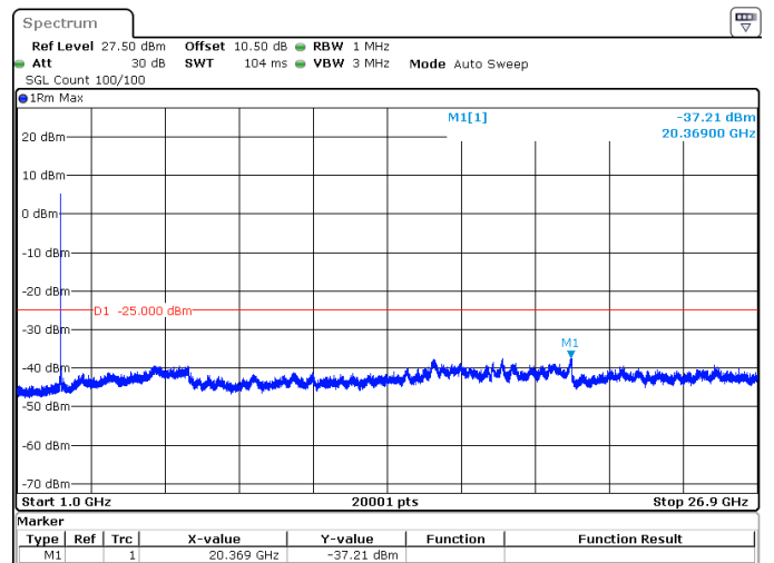
20MHz_30kHz_2506.02MHz_DFT-s-OFDM QPSK_RB50@0 -37.21 dBm
