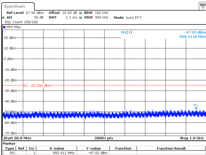
20MHz_30kHz_2592.99MHz_DFT-s-OFDM QPSK_RB50@0 -47.55 dBm
