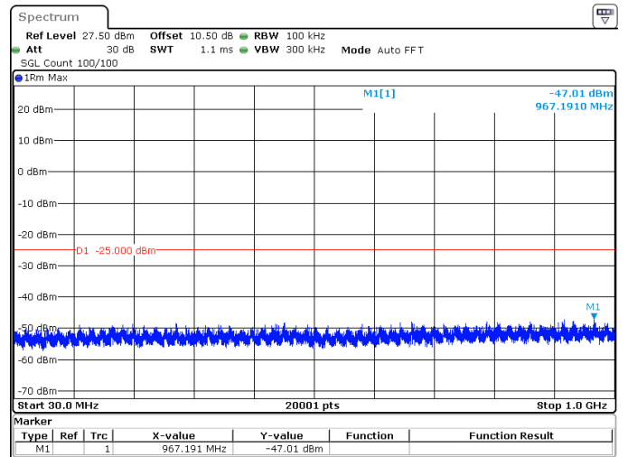
20MHz_30kHz_2679.99MHz_DFT-s-OFDM QPSK_RB50@0 -47.01 dBm
