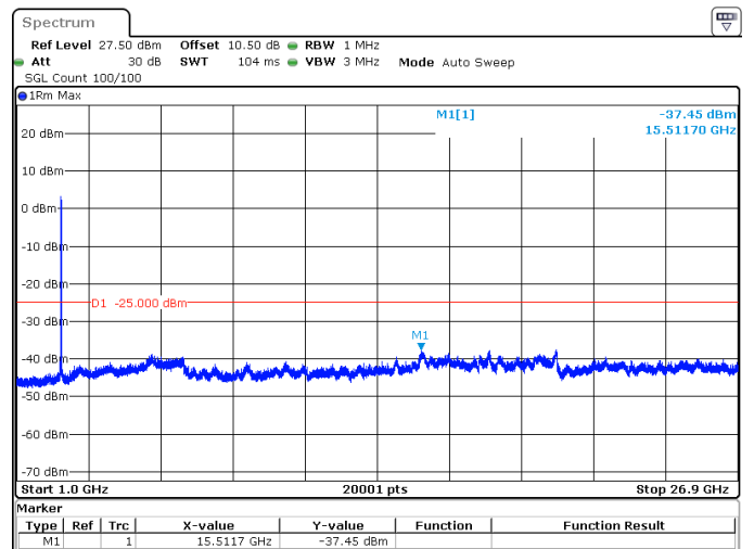
30MHz_30kHz_2592.99MHz_DFT-s-OFDM QPSK_RB75@0 -37.45 dBm
