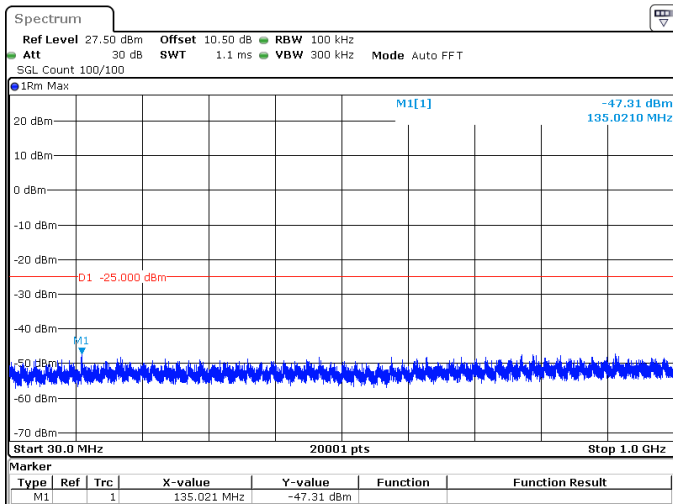
50MHz_15kHz_2664.99MHz_DFT-s-OFDM QPSK_RB270@0 -47.31 dBm
