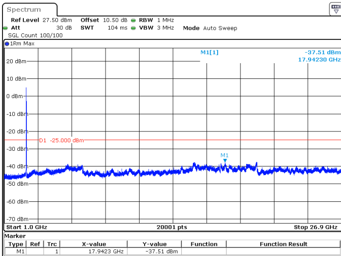
20MHz_30kHz_2679.99MHz_DFT-s-OFDM QPSK_RB50@0 -37.51 dBm
