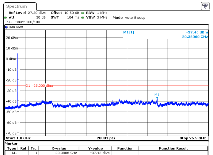
20MHz_30kHz_2592.99MHz_DFT-s-OFDM QPSK_RB50@0 -37.45 dBm
