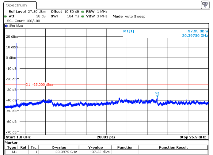
20MHz_30kHz_2506.02MHz_DFT-s-OFDM QPSK_RB1@0 -37.33 dBm
