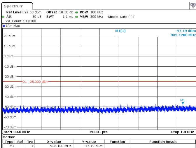
20MHz_30kHz_2506.02MHz_DFT-s-OFDM QPSK_RB50@0 -47.19 dBm
