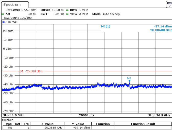
20MHz_30kHz_2506.02MHz_DFT-s-OFDM QPSK_RB1@50 -37.14 dBm
