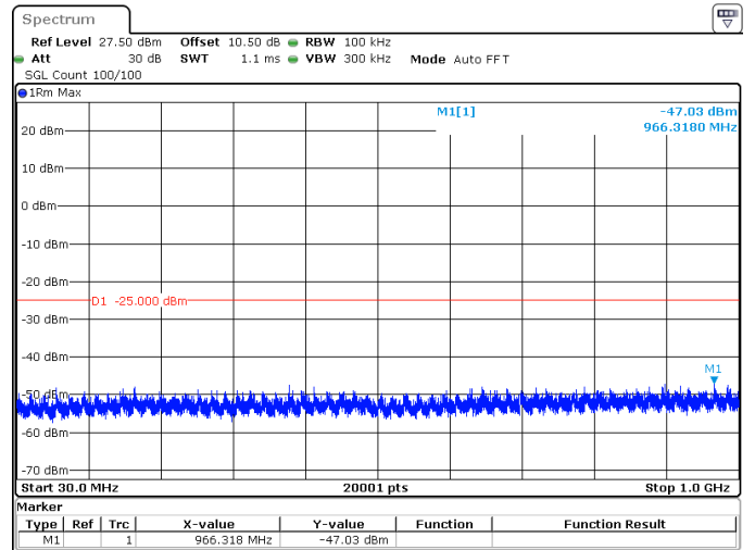
20MHz_30kHz_2506.02MHz_DFT-s-OFDM QPSK_RB1@50 -47.03 dBm
