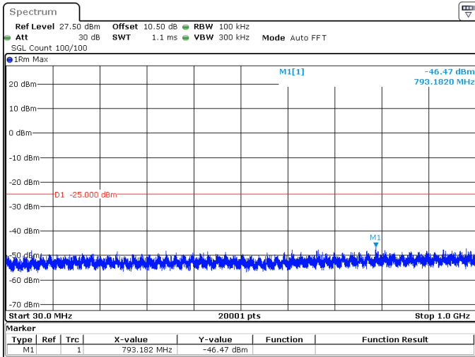
20MHz_30kHz_2506.02MHz_DFT-s-OFDM QPSK_RB1@0 -46.47 dBm
