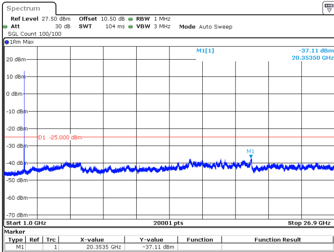
60MHz_30kHz_2592.99MHz_DFT-s-OFDM QPSK_RB1@0 -37.11 dBm
