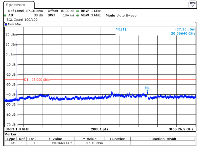
20MHz_30kHz_2592.99MHz_DFT-s-OFDM QPSK_RB1@0 -37.15 dBm
