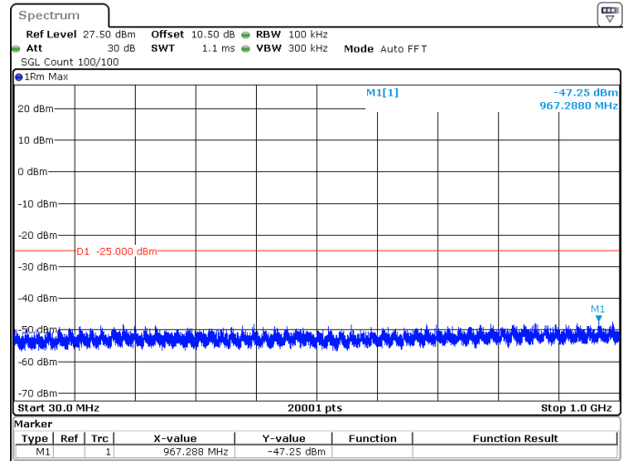
60MHz_30kHz_2592.99MHz_DFT-s-OFDM QPSK_RB1@0 -47.25 dBm
