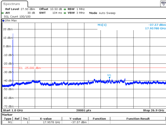
20MHz_30kHz_2679.99MHz_DFT-s-OFDM QPSK_RB1@50 -37.57 dBm
