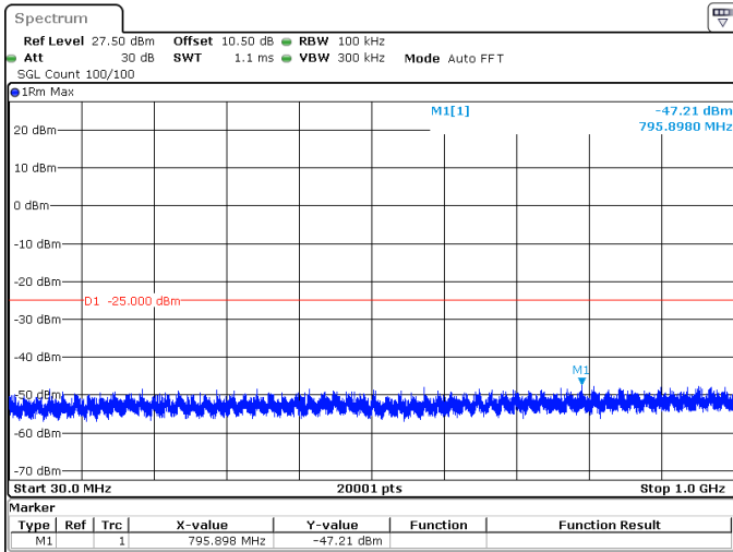
20MHz_30kHz_2679.99MHz_DFT-s-OFDM QPSK_RB1@0 -47.21 dBm
