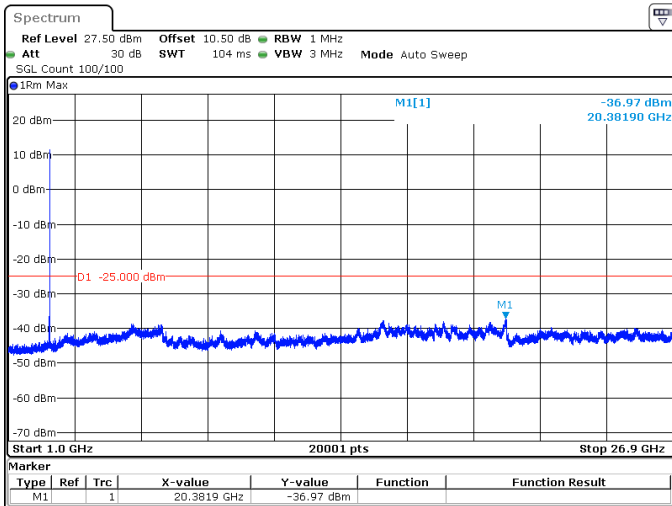
20MHz_30kHz_2592.99MHz_DFT-s-OFDM QPSK_RB1@50 -36.97 dBm
