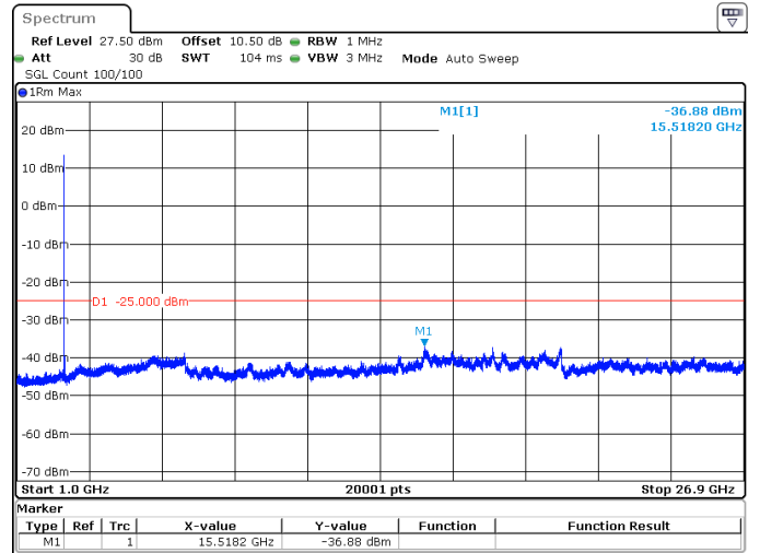
20MHz_30kHz_2679.99MHz_DFT-s-OFDM QPSK_RB1@0 -36.88 dBm
