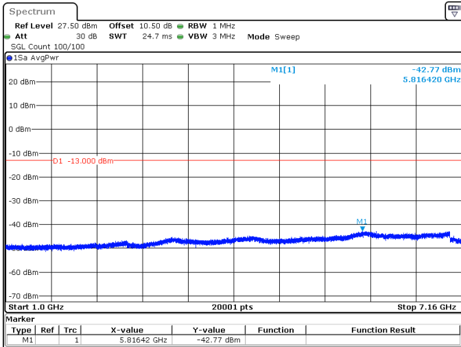
5MHz_15kHz_701.5MHz_DFT-s-OFDM QPSK_RB1@0 -42.77 dBm
