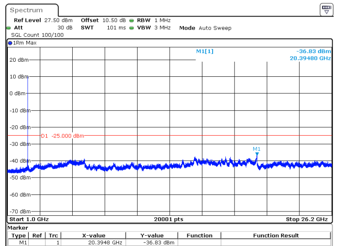
5MHz_15kHz_2572.5MHz_DFT-s-OFDM QPSK_RB25@0 -36.83 dBm
