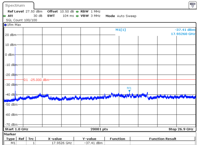
10MHz_15kHz_2501.01MHz_DFT-s-OFDM QPSK_RB50@0 -37.41 dBm
