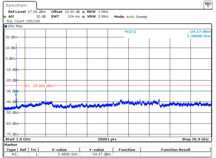
10MHz_15kHz_2501.01MHz_DFT-s-OFDM QPSK_RB1@0 -34.57 dBm
