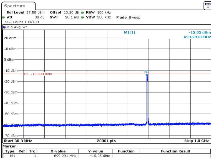
5MHz_15kHz_701.5MHz_DFT-s-OFDM QPSK_RB25@0 -15.05 dBm
