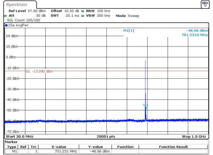
5MHz_15kHz_701.5MHz_DFT-s-OFDM QPSK_RB1@0 -48.86 dBm
