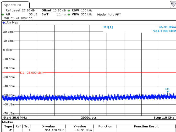
10MHz_15kHz_2501.01MHz_DFT-s-OFDM QPSK_RB50@0 -46.91 dBm
