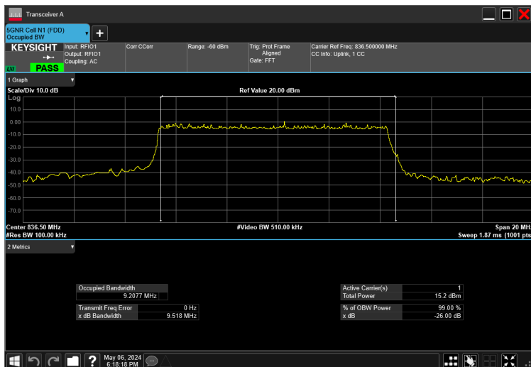
10MHz_15kHz_836.5MHz_DFT-s-OFDM QPSK_RB50@0 9.208 MHz
