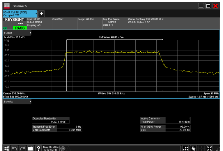
10MHz_15kHz_836.5MHz_DFT-s-OFDM pi/2 BPSK_RB50@0 9.207 MHz
