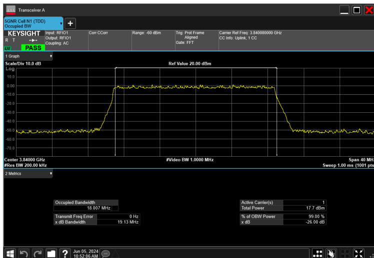
20MHz_30kHz_3840MHz_DFT-s-OFDM 16 QAM_RB50@0 18.007 MHz
