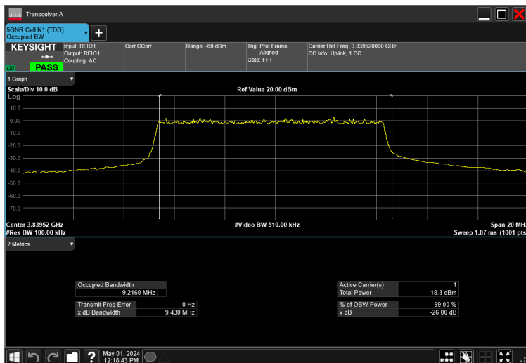
10MHz_15kHz_3840MHz_DFT-s-OFDM QPSK_RB50@0 9.216 MHz
