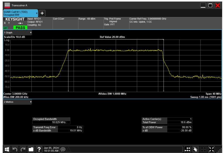
20MHz_30kHz_3840MHz_DFT-s-OFDM QPSK_RB50@0 18.029 MHz
