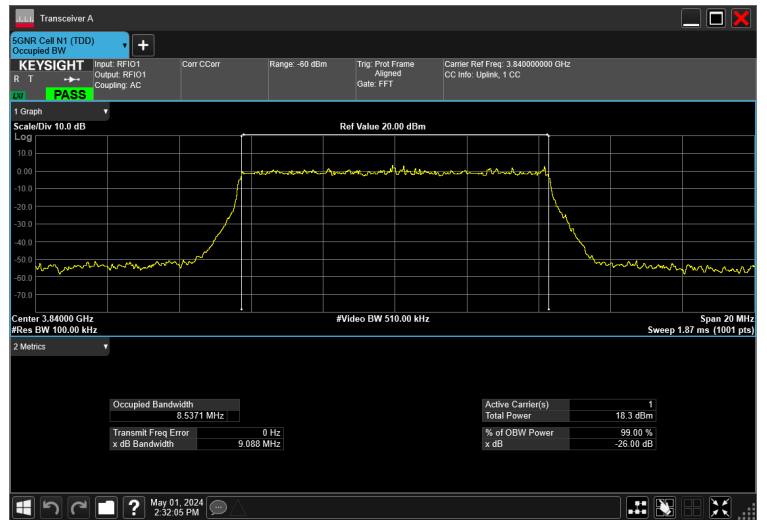
10MHz_30kHz_3840MHz_DFT-s-OFDM QPSK_RB24@0 8.537 MHz
