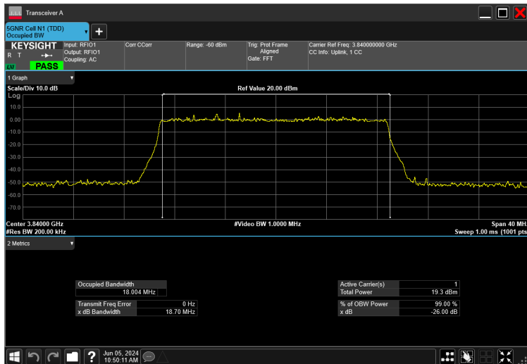
20MHz_30kHz_3840MHz_DFT-s-OFDM \pi/2 BPSK_RB50@0 18.004 MHz
