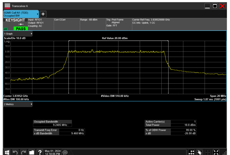
10MHz_15kHz_3840MHz_DFT-s-OFDM pi/2 BPSK_RB50@0 9.240 MHz
