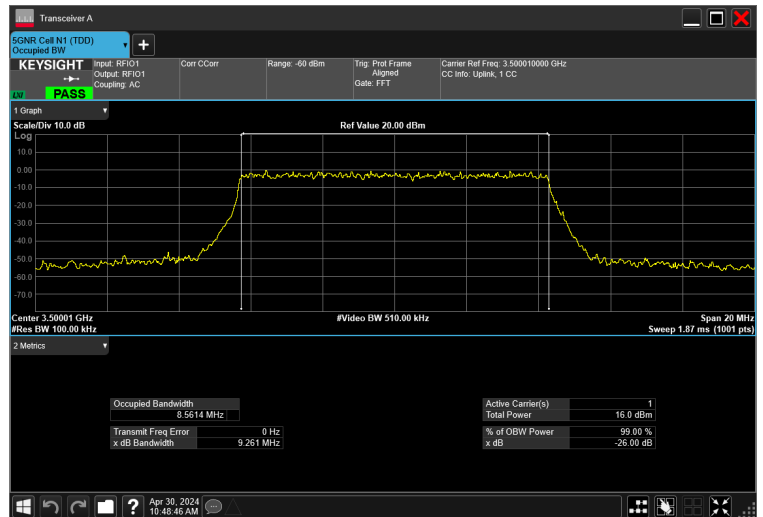
10MHz_30kHz_3500MHz_CP-OFDM QPSK_RB24@0 8.561 MHz
