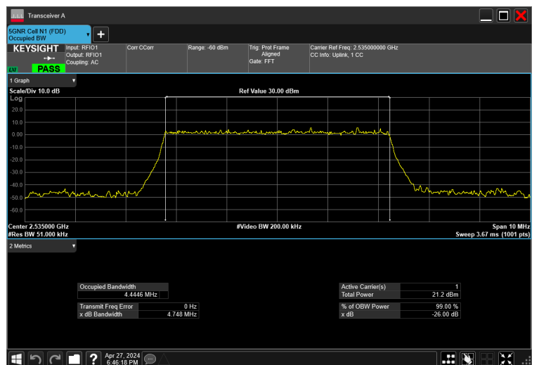
5MHz_15kHz_2535MHz_DFT-s-OFDM \pi/2 BPSK_RB25@0 4.445 MHz
