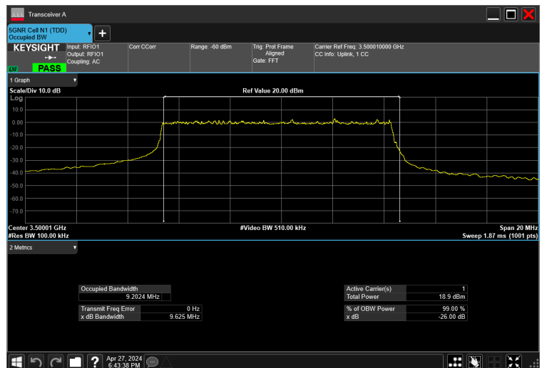
10MHz_15kHz_3500MHz_DFT-s-OFDM \pi/2 BPSK_RB50@0 9.202 MHz
