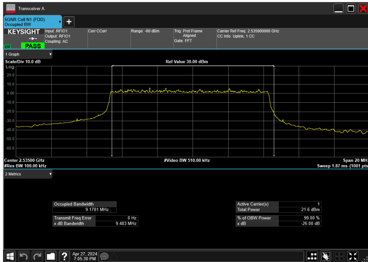
10MHz_15kHz_2535MHz_DFT-s-OFDM \pi/2 BPSK_RB50@0 9.178 MHz
