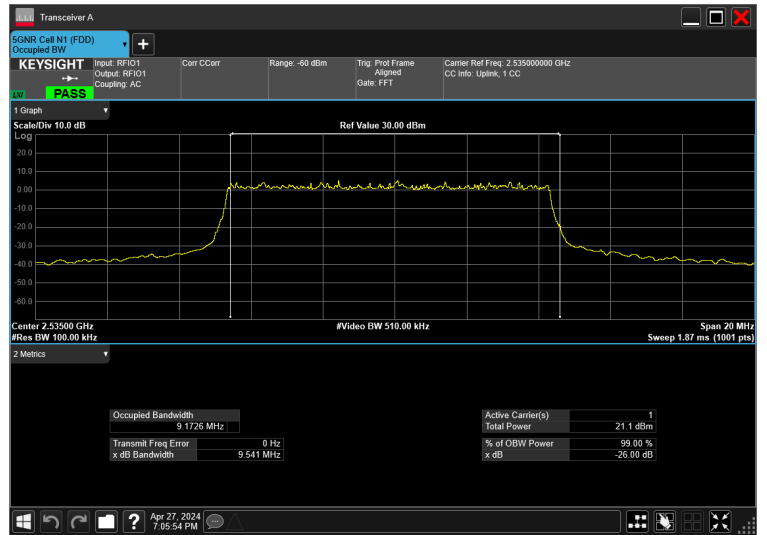
10MHz_15kHz_2535MHz_DFT-s-OFDM QPSK_RB50@0 9.173 MHz
