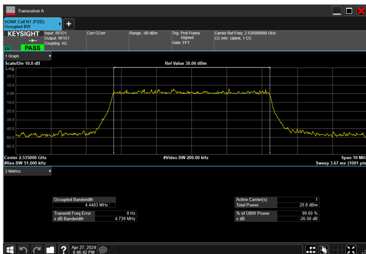
5MHz_15kHz_2535MHz_DFT-s-OFDM QPSK_RB25@0 4.448 MHz
