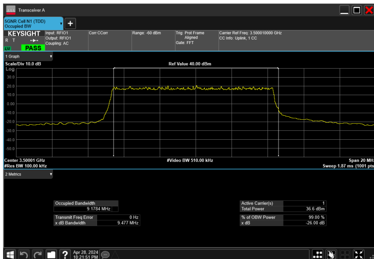
10MHz_15kHz_3500MHz_DFT-s-OFDM QPSK_RB50@0 9.178 MHz
