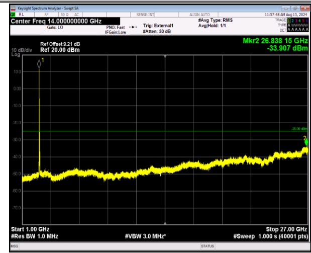
41-41-20MHz-20MHz-QPSK-QPSK-40340-40538-1RB#0- 1RB#99-1000~27000MHz-PASS
