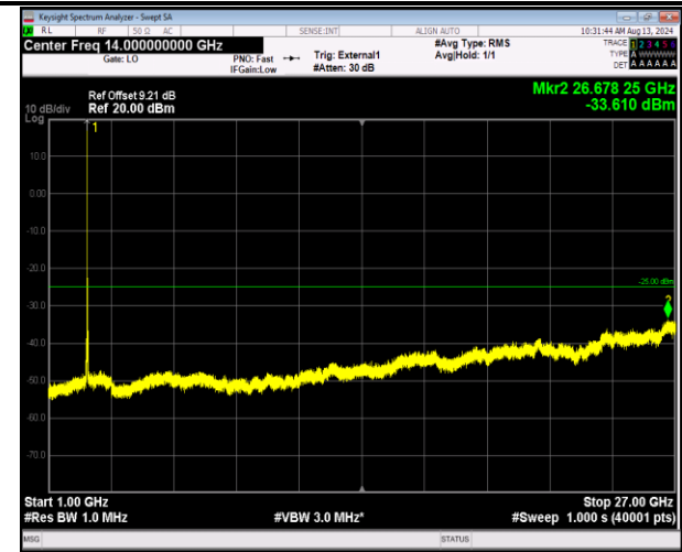
41-41-20MHz-5MHz-QPSK-QPSK-40715-40832-1RB#0-0RB#0-1000~27000MHz-PASS
