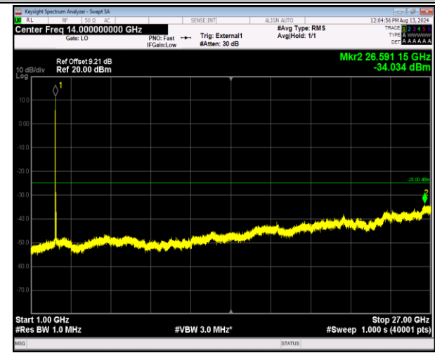
41-41-20MHz-20MHz-QPSK-QPSK-40641-40839-1RB#0- 1RB#99-1000~27000MHz-PASS
