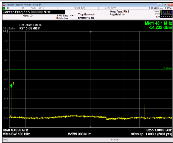
41-41-20MHz-20MHz-QPSK-QPSK-40641-40839-1RB# 99-0RB#0-30~1000MHz-PASS
