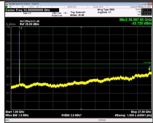
41-41-20MHz-20MHz-QPSK-QPSK-40641-40839-1RB#0- 0RB#0-1000~27000MHz-PASS
