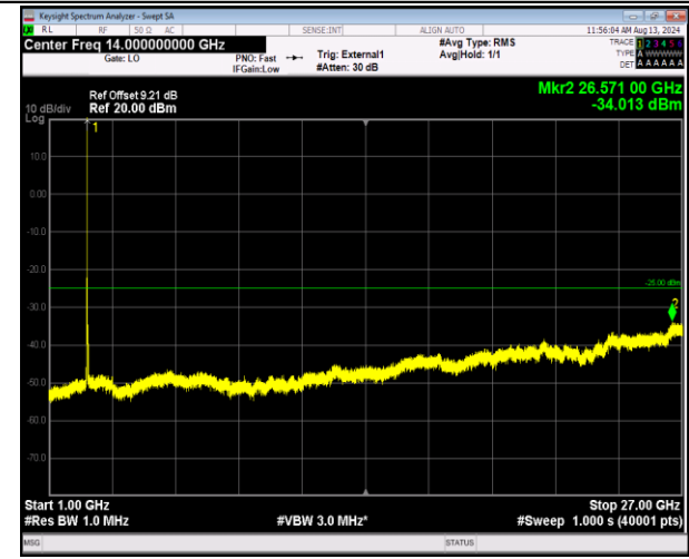
41-41-20MHz-20MHz-QPSK-QPSK-40340-40538-1RB#9 9-ORB#0-1000~27000MHz-PASS
