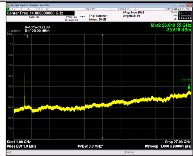
41-41-20MHz-5MHz-QPSK-QPSK-41090-41207-1RB#99-0RB#0-1000~27000MHz-PASS
