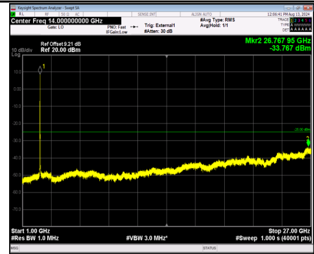
41-41-20MHz-20MHz-QPSK-QPSK-40641-40839-100RB #0-100RB#0-1000~27000MHz-PASS
