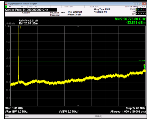
41-41-20MHz-20MHz-QPSK-QPSK-40340-40538-1RB#0- ORB#0-1000~27000MHz-PASS
