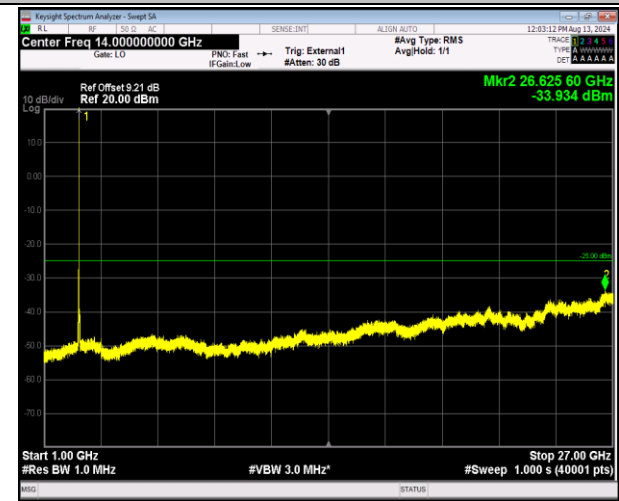
41-41-20MHz-20MHz-QPSK-QPSK-40641-40839-1RB#9 9-0RB#0-1000~27000MHz-PASS
