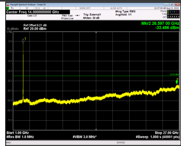
41-41-20MHz-5MHz-QPSK-QPSK-40715-40832-100RB# 0-25RB#0-1000~27000MHz-PASS
