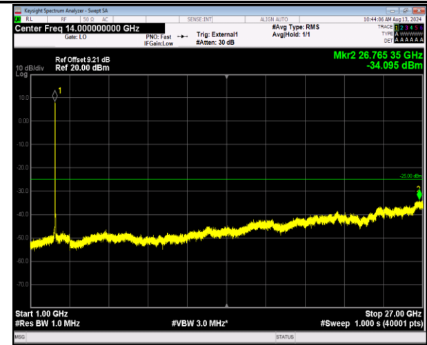
41-41-20MHz-5MHz-QPSK-QPSK-41090-41207-100RB# 0-25RB#0-1000~27000MHz-PASS
