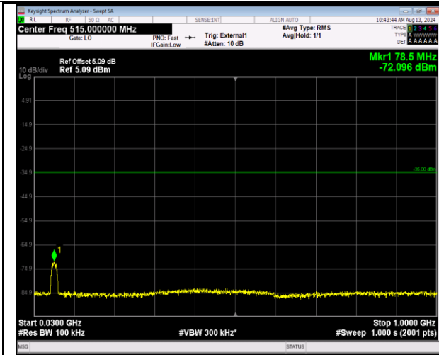
41-41-20MHz-5MHz-QPSK-QPSK-41090-41207-100RB #0-25RB#0-30~1000MHz-PASS
