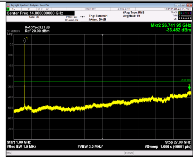
41-41-20MHz-5MHz-QPSK-QPSK-40715-40832-1RB#0-1RB#24-1000~27000MHz-PASS
