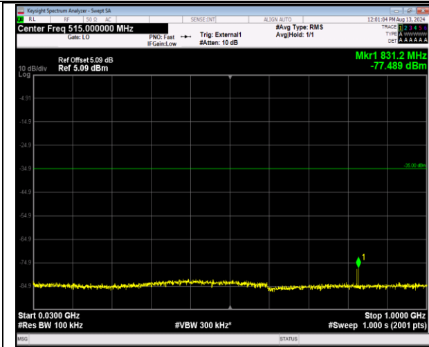
41-41-20MHz-20MHz-QPSK-QPSK-40641-40839-1RB# 0-0RB#0-30~1000MHz-PASS
