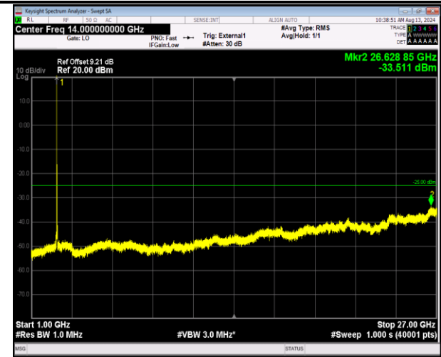
41-41-20MHz-5MHz-QPSK-QPSK-41090-41207-1RB#0-0RB#0-1000~27000MHz-PASS
