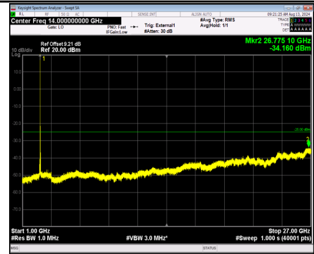
41-41-5MHz-20MHz-QPSK-QPSK-40648-40765-1RB#0-0RB#0-1000~27000MHz-PASS
