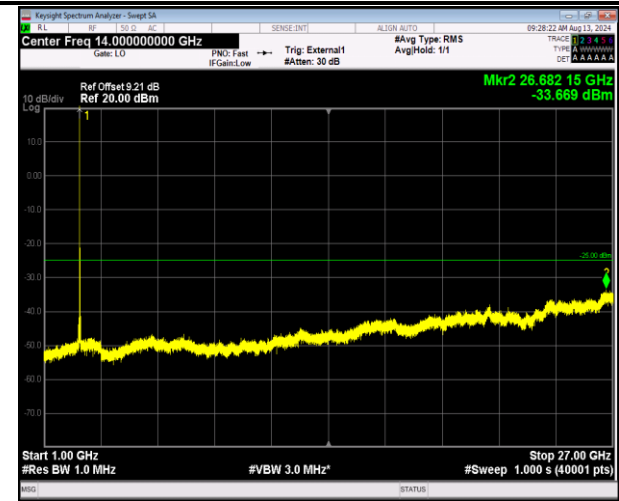
41-41-5MHz-20MHz-QPSK-QPSK-41023-41140-1RB#0-0RB#0-1000~27000MHz-PASS
