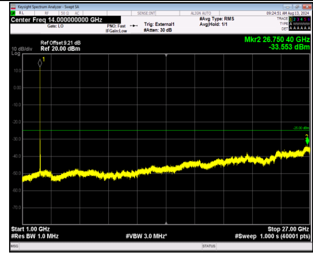
41-41-5MHz-20MHz-QPSK-QPSK-40648-40765-1RB#0-1RB#99-1000~27000MHz-PASS
