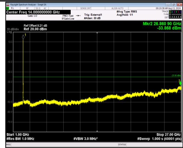
41-41-5MHz-20MHz-QPSK-QPSK-40273-40390-25RB#0- 100RB#0-1000~27000MHz-PASS
