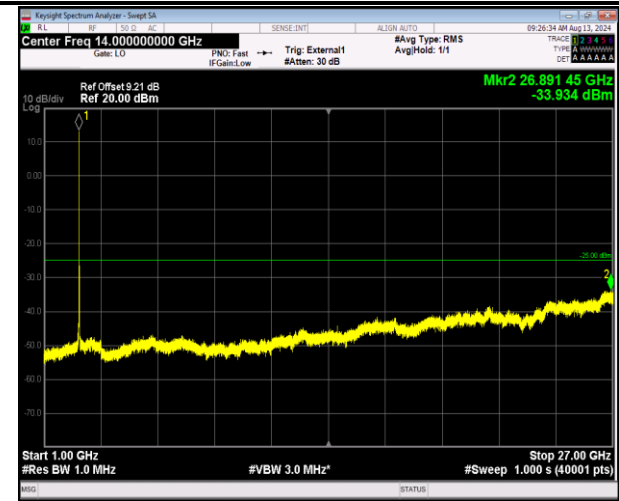
41-41-5MHz-20MHz-QPSK-QPSK-40648-40765-25RB#0- 100RB#0-1000~27000MHz-PASS
