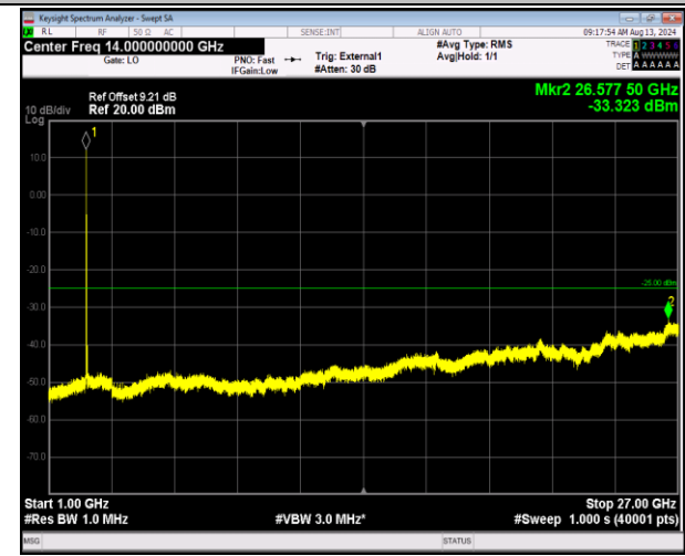
41-41-5MHz-20MHz-QPSK-QPSK-40273-40390-1RB#0-1RB#99-1000~27000MHz-PASS
