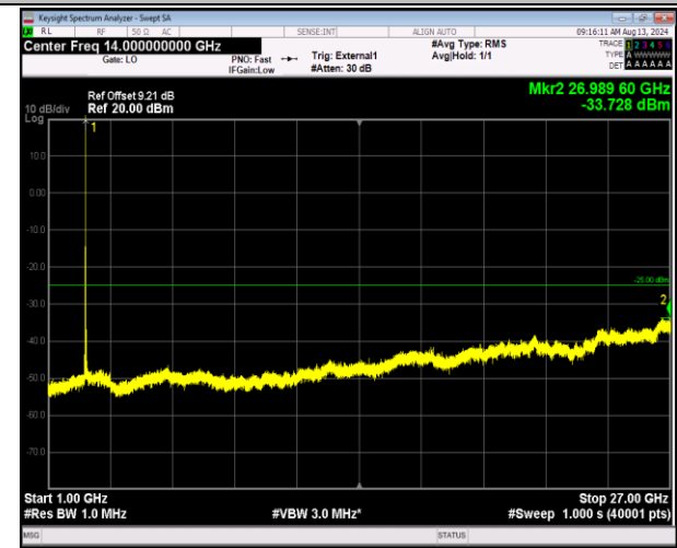
41-41-5MHz-20MHz-QPSK-QPSK-40273-40390-1RB#24-0RB#0-1000~27000MHz-PASS
