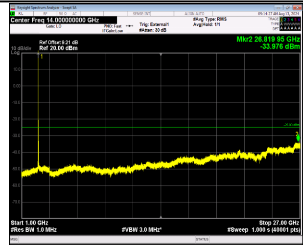
41-41-5MHz-20MHz-QPSK-QPSK-40273-40390-1RB#0-0RB#0-1000~27000MHz-PASS
