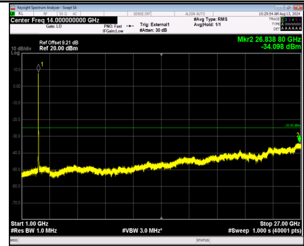
41-41-20MHz-5MHz-QPSK-QPSK-40340-40457-100RB# 0-25RB#0-1000~27000MHz-PASS
