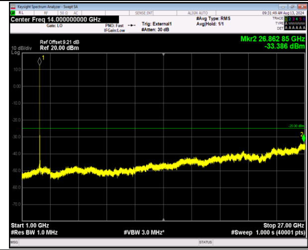
41-41-5MHz-20MHz-QPSK-QPSK-41023-41140-1RB#0-1RB#99-1000~27000MHz-PASS
