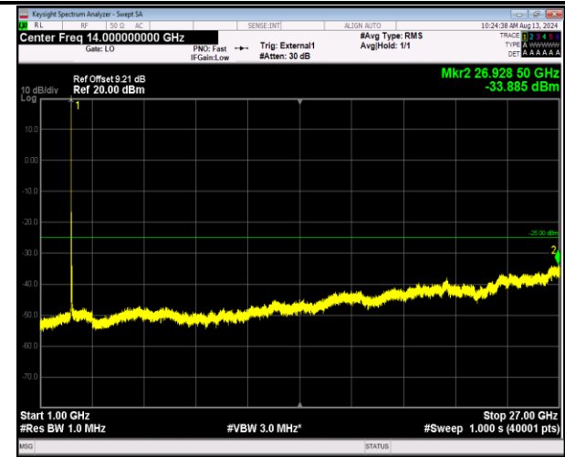
41-41-20MHz-5MHz-QPSK-QPSK-40340-40457-1RB#0-0RB#0-1000~27000MHz-PASS
