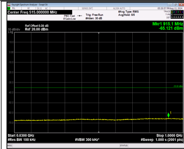
7-7-20MHz-10MHz-QPSK-QPSK-21251-21395-100RB# 0-50RB#0-30~1000MHz-PASS
