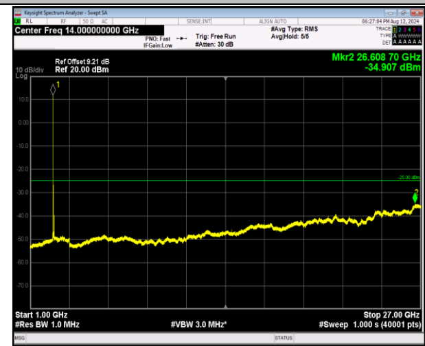
7-7-20MHz-20MHz-QPSK-QPSK-21001-21199-1RB#0-1 RB#99-1000~27000MHz-PASS
