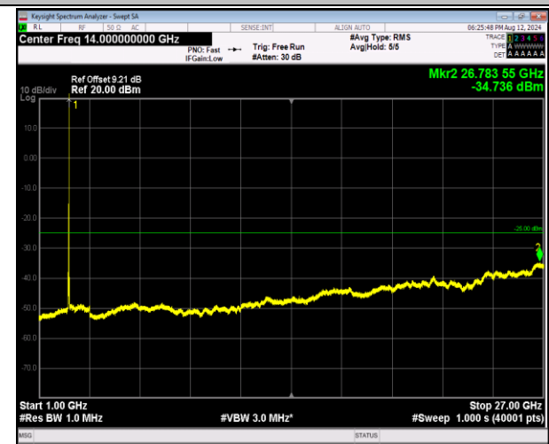
7-7-20MHz-20MHz-QPSK-QPSK-21001-21199-1RB#99-0 RB#0-1000~27000MHz-PASS
