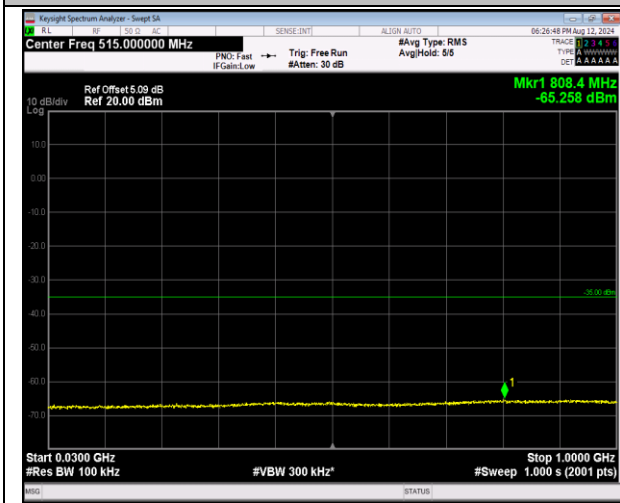
7-7-20MHz-20MHz-QPSK-QPSK-21001-21199-1RB#0-1 RB#99-30~1000MHz-PASS
