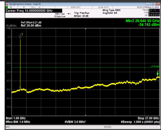
7-7-20MHz-10MHz-QPSK-QPSK-21251-21395-100RB#0- 50RB#0-1000~27000MHz-PASS
