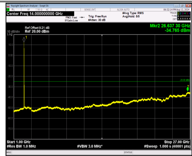
7-7-20MHz-20MHz-QPSK-QPSK-21152-21350-1RB#0-1 RB#99-1000~27000MHz-PASS
