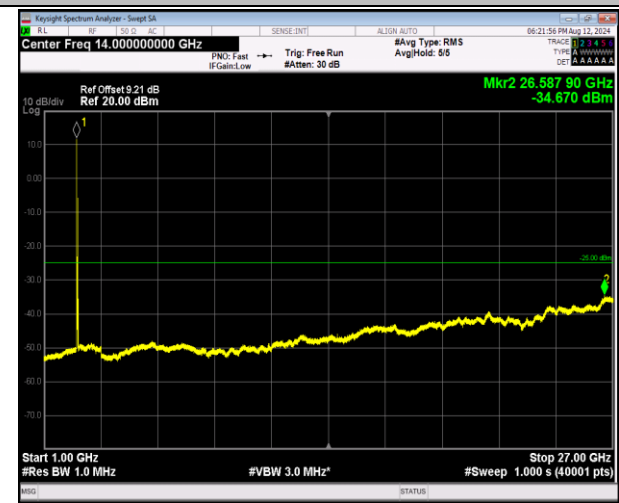
7-7-20MHz-20MHz-QPSK-QPSK-20850-21048-1RB#0-1 RB#99-1000~27000MHz-PASS
