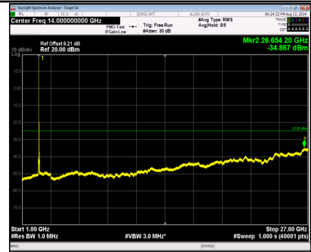
7-7-20MHz-20MHz-QPSK-QPSK-21001-21199-1RB#0-0 RB#0-1000~27000MHz-PASS
