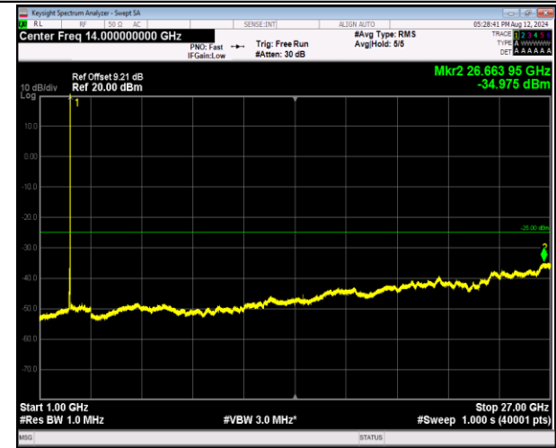
7-7-20MHz-10MHz-QPSK-QPSK-21251-21395-1RB#99-0 RB#0-1000~27000MHz-PASS
