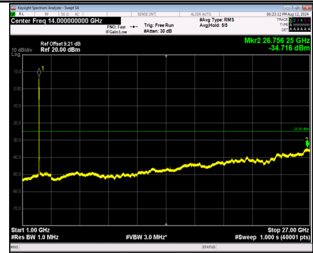
7-7-20MHz-20MHz-QPSK-QPSK-20850-21048-100RB#0- 100RB#0-1000~27000MHz-PASS
