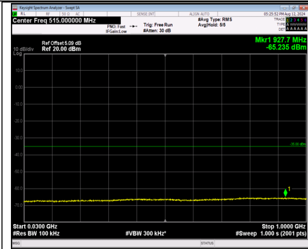
7-7-20MHz-10MHz-QPSK-QPSK-21051-21195-100RB#0-50RB#0-30~1000MHz-PASS
