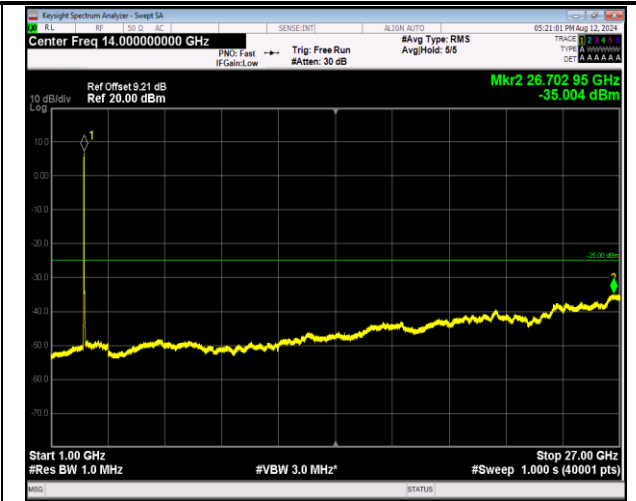
7-7-20MHz-10MHz-QPSK-QPSK-20850-20994-100RB#0-50RB#0-1000~27000MHz-PASS
