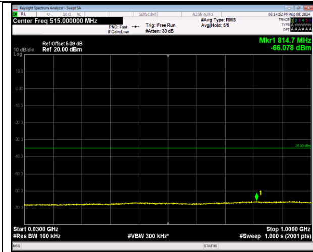
7-7-10MHz-20MHz-QPSK-QPSK-20805-20949-50RB#0-100RB#0-30~1000MHz-PASS
