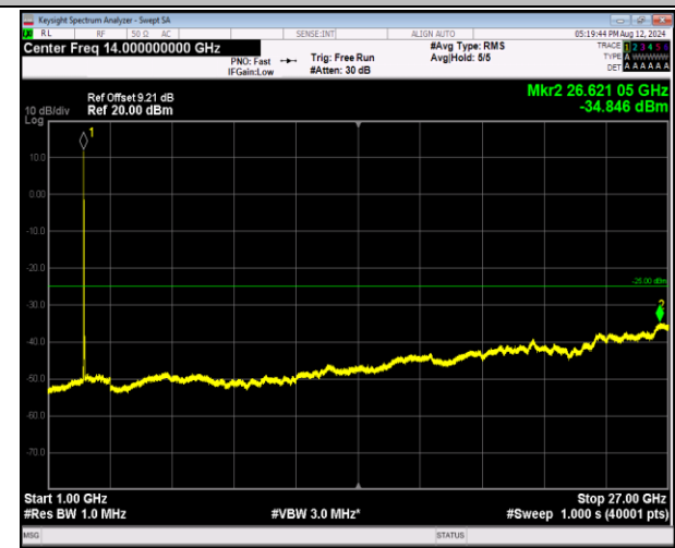
7-7-20MHz-10MHz-QPSK-QPSK-20850-20994-1RB#0-1 RB#49-1000~27000MHz-PASS
