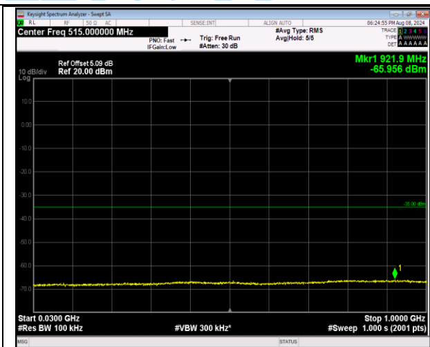
7-7-10MHz-20MHz-QPSK-QPSK-21206-21350-50RB#0-100RB#0-30~1000MHz-PASS
