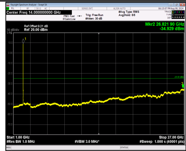
7-7-10MHz-20MHz-QPSK-QPSK-20805-20949-50RB#0-100RB#0-1000~27000MHz-PASS
