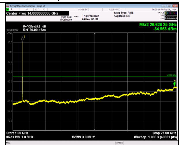
7-7-10MHz-20MHz-QPSK-QPSK-21206-21350-50RB#0-100RB#0-1000~27000MHz-PASS
