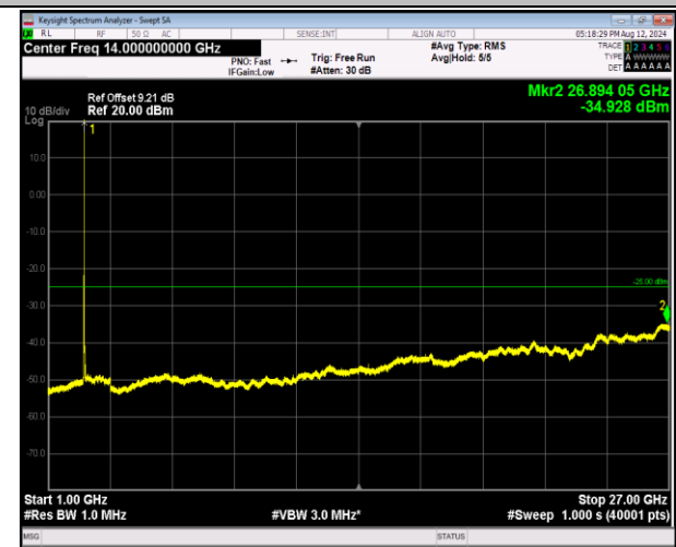
7-7-20MHz-10MHz-QPSK-QPSK-20850-20994-1RB#99-0 RB#0-1000~27000MHz-PASS
