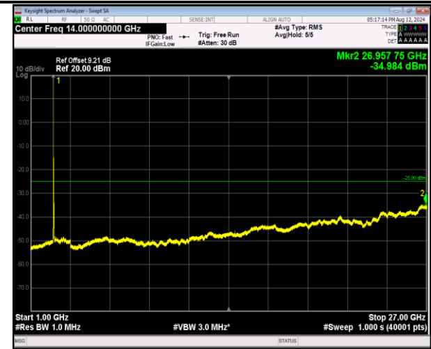
7-7-20MHz-10MHz-QPSK-QPSK-20850-20994-1RB#0-0 RB#0-1000~27000MHz-PASS
