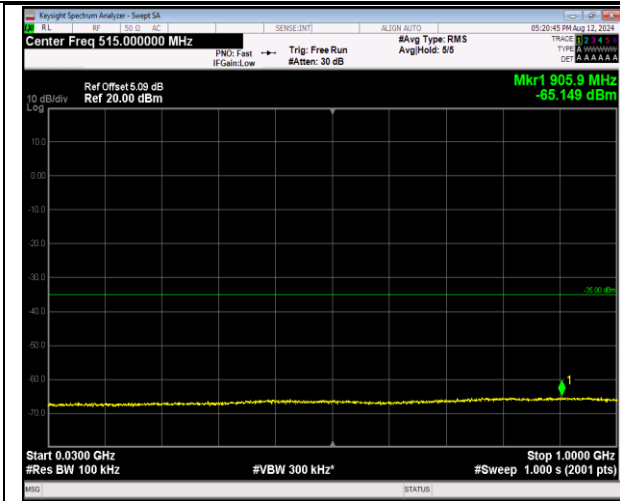
7-7-20MHz-10MHz-QPSK-QPSK-20850-20994-100RB#0-50RB#0-30~1000MHz-PASS
