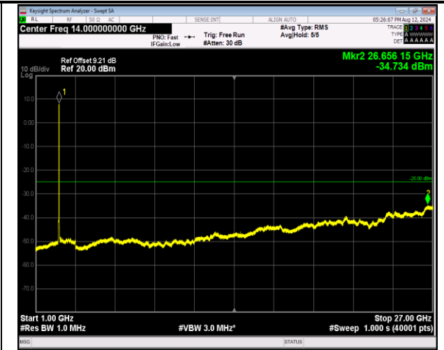
7-7-20MHz-10MHz-QPSK-QPSK-21051-21195-100RB#0-50RB#0-1000~27000MHz-PASS
