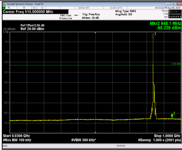
5-5-5MHz-3MHz-QPSK-QPSK-20595-20634-1RB#0-1R B#15-30~1000MHz-PASS
