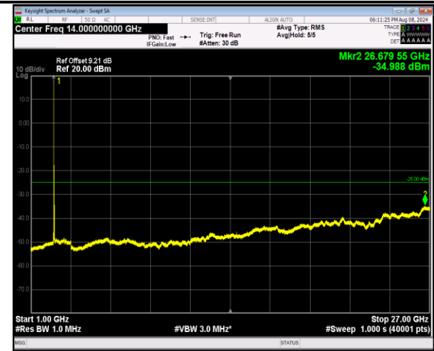
7-7-10MHz-20MHz-QPSK-QPSK-20805-20949-1RB#0-0 RB#0-1000~27000MHz-PASS
