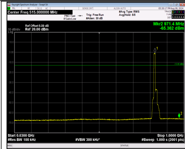
5-5-10MHz-10MHz-QPSK-QPSK-20476-20575-50RB#0-50RB#0-30~1000MHz-PASS
