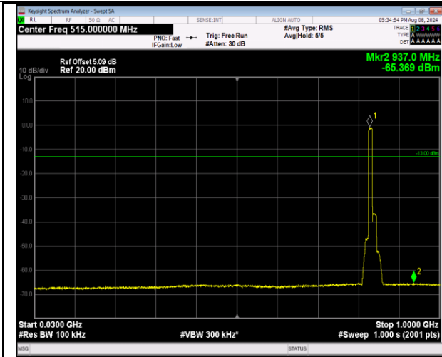
5-5-10MHz-10MHz-QPSK-QPSK-20501-20600-50RB#0-50RB#0-30~1000MHz-PASS
