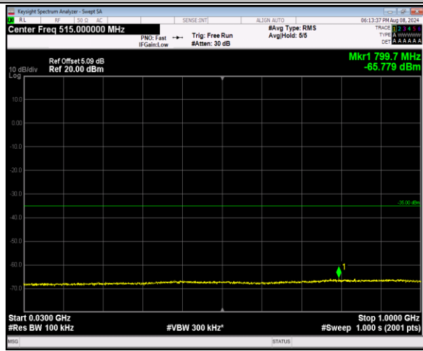
7-7-10MHz-20MHz-QPSK-QPSK-20805-20949-1RB#0-1 RB#99-30~1000MHz-PASS
