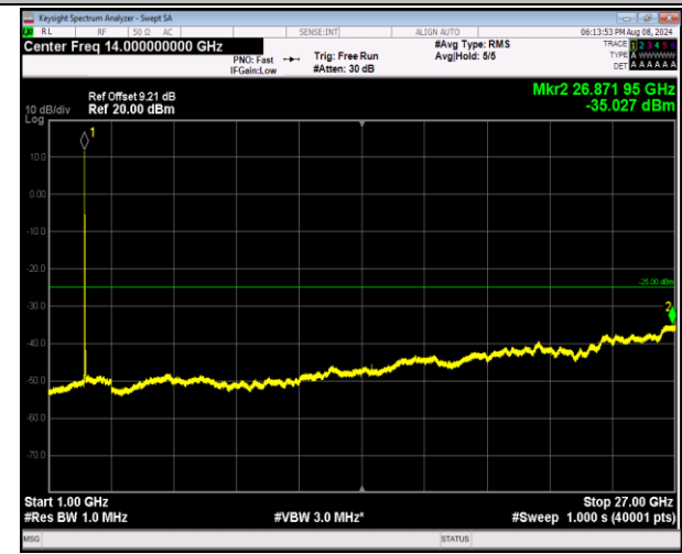
7-7-10MHz-20MHz-QPSK-QPSK-20805-20949-1RB#0-1 RB#99-1000~27000MHz-PASS
