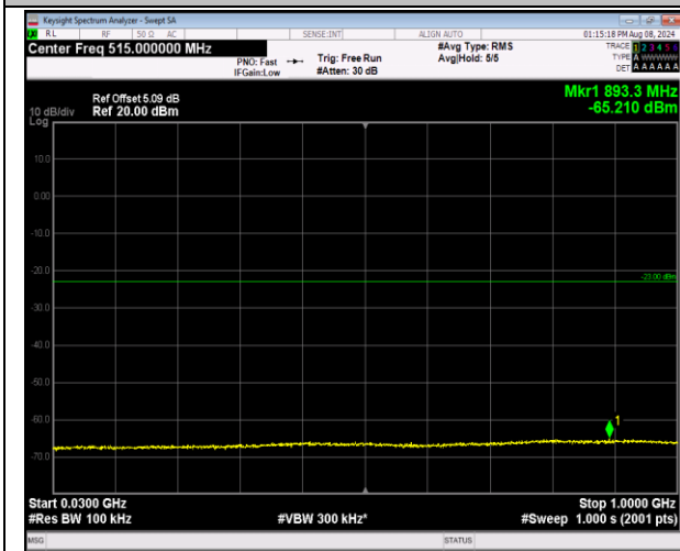
2-2-20MHz-20MHz-16QAM-16QAM-18700-18898-1RB# 0-1RB#99-30~1000MHz-PASS
