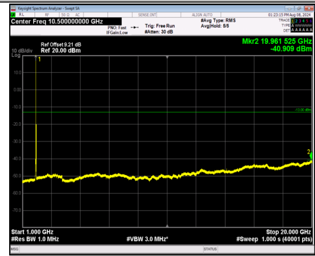
2-2-20MHz-20MHz-16QAM-16QAM-18902-19100-1RB#0 -0RB#0-1000~20000MHz-PASS
