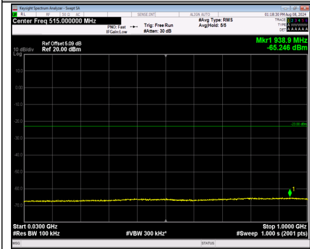
2-2-20MHz-20MHz-QPSK-QPSK-18801-18999-1RB#99-0 ORB#0-30~1000MHz-PASS
