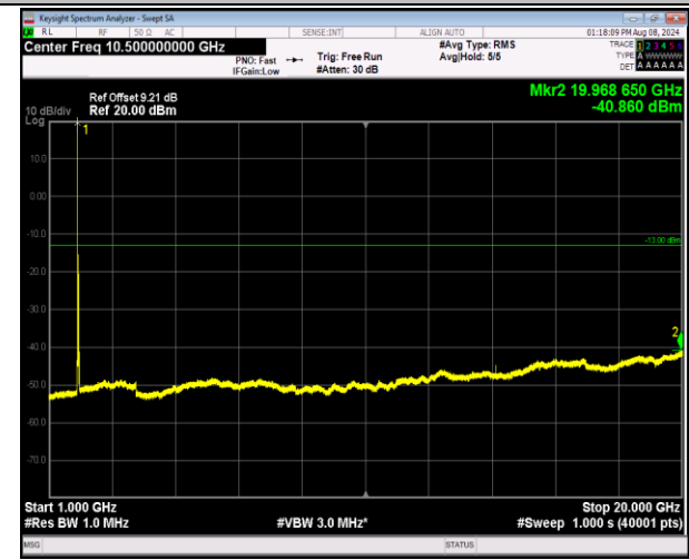
2-2-20MHz-20MHz-16QAM-16QAM-18801-18999-1RB#0 -0RB#0-1000~20000MHz-PASS
