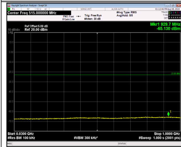
2-2-20MHz-20MHz-16QAM-16QAM-18700-18898-1RB# 0-0RB#0-30~1000MHz-PASS
