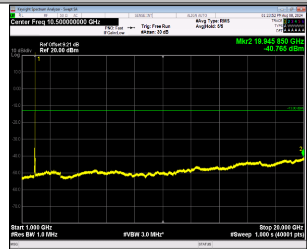
2-2-20MHz-20MHz-QPSK-QPSK-18902-19100-1RB#99-0 RB#0-1000~20000MHz-PASS
