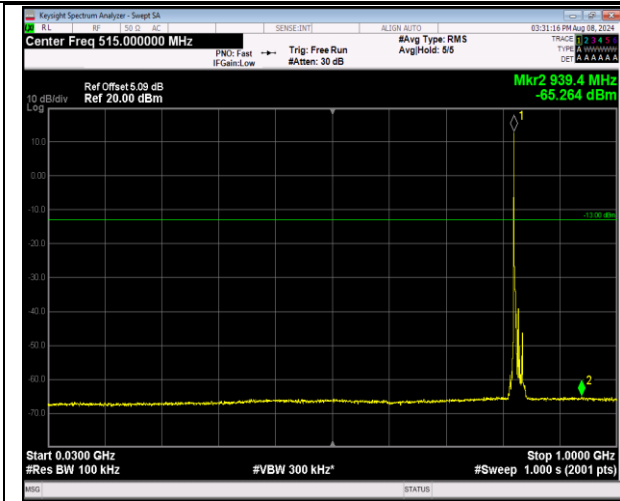
5-5-3MHz-5MHz-QPSK-QPSK-20416-20455-1RB#0-0R B#0-30~1000MHz-PASS
