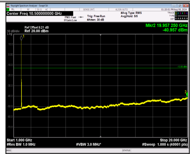
2-2-20MHz-20MHz-QPSK-QPSK-18801-18999-1RB#0-1 RB#99-1000~20000MHz-PASS
