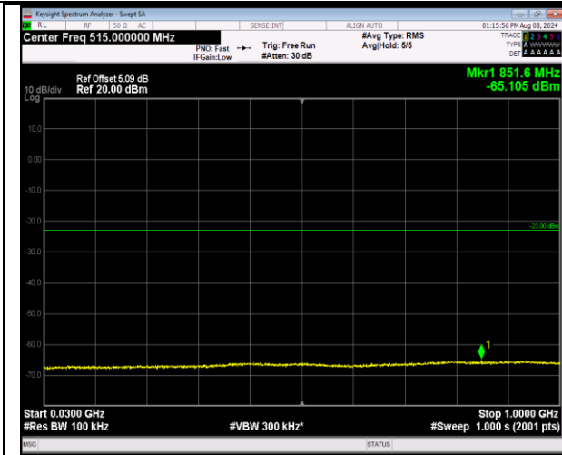
2-2-20MHz-20MHz-QPSK-QPSK-18700-18898-100RB# 0-100RB#0-30~1000MHz-PASS
