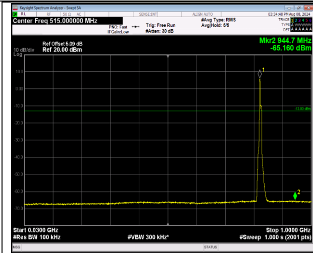
5-5-3MHz-5MHz-QPSK-QPSK-20416-20455-15RB#0-25 RB#0-30~1000MHz-PASS
