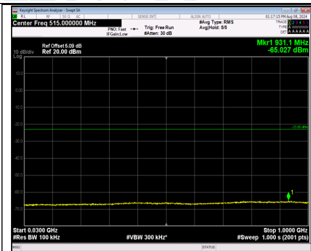
2-2-20MHz-20MHz-QPSK-QPSK-18801-18999-1RB#0-0 RB#0-30~1000MHz-PASS
