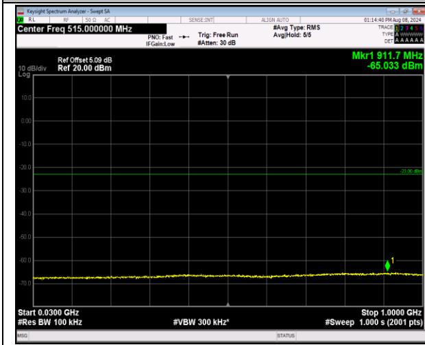
2-2-20MHz-20MHz-QPSK-QPSK-18700-18898-1RB#0-1 RB#99-30~1000MHz-PASS
