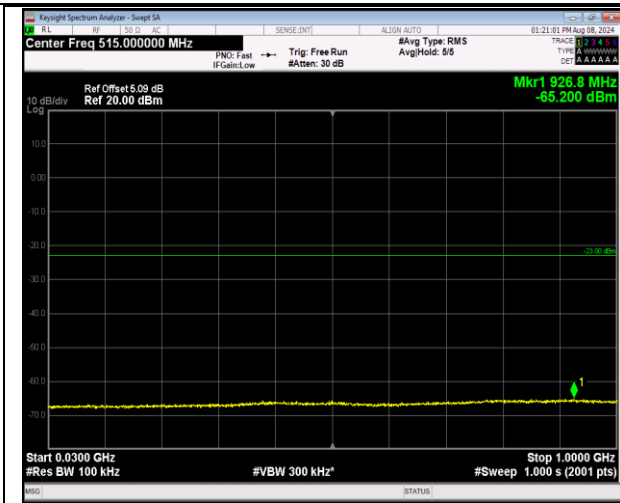
2-2-20MHz-20MHz-QPSK-QPSK-18801-18999-100RB# 0-100RB#0-30~1000MHz-PASS
