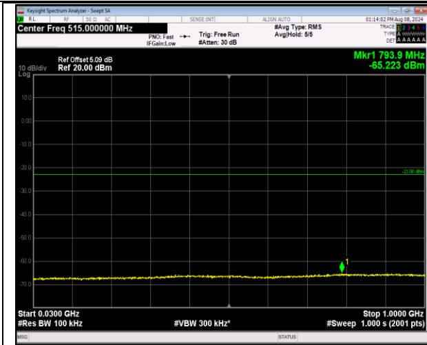
2-2-20MHz-20MHz-16QAM-16QAM-18700-18898-1RB# 99-0RB#0-30~1000MHz-PASS
