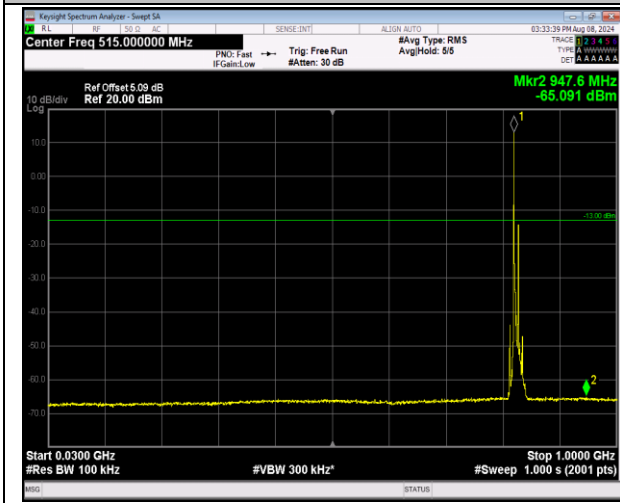
5-5-3MHz-5MHz-QPSK-QPSK-20416-20455-1RB#0-1R B#24-30~1000MHz-PASS
