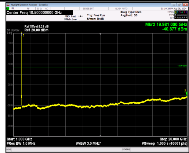
2-2-20MHz-20MHz-16QAM-16QAM-18801-18999-1RB#99-0RB#0-1000~20000MHz-PASS
