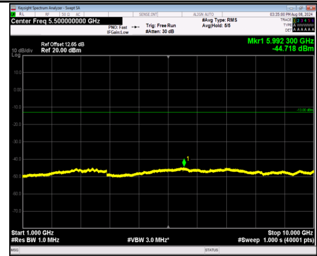
5-5-3MHz-5MHz-QPSK-QPSK-20416-20455-15RB#0-25 RB#0-1000~10000MHz-PASS
