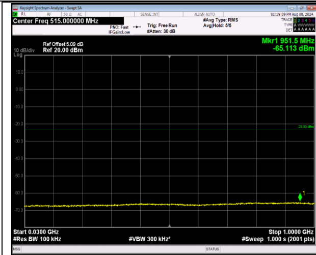
2-2-20MHz-20MHz-16QAM-16QAM-18801-18999-1RB#99-0RB#0-30~1000MHz-PASS
