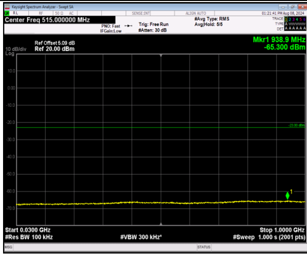
2-2-20MHz-20MHz-16QAM-16QAM-18801-18999-100RB#0-100RB#0-30~1000MHz-PASS
