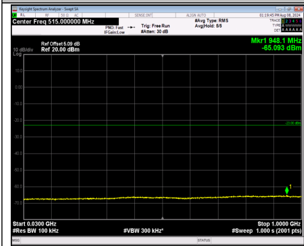
2-2-20MHz-20MHz-QPSK-QPSK-18801-18999-1RB#0-1 RB#99-30~1000MHz-PASS
