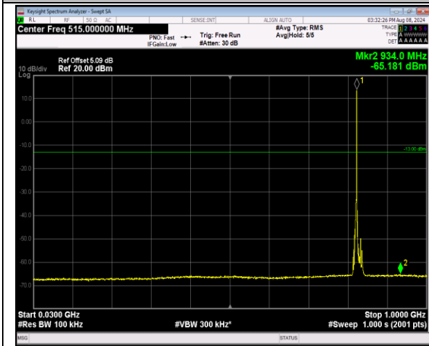
5-5-3MHz-5MHz-QPSK-QPSK-20416-20455-1RB#14-0R B#0-30~1000MHz-PASS
