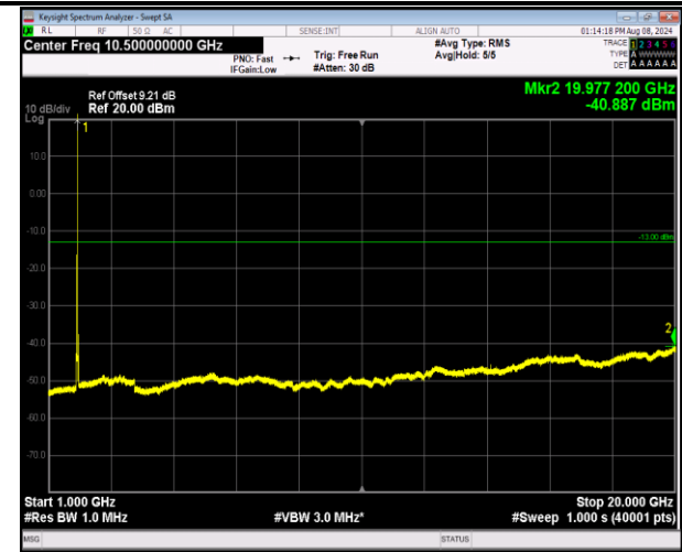
2-2-20MHz-20MHz-16QAM-16QAM-18700-18898-1RB#9 9-0RB#0-1000~20000MHz-PASS
