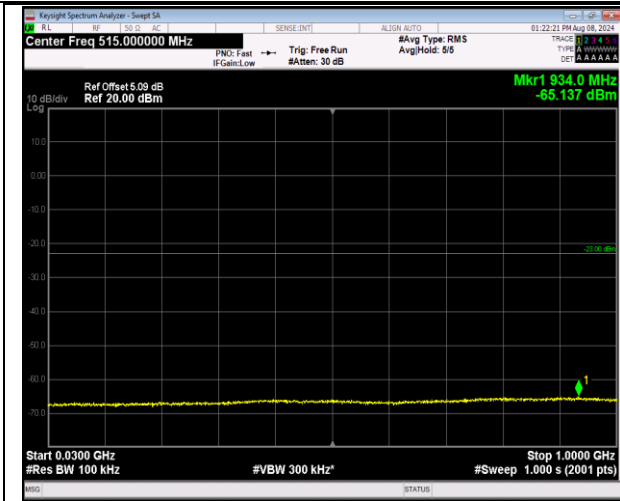
2-2-20MHz-20MHz-QPSK-QPSK-18902-19100-1RB#0-0 RB#0-30~1000MHz-PASS
