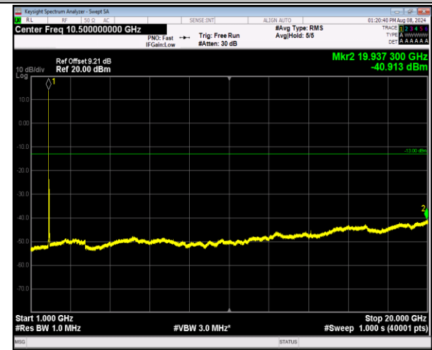
2-2-20MHz-20MHz-16QAM-16QAM-18801-18999-1RB#0 -1RB#99-1000~20000MHz-PASS
