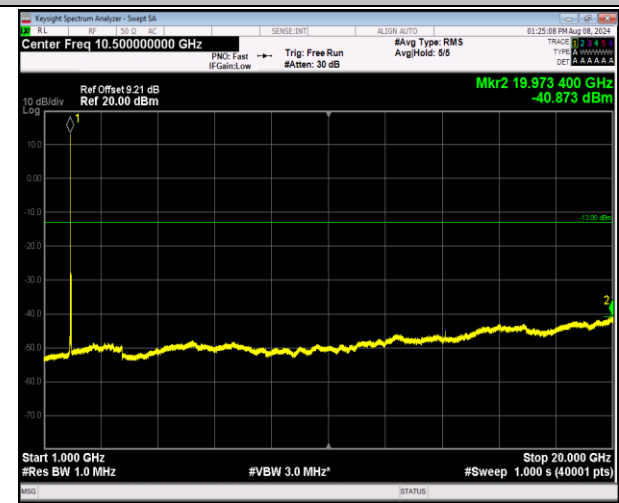
2-2-20MHz-20MHz-QPSK-QPSK-18902-19100-1RB#0-1 RB#99-1000~20000MHz-PASS
