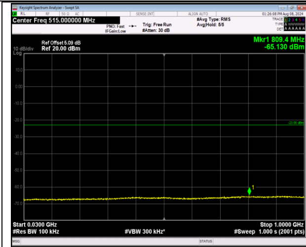
2-2-20MHz-20MHz-QPSK-QPSK-18902-19100-100RB# 0-100RB#0-30~1000MHz-PASS
