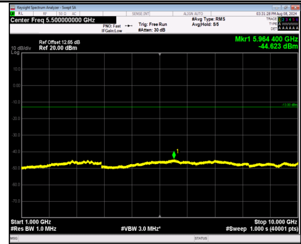
5-5-3MHz-5MHz-QPSK-QPSK-20416-20455-1RB#0-0RB #0-1000~10000MHz-PASS
