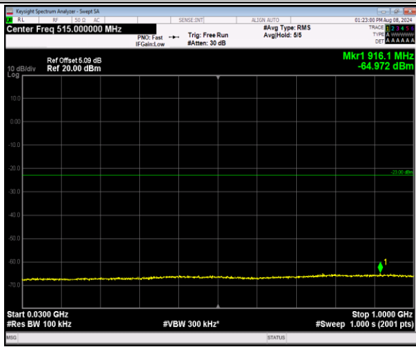
2-2-20MHz-20MHz-16QAM-16QAM-18902-19100-1RB# 0-0RB#0-30~1000MHz-PASS
