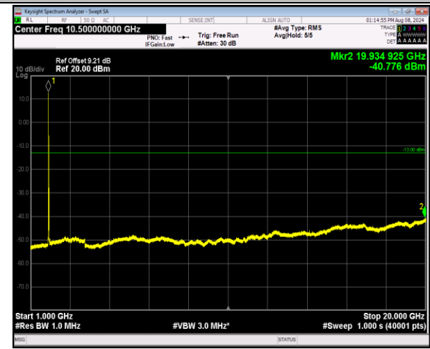
2-2-20MHz-20MHz-QPSK-QPSK-18700-18898-1RB#0-1 RB#99-1000~20000MHz-PASS
