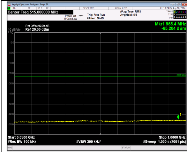
2-2-20MHz-20MHz-QPSK-QPSK-18700-18898-1RB#99-0 ORB#0-30~1000MHz-PASS
