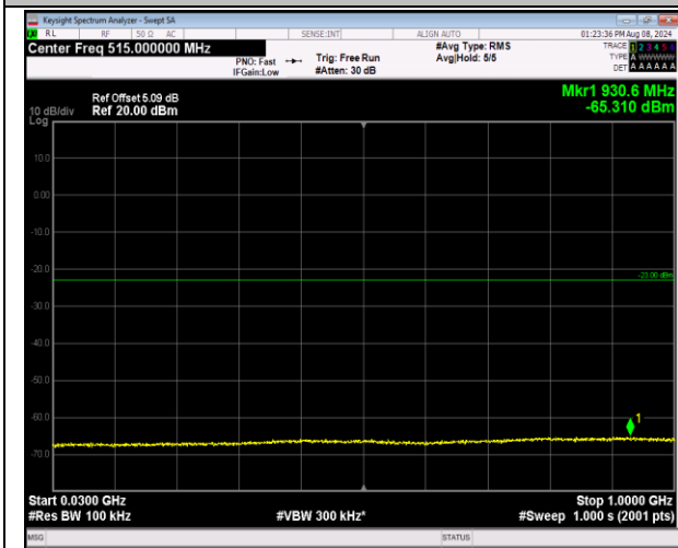
2-2-20MHz-20MHz-QPSK-QPSK-18902-19100-1RB#99-0 ORB#0-30~1000MHz-PASS
