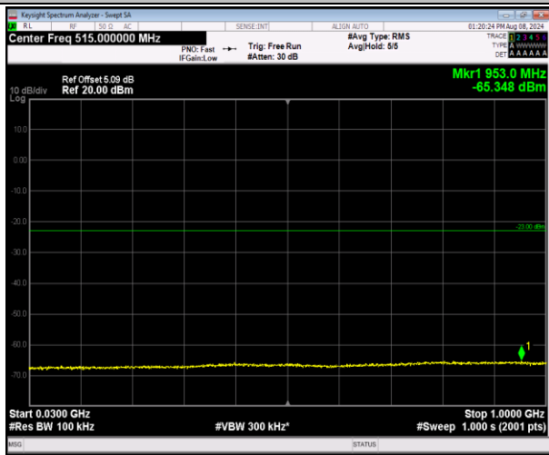
2-2-20MHz-20MHz-16QAM-16QAM-18801-18999-1RB# 0-1RB#99-30~1000MHz-PASS
