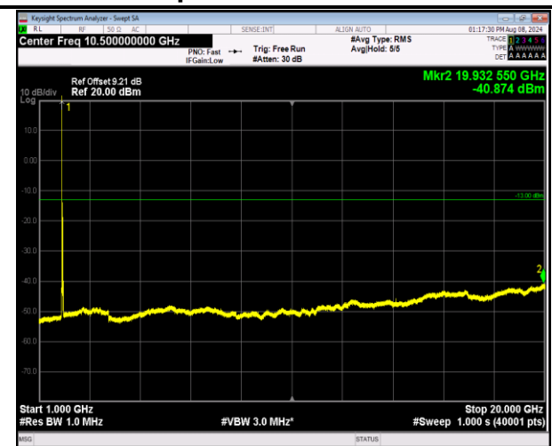
2-2-20MHz-20MHz-QPSK-QPSK-18801-18999-1RB#0-0 RB#0-1000~20000MHz-PASS
