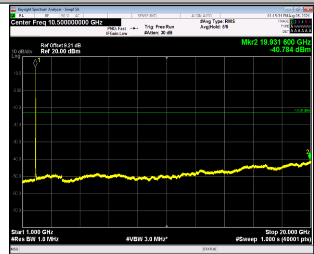
2-2-20MHz-20MHz-16QAM-16QAM-18700-18898-1RB#0 -1RB#99-1000~20000MHz-PASS
