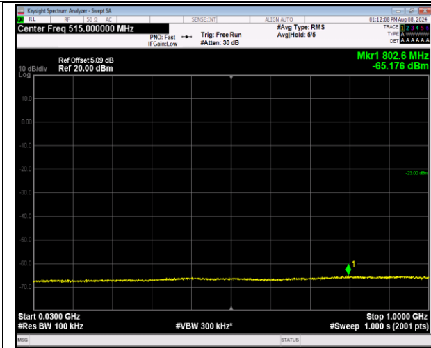
2-2-20MHz-20MHz-QPSK-QPSK-18700-18898-1RB#0-0 RB#0-30~1000MHz-PASS
