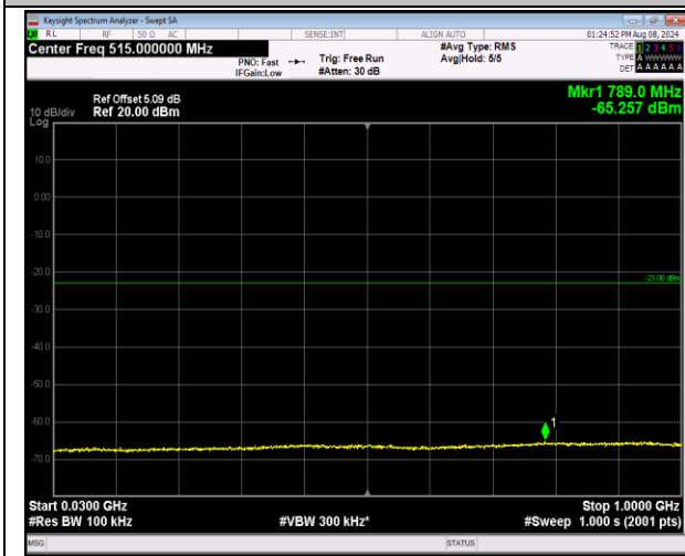
2-2-20MHz-20MHz-QPSK-QPSK-18902-19100-1RB#0-1 RB#99-30~1000MHz-PASS
