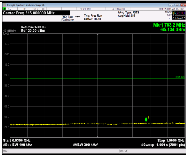
2-2-20MHz-20MHz-16QAM-16QAM-18801-18999-1RB# 0-0RB#0-30~1000MHz-PASS
