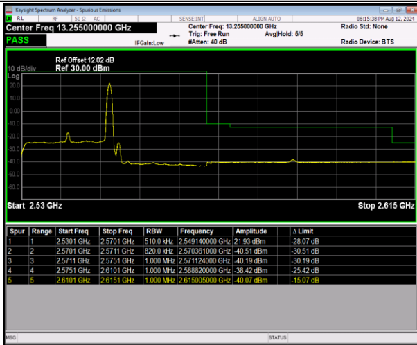
7-7-20MHz-20MHz-16QAM@16QAM-16QAM@16QAM-2
