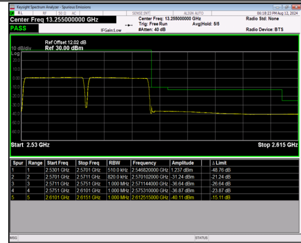
7-7-20MHz-20MHz-16QAM@16QAM-16QAM@16QAM-2
