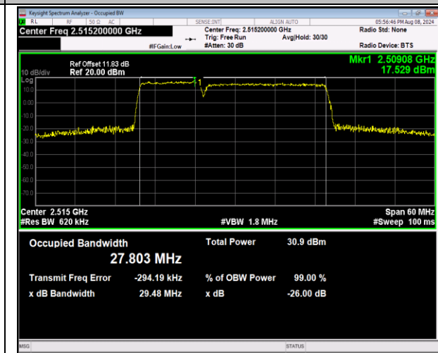
7-7-10MHz-20MHz-QPSK-QPSK-20805-20949-50RB#0- 100RB#0-PASS
