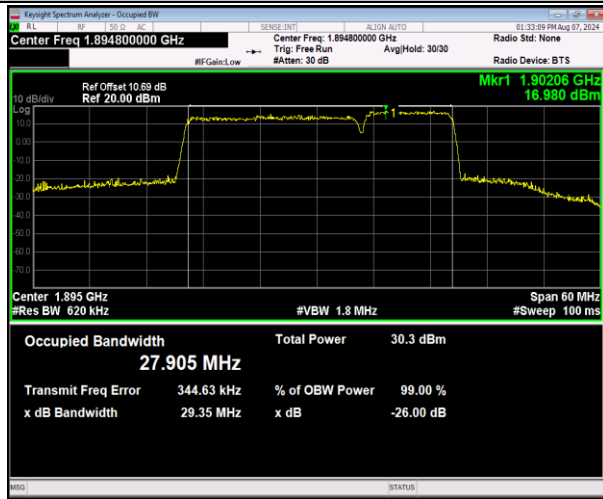
2-2-20MHz-10MHz-16QAM-16QAM-19001-19145-100RB#0-50RB#0-PASS
