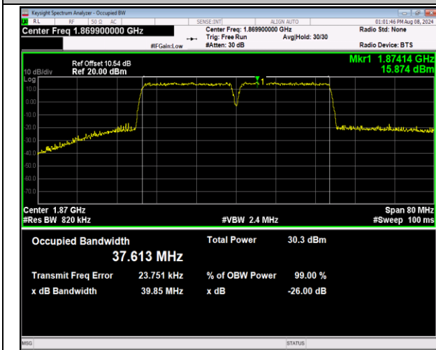
2-2-20MHz-20MHz-16QAM-16QAM-18700-18898-100RB#0-100RB#0-PASS
