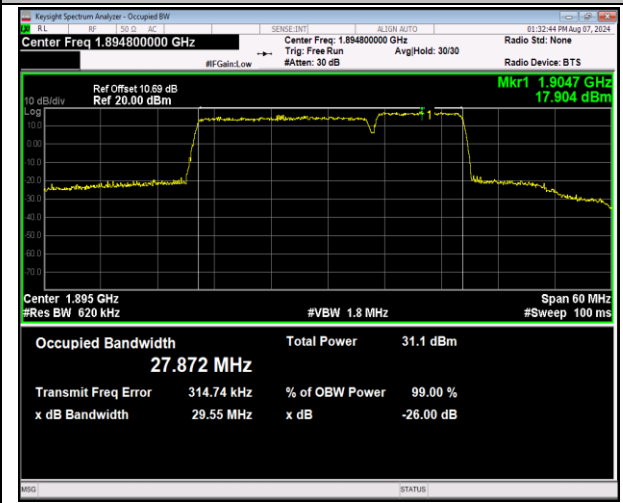
2-2-20MHz-10MHz-QPSK-QPSK-19001-19145-100RB#0-50RB#0-PASS
