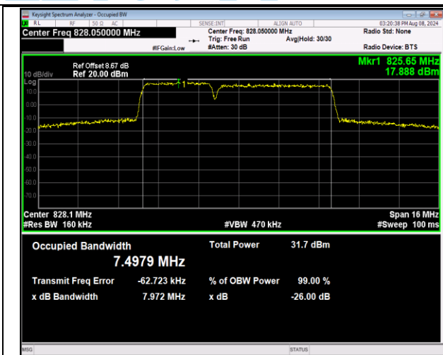
5-5-3MHz-5MHz-QPSK-QPSK-20416-20455-15RB#0-25 RB#0-PASS
