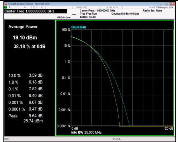
2-2-20MHz-20MHz-16QAM-16QAM-18801-18999-100RB#0 #0-100RB#0-PASS
