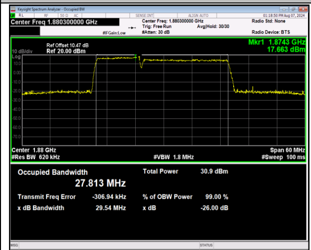
2-2-10MHz-20MHz-QPSK-QPSK-18806-18950-50RB#0- 100RB#0-PASS
