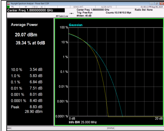
2-2-20MHz-20MHz-QPSK-QPSK-18801-18999-100RB#0 -100RB#0-PASS
