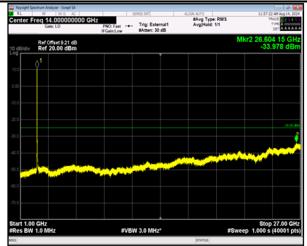
41-41-5MHz-20MHz-QPSK-QPSK-40273-40390-25RB#0-1 00RB#0-1000~27000MHz-PASS
