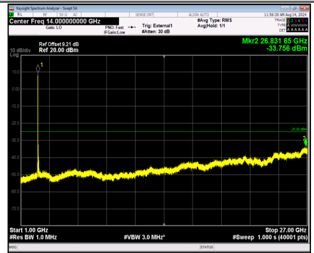
41-41-5MHz-20MHz-16QAM-16QAM-40273-40390-1RB#0- 1RB#99-1000~27000MHz-PASS
