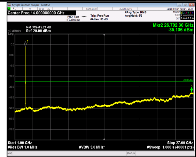
7-7-20MHz-20MHz-QPSK-QPSK-21152-21350-100RB#0-1 00RB#0-1000~27000MHz-PASS
