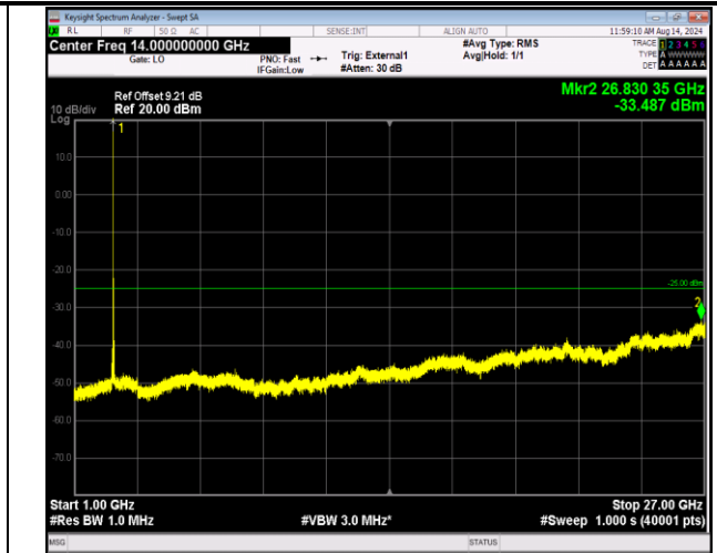
41-41-5MHz-20MHz-QPSK-QPSK-40648-40765-1RB#0-0RB#0-1000~27000MHz-PASS
