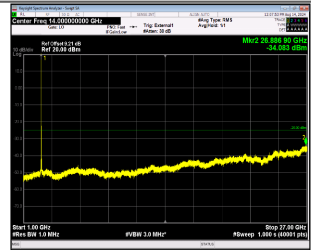
41-41-5MHz-20MHz-QPSK-QPSK-41023-41140-1RB#24-0RB#0-1000~27000MHz-PASS
