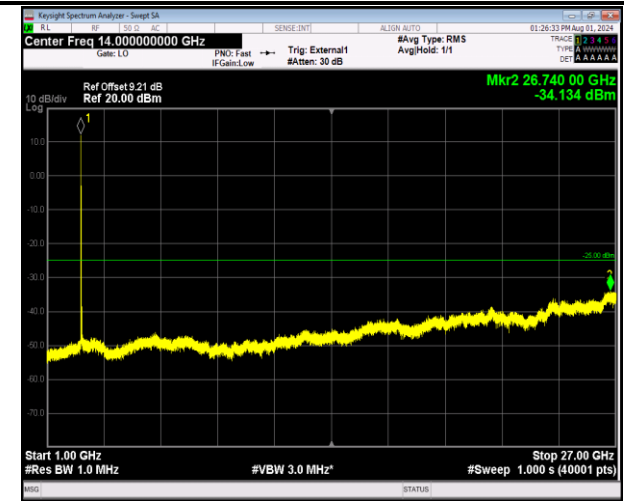
41-41-5MHz-20MHz-64QAM-64QAM-40273-40390-1RB#0- 1RB#99-1000~27000MHz-PASS
