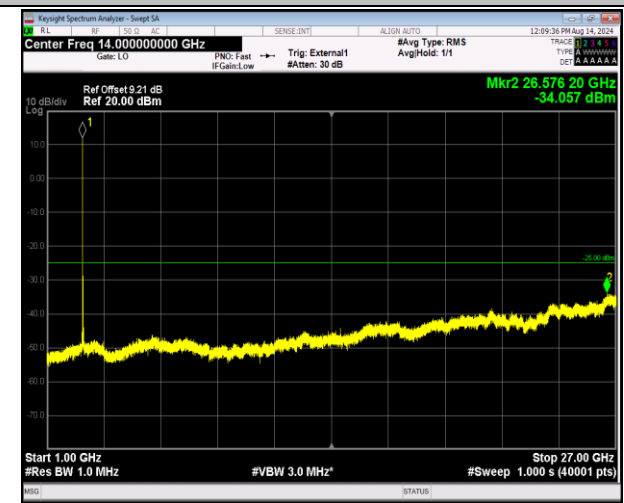
41-41-5MHz-20MHz-QPSK-QPSK-41023-41140-1RB#0-1RB#99-1000~27000MHz-PASS
