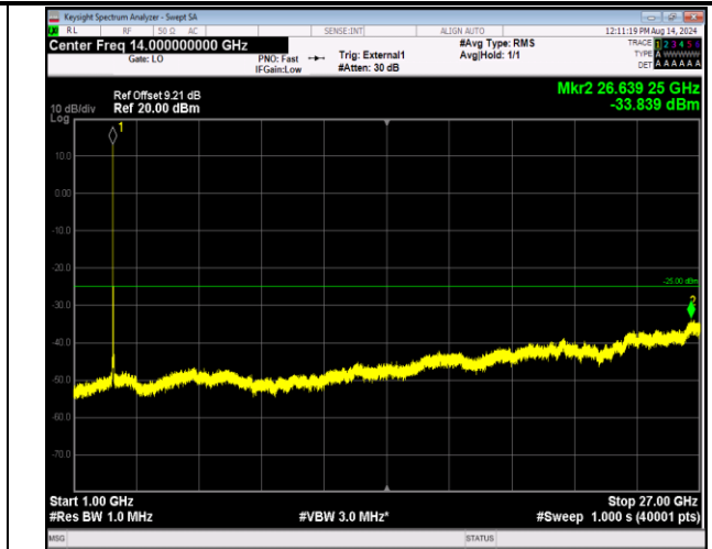
41-41-5MHz-20MHz-QPSK-QPSK-41023-41140-25RB#0-1 00RB#0-1000~27000MHz-PASS
