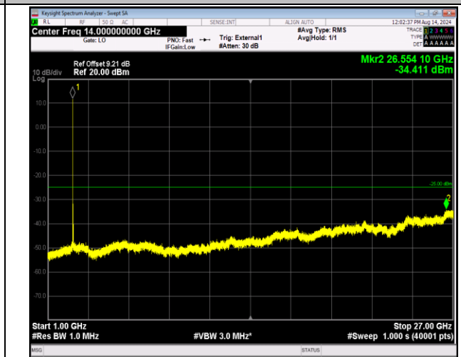
41-41-5MHz-20MHz-QPSK-QPSK-40648-40765-1RB#0-1RB#99-1000~27000MHz-PASS
