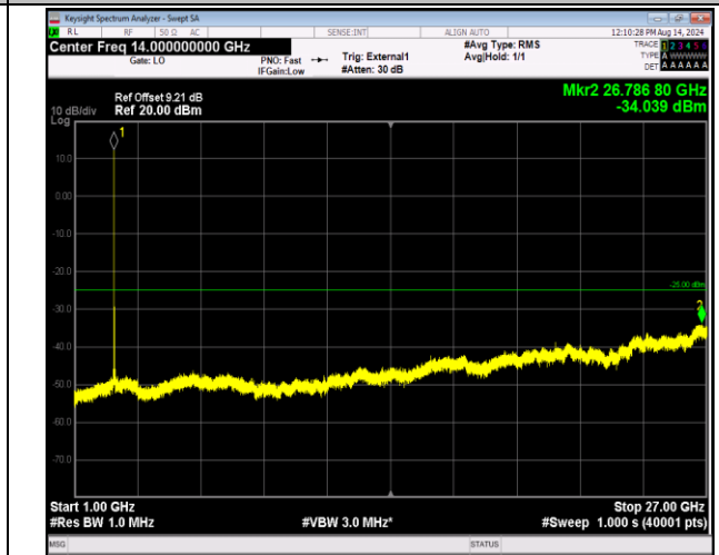
41-41-5MHz-20MHz-16QAM-16QAM-41023-41140-1RB#0- 1RB#99-1000~27000MHz-PASS
