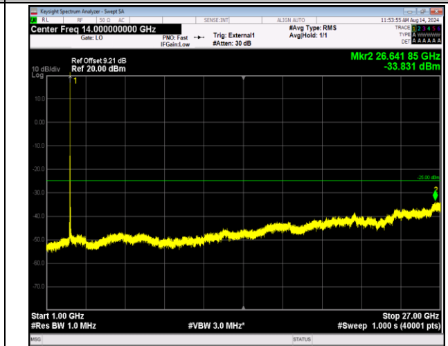
41-41-5MHz-20MHz-QPSK-QPSK-40273-40390-1RB#24-0RB#0-1000~27000MHz-PASS
