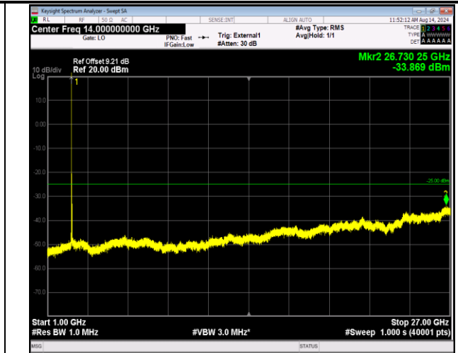
41-41-5MHz-20MHz-QPSK-QPSK-40273-40390-1RB#0-0RB#0-1000~27000MHz-PASS
