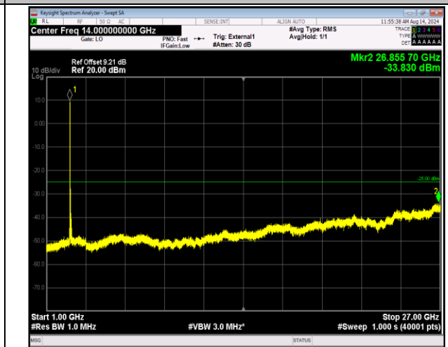
41-41-5MHz-20MHz-QPSK-QPSK-40273-40390-1RB#0-1RB#99-1000~27000MHz-PASS
