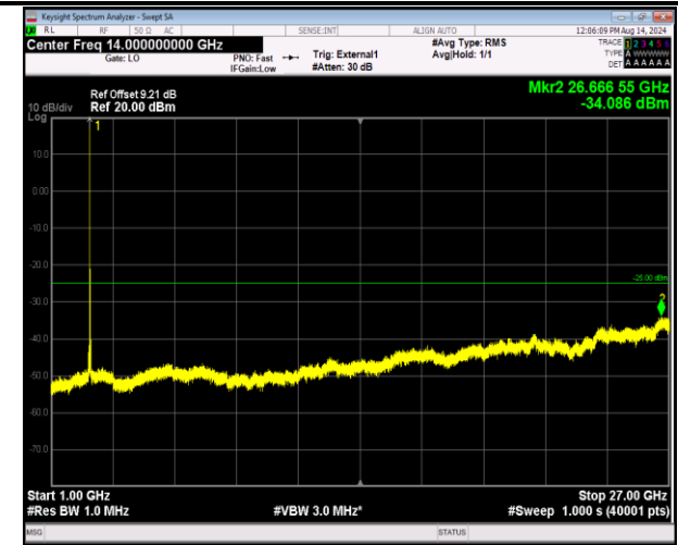
41-41-5MHz-20MHz-QPSK-QPSK-41023-41140-1RB#0-0RB#0-1000~27000MHz-PASS
