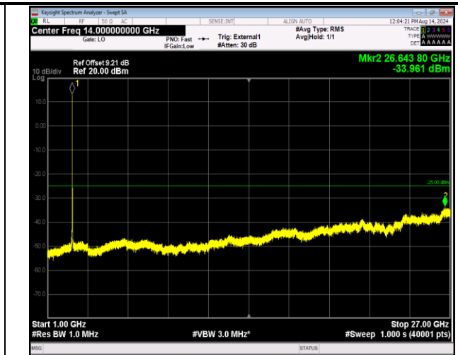
41-41-5MHz-20MHz-QPSK-QPSK-40648-40765-25RB#0-1 00RB#0-1000~27000MHz-PASS
