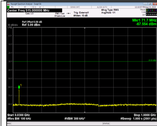
41-41-5MHz-20MHz-QPSK-QPSK-41023-41140-25RB#0 -100RB#0-30~1000MHz-PASS
